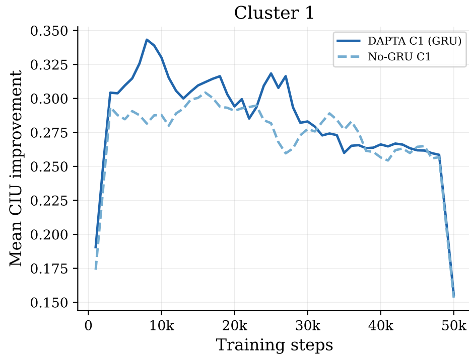
CIU improvement per cluster: GRU vs No-GRU DAPTA
