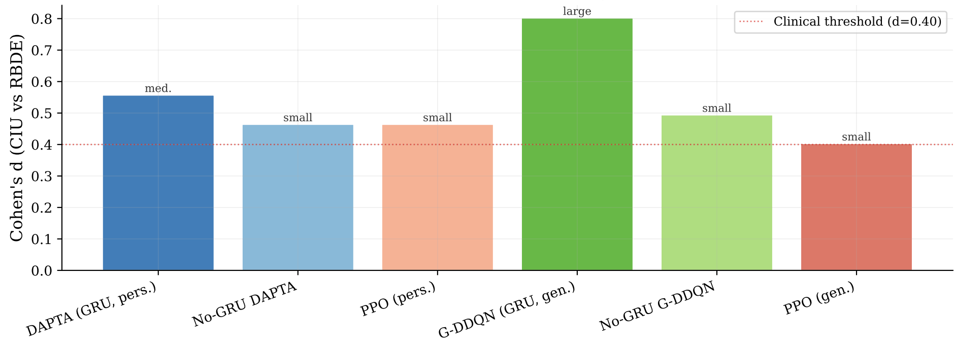
Ablation: GRU vs no-GRU, DDQN vs PPO
