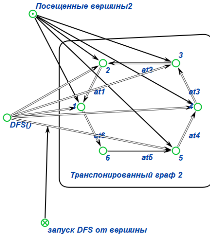
Рис. 21: Состояние SC-памяти на пятом шаге DFS транспонированного графа
