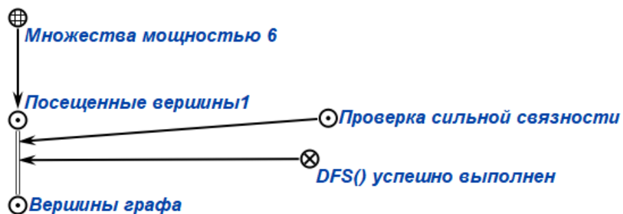
Рис. 15: Состояние SC-памяти после DFS 1 для Примера 2
