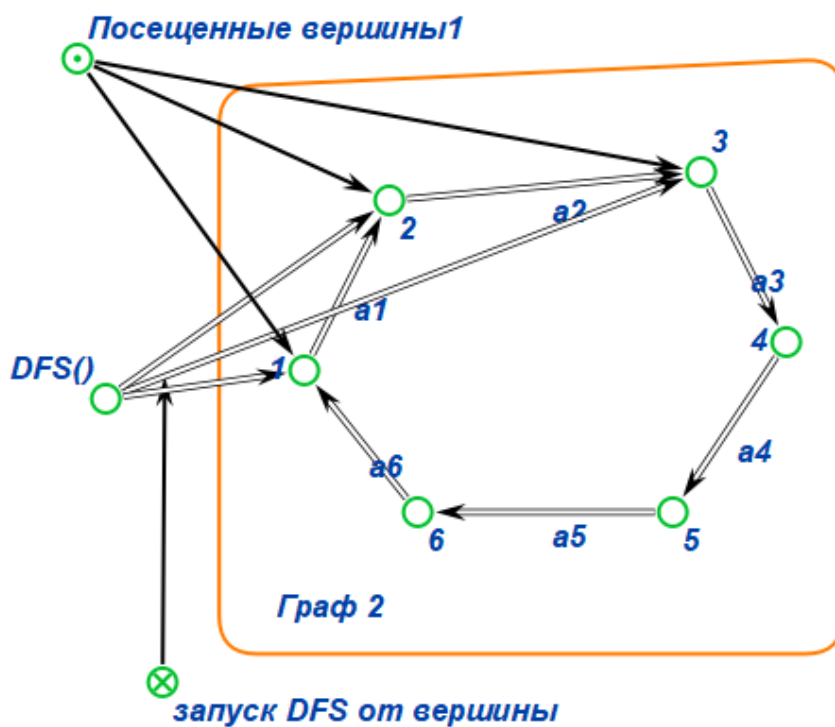
Рис. 11: Состояние SC-памяти на третьем шаге DFS
