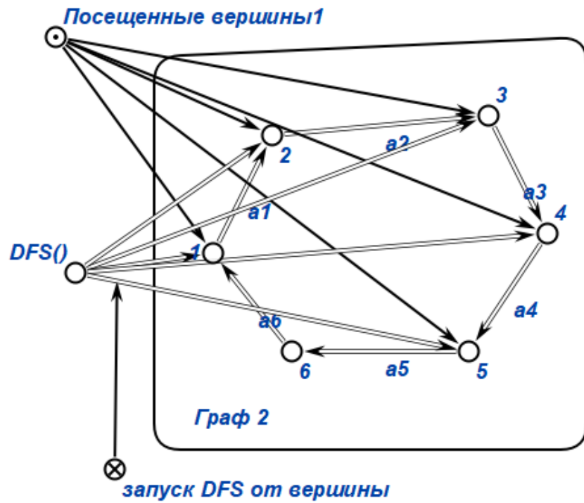
Рис. 13: Состояние SC-памяти на пятом шаге DFS
