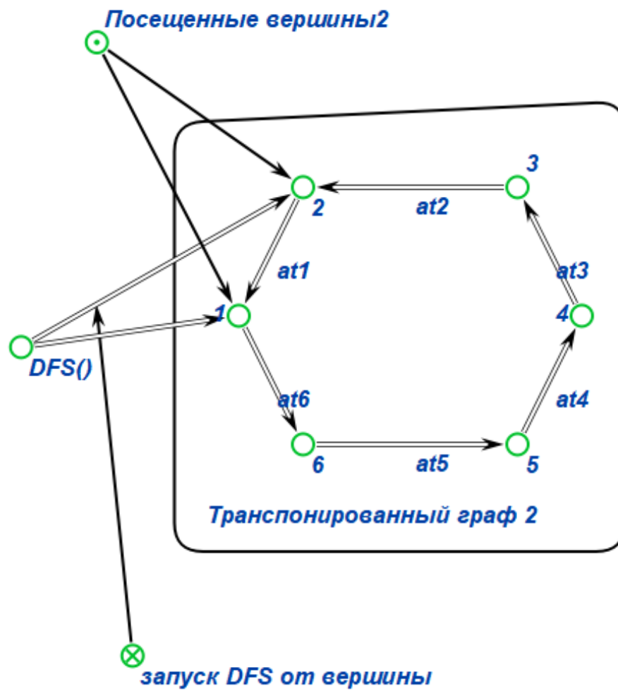
Рис. 18: Состояние SC-памяти на втором шаге DFS транспонированного графа
