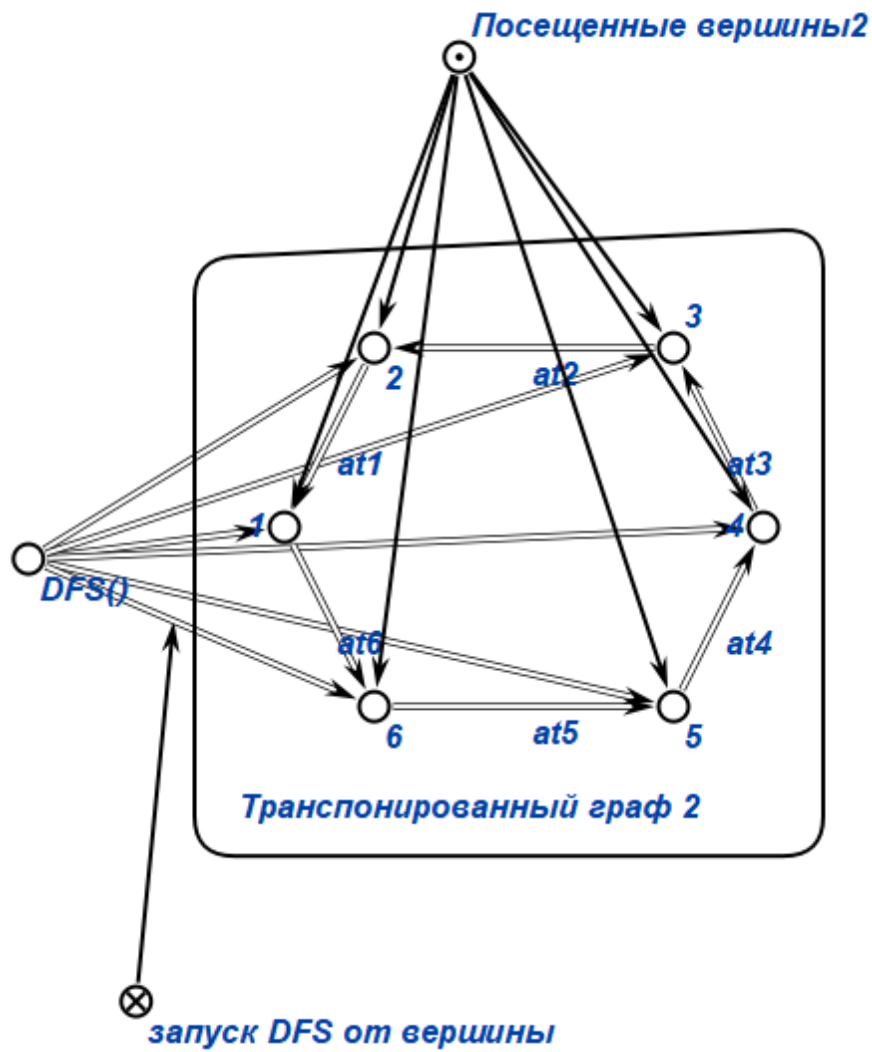
Рис. 22: Состояние SC-памяти на шестом шаге DFS транспонированного графа
