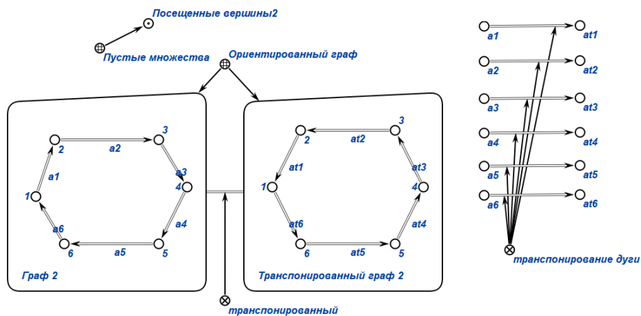
Рис. 16: SCg-представление транспонированного графа 2 для Примера 2
