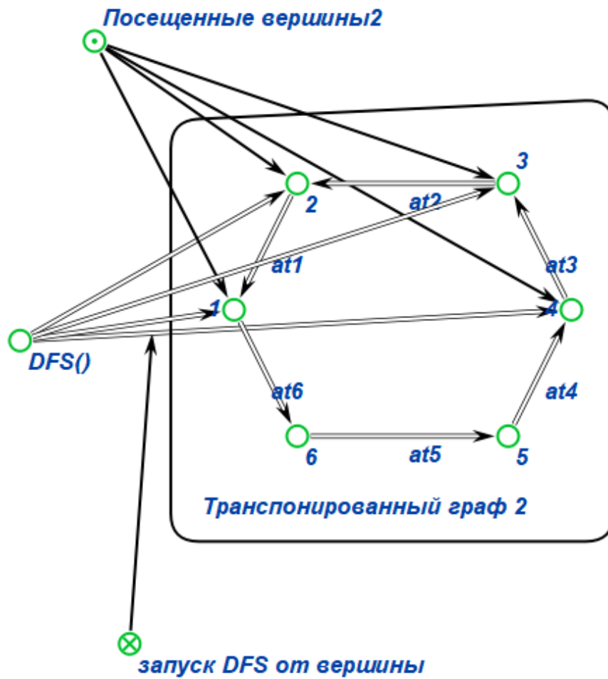
Рис. 20: Состояние SC-памяти на четвёртом шаге DFS транспонированного графа
