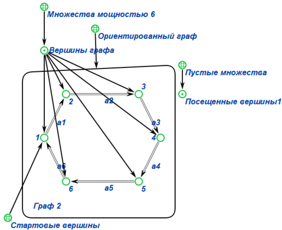
Рис. 8: SC-g представление условия Примера 2
