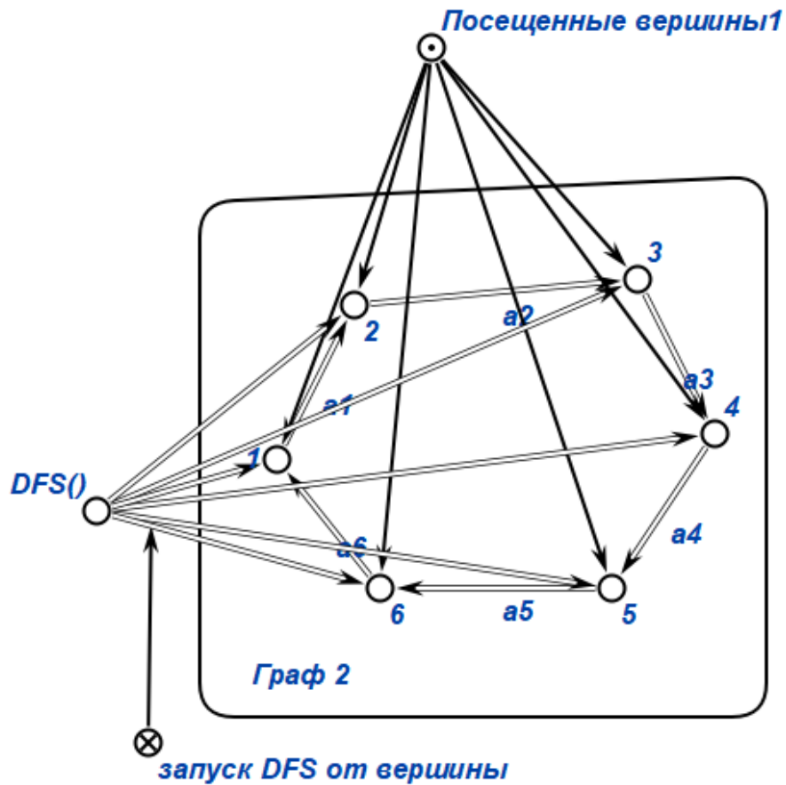
Рис. 14: Состояние SC-памяти на шестом шаге DFS
