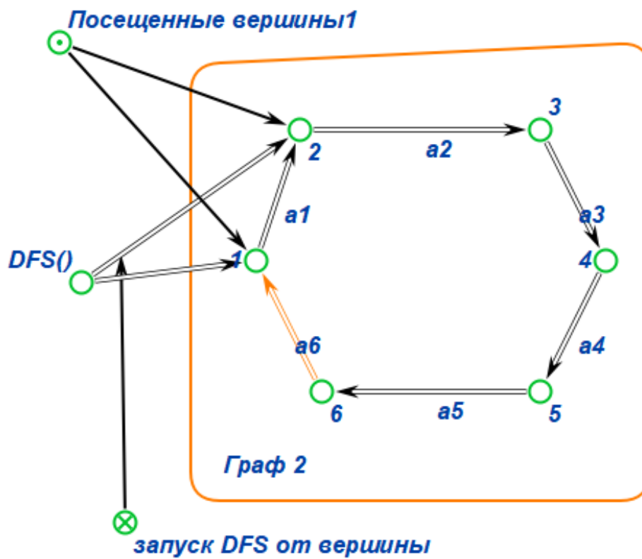
Рис. 10: Состояние SC-памяти на втором шаге DFS
