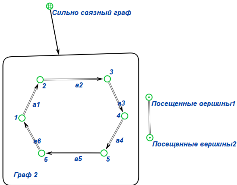
Рис. 24: Итоговое состояние SC-памяти для Примера 2
