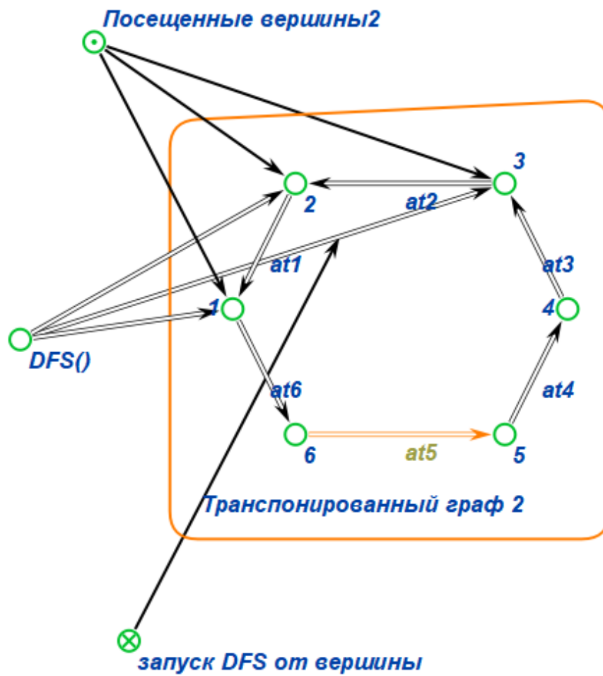
Рис. 19: Состояние SC-памяти на третьем шаге DFS транспонированного графа
