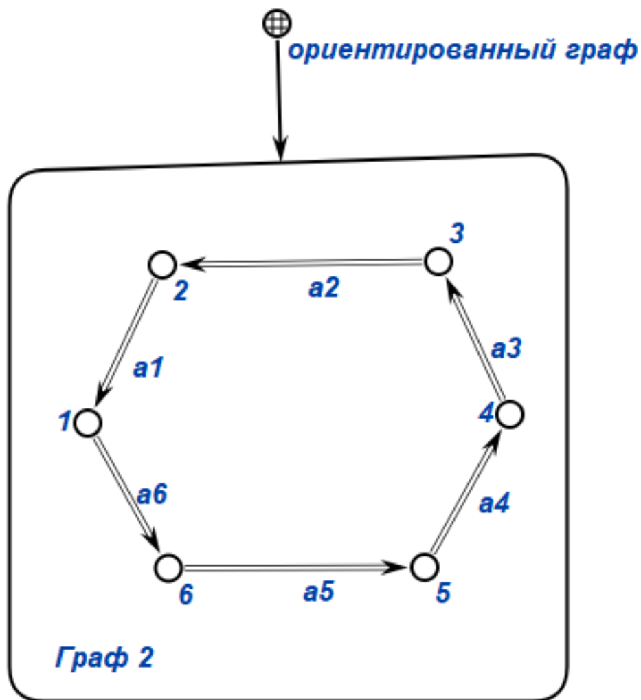
Рис. 9: SCg-представление транспонированного графа 2 для Примера 2
