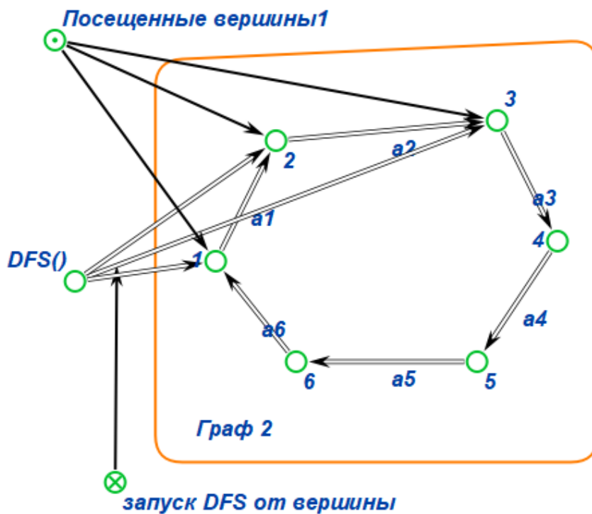
Рис. 11: Состояние SC-памяти на третьем шаге DFS
