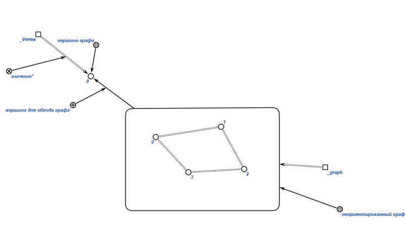
Рис. 4: Исходный граф
