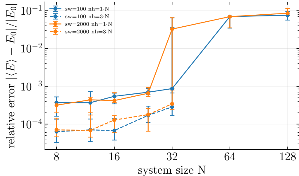
TFIM 1D — FPGA SA (median \pm IQR, 20 seeds)
