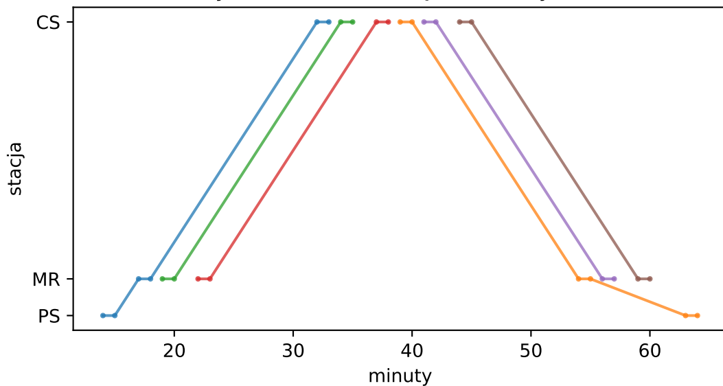
wykres ruchu rozwiązanie klasyczne
