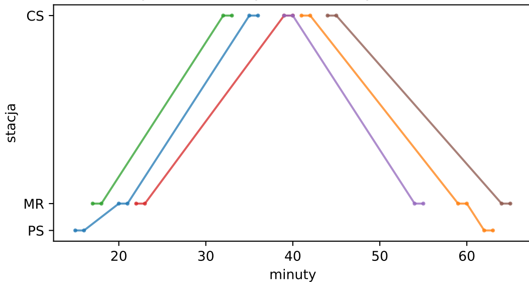
wykres ruchu symulowane wyżarzanie 2
