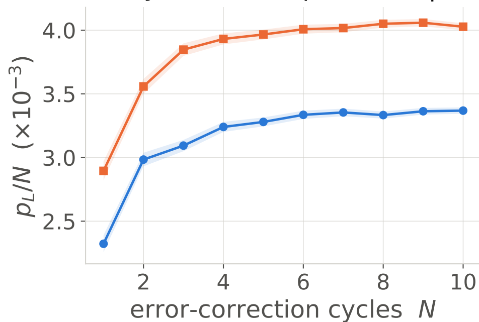
(d) cycle scan at p = 10^{-3} , |+\rangle_L
