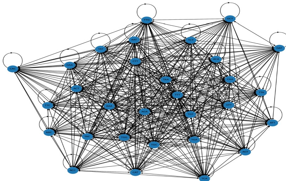
Figura 5: Rede de Transições entre os 30 Códon Mais Frequentes do SARS-CoV-2. Fonte. Os autores (2025).
