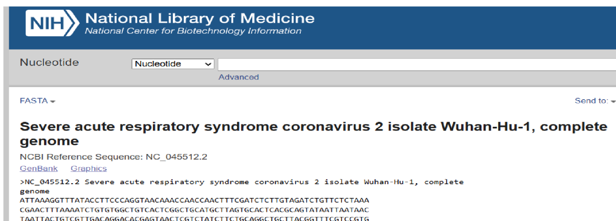
Figura 1 – Sequência FASTA do SARS-CoV-2 (NC_045512.2). Fonte: Adaptado de NCBI (2025)
