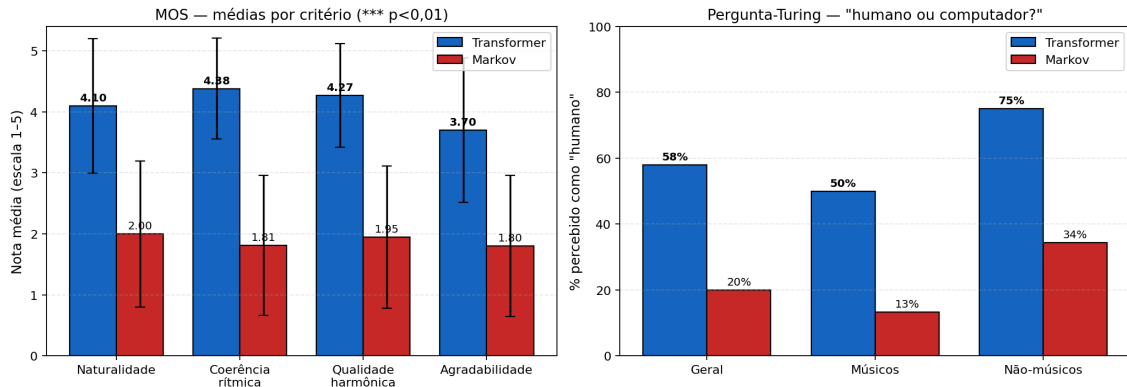
Figura 3. Resultados da avaliação subjetiva (MOS, N = 25 ). À esquerda, as médias por critério na escala Likert (1–5); à direita, o percentual de avaliadores que percebeu cada modelo como “composto por um humano”, segmentado por perfil musical. As barras de erro indicam o desvio-padrão.
