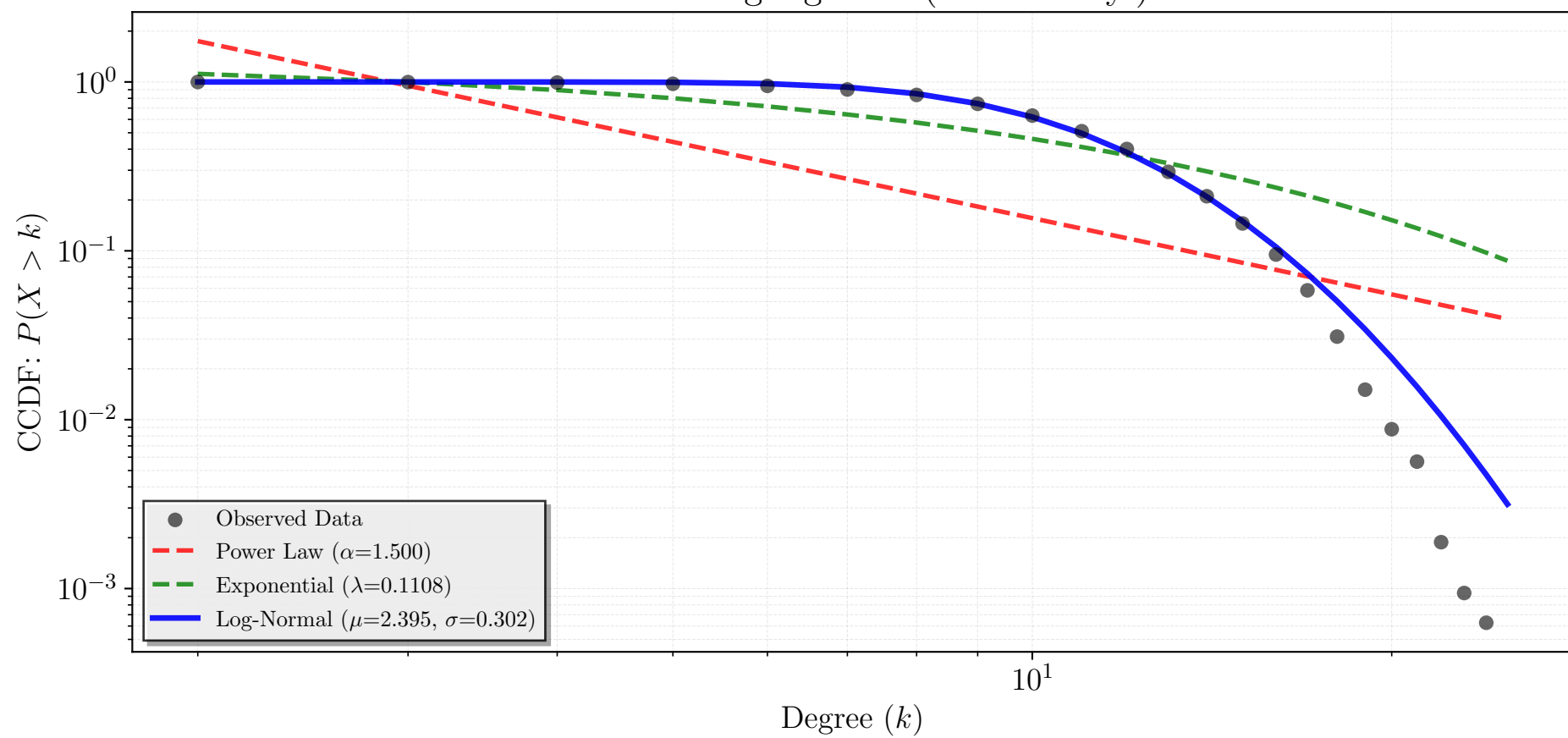
CCDF in log-log scale (Erdős-Rényi)
