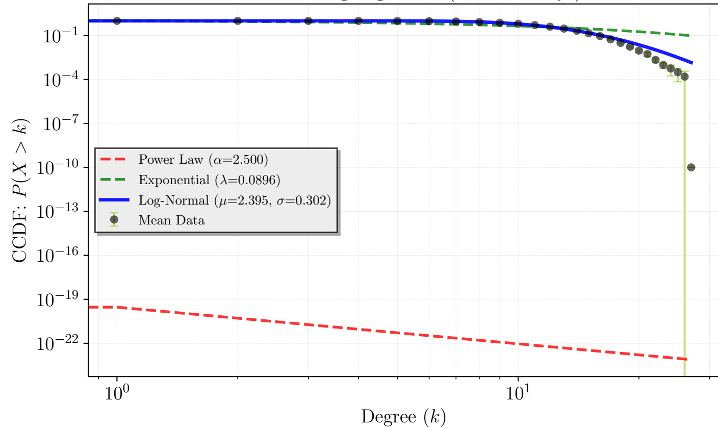
CCDF in log-log scale (Erdős-Rényi)
