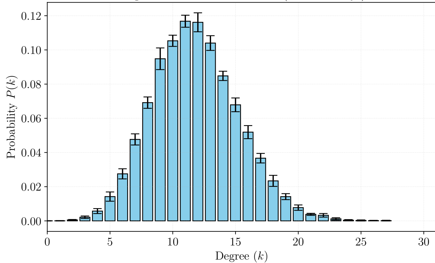
Degree Distribution - PDF (Erdős-Rényi)
