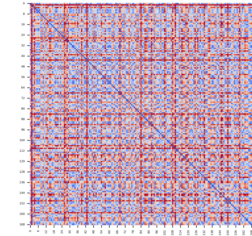
Perm 4 (seed=44)
