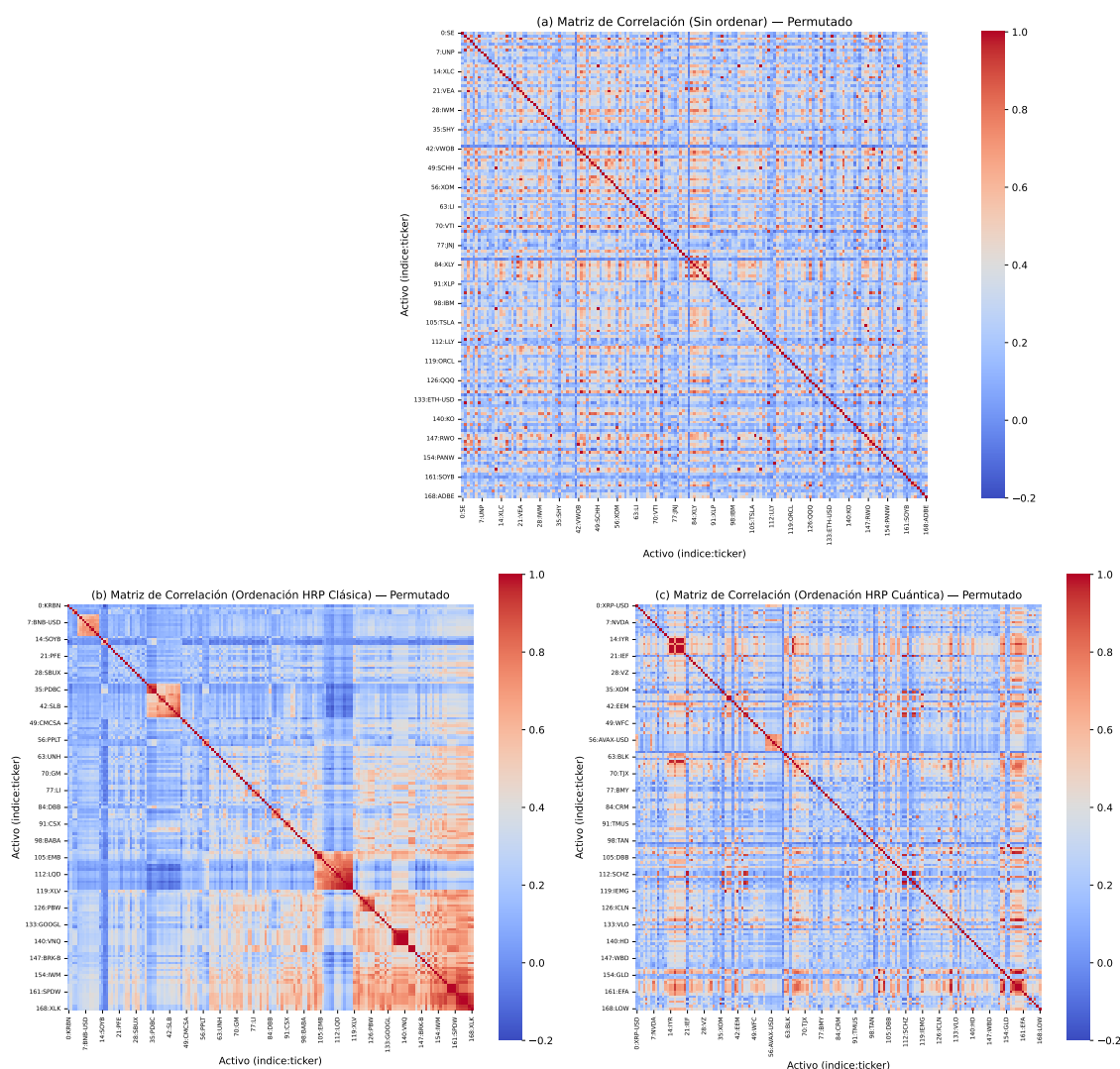
Figura 6.1: Visualización de matrices de correlación sin ordenar y tras HRP clásico en una permutación representativa de activos.
