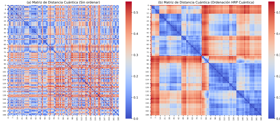
Figura 6.4: Figura de distancias cuánticas obtenida en este TFG con el mismo esquema metodológico que el utilizado en el paper de referencia [1].
