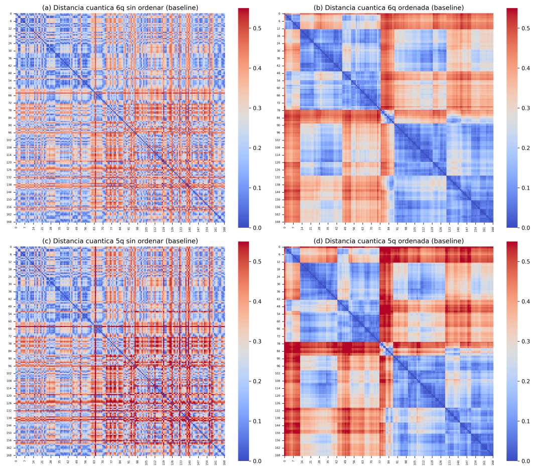
Figura 6.8: Matrices de distancia cuántica antes y después del ordenamiento QHRP para los escenarios de 6 y 5 qubits.
