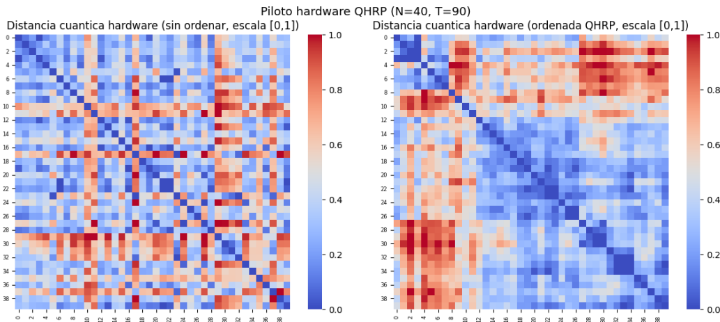
Figura 6.6: Equivalente a la Figura 4 del experimento principal, para el prototipo en hardware IBM ibm_fez. Los dos paneles muestran la matriz de distancia cuántica de Hellinger sin ordenar y tras el ordenamiento QHRP. El panel derecho evidencia la aparición de bloques de baja distancia cerca de la diagonal, indicando que la estructura jerárquica se transfiere al hardware real, si bien con mayor dispersión que en simulación ideal.
