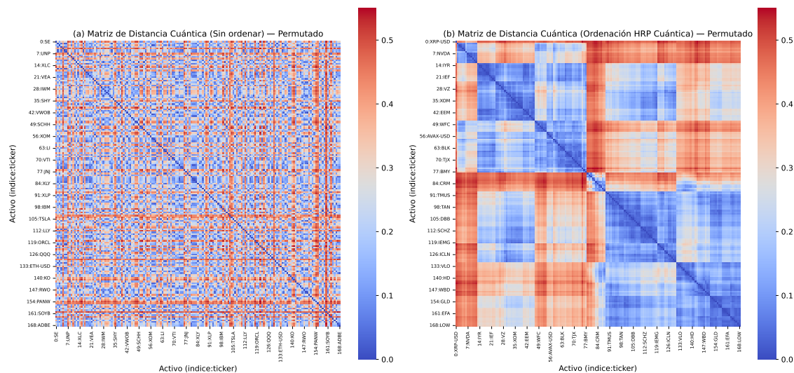
Figura 6.2: Visualización de matrices de distancia cuántica sin ordenar y tras QHRP en una permutación representativa de activos.
