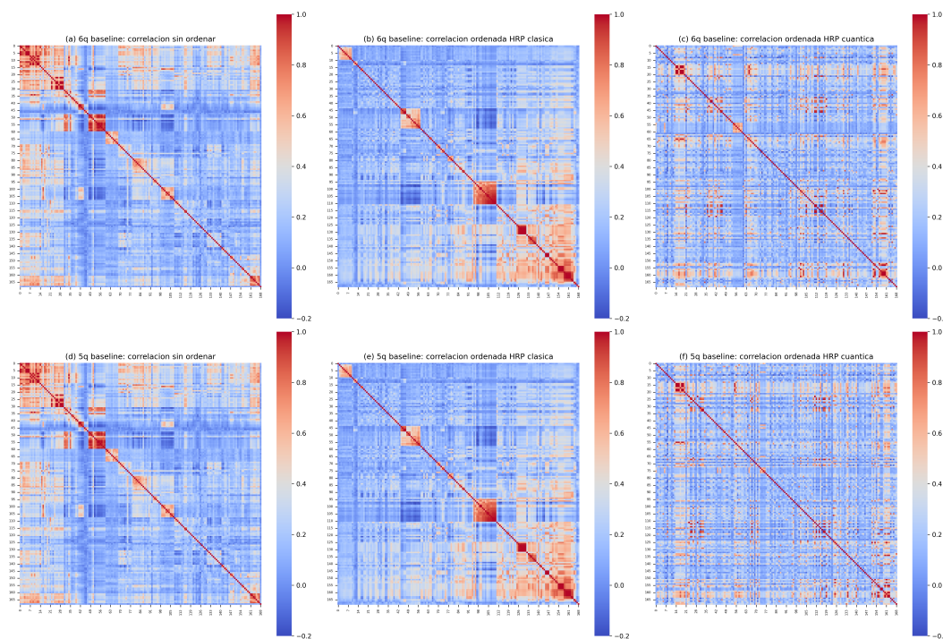
Figura 6.7: Matrices de correlación sin ordenar, ordenada por HRP clásico y ordenada por QHRP, para 6 qubits fila superior y 5 qubits fila inferior. La estructura de bloques cuasi-diagonales es equivalente en ambas configuraciones.
