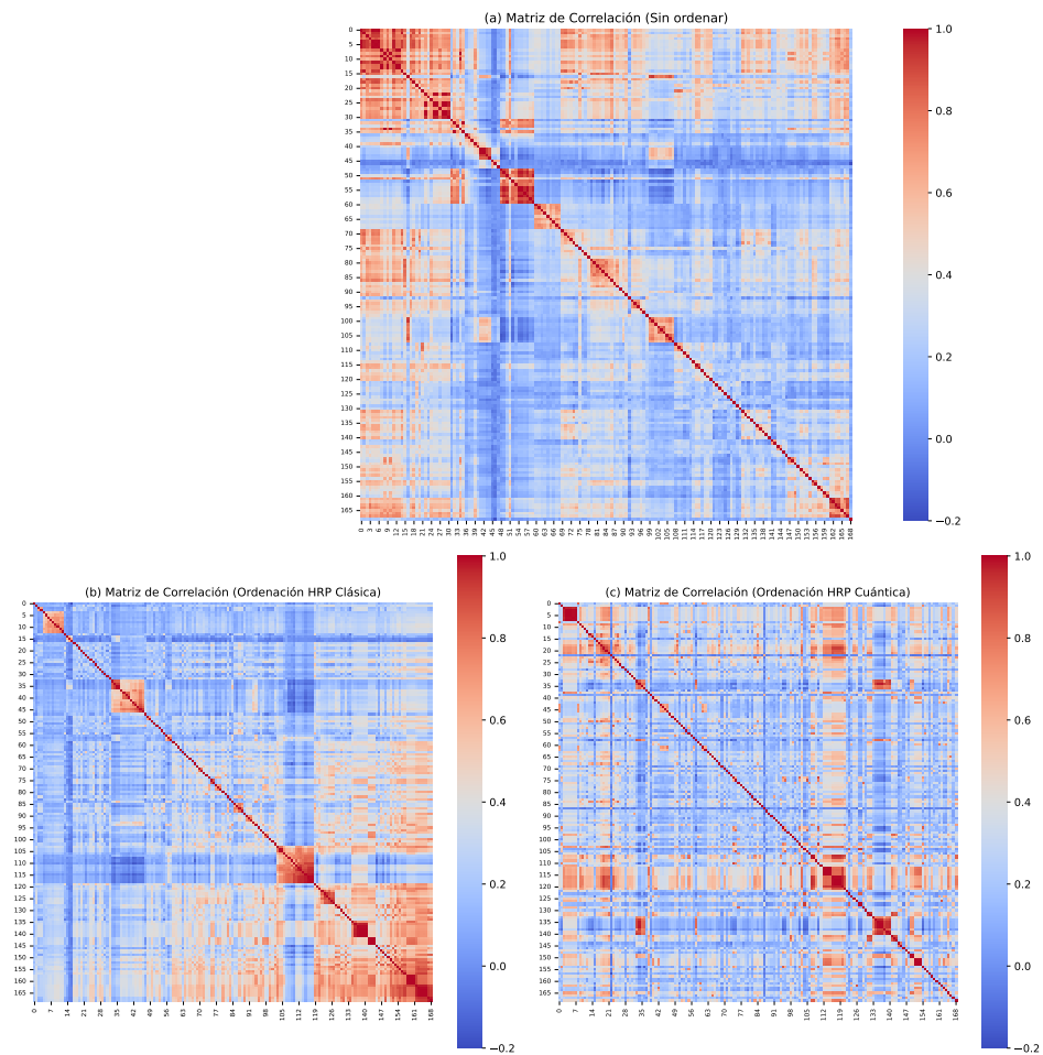
Figura 6.3: Figura de correlaciones reordenadas obtenida en este TFG con el mismo esquema metodológico que el utilizado en el paper de referencia [1].
