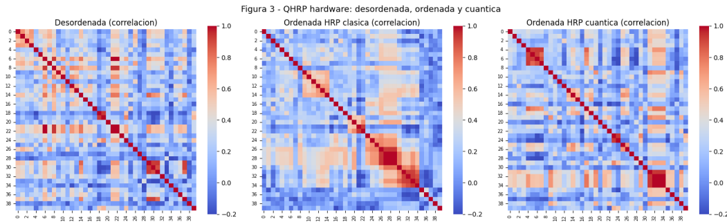
Figura 6.5: Equivalente a la Figura 3 del experimento principal, obtenido en el prototipo con hardware IBM ibm_fez ( N = 40 valores, T = 90 instantes temporales, P = 6 características, 256 ejecuciones/circuito). Los tres paneles muestran la matriz de correlación sin ordenar, ordenada por HRP clásico y ordenada por QHRP cuyo ordenamiento se derivó del hardware real.
