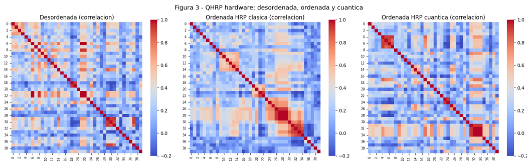
Figura 6.5: Equivalente a la Figura 3 del experimento principal, obtenido en el prototipo con hardware IBM ibm_fez ( N = 40 , T = 90 , 256 ejecuciones/circuito). Los tres paneles muestran la matriz de correlación sin ordenar, ordenada por HRP clásico y ordenada por QHRP cuyo ordenamiento se derivó del hardware real.
