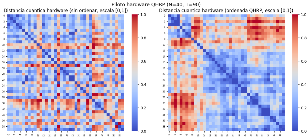
Figura 6.6: Equivalente a la Figura 4 del experimento principal, para el prototipo en hardware IBM ibm_fez . Los dos paneles muestran la matriz de distancia cuántica (Hellinger) sin ordenar y tras el ordenamiento QHRP. El panel derecho evidencia la aparición de bloques de baja distancia cerca de la diagonal, indicando que la estructura jerárquica se transfiere al hardware real, si bien con mayor dispersión que en simulación ideal.
