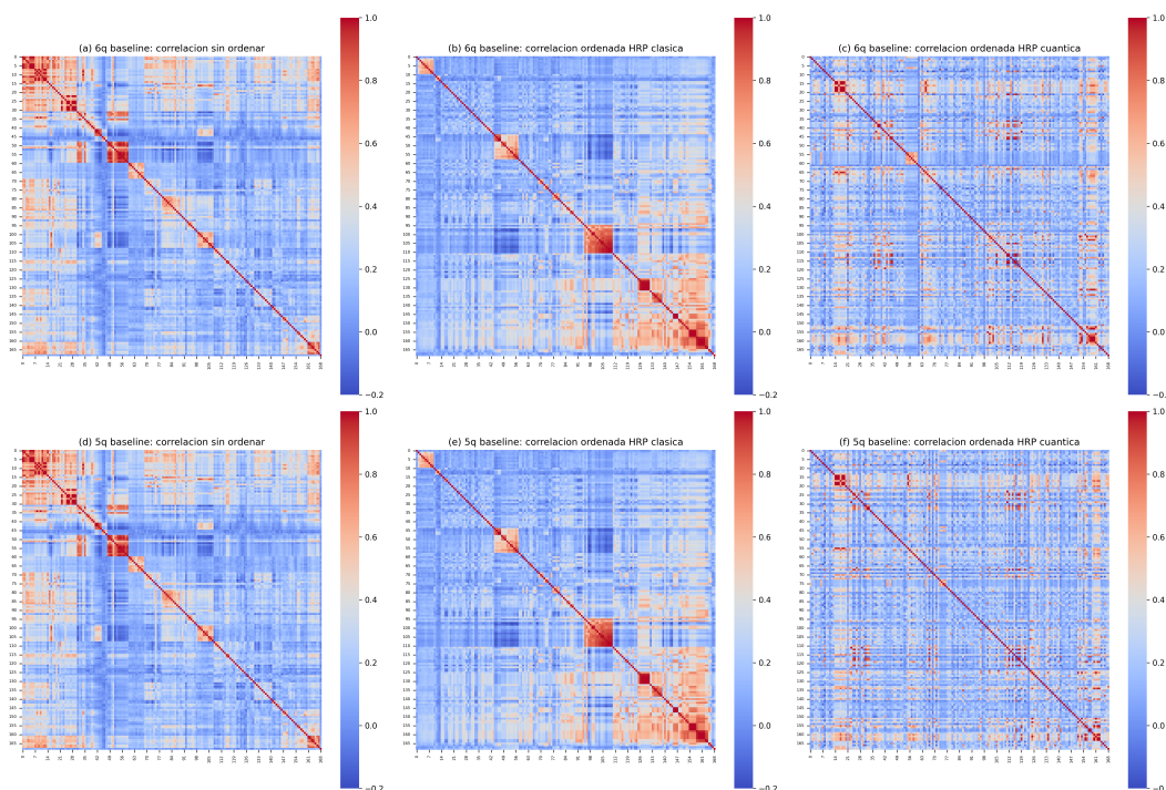
Figura 6.7: Matrices de correlación sin ordenar, ordenada por HRP clásico y ordenada por QHRP, para 6 qubits (fila superior) y 5 qubits (fila inferior). La estructura de bloques cuasi-diagonales es equivalente en ambas configuraciones.
