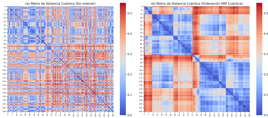
Figura 6.4: Figura de distancias cuánticas obtenida en este TFG con el mismo esquema metodológico que el utilizado en el paper de referencia [1].
