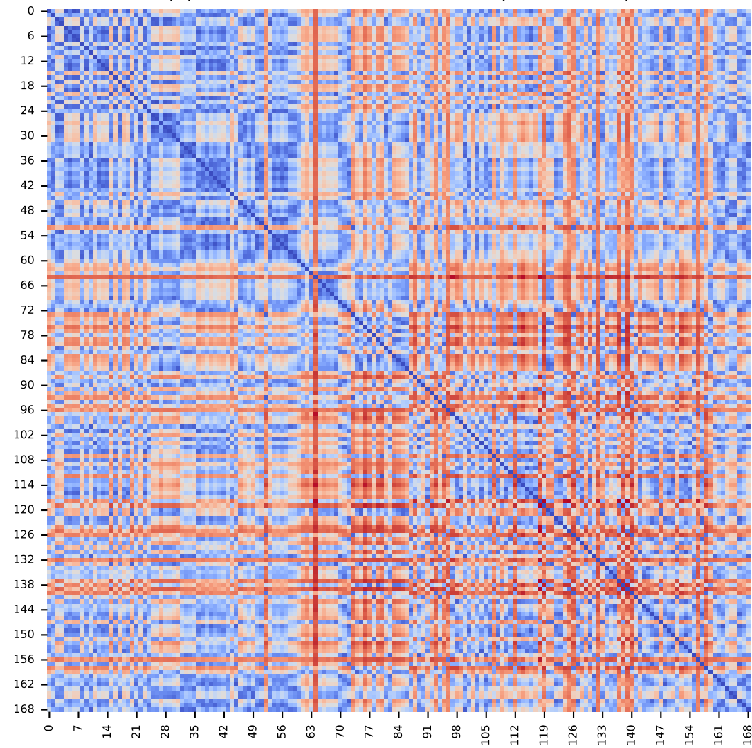
(a) Matriz de Distancia Cuántica (Sin ordenar)
