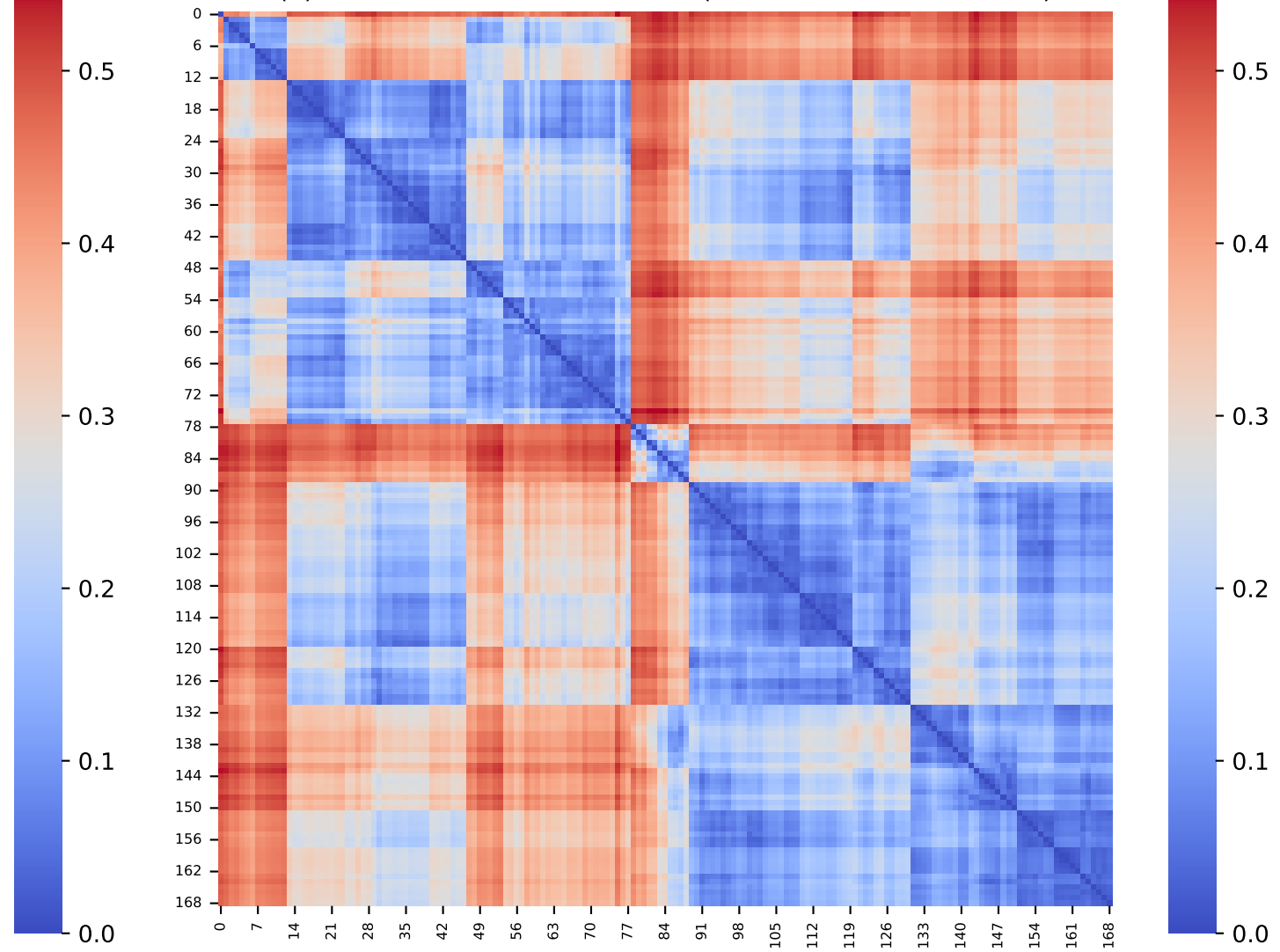
(b) Matriz de Distancia Cuántica (Ordenación HRP Cuántica)
