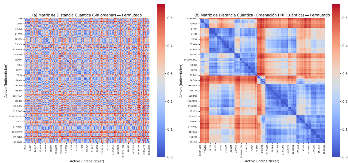
Figura 6.2: Visualización de matrices de distancia cuántica sin ordenar y tras QHRP en una permutación representativa de activos. a) Matriz de distancia cuántica sin ordenar, b) Matriz de distancia cuántica ordenada por HRP Cuántico
