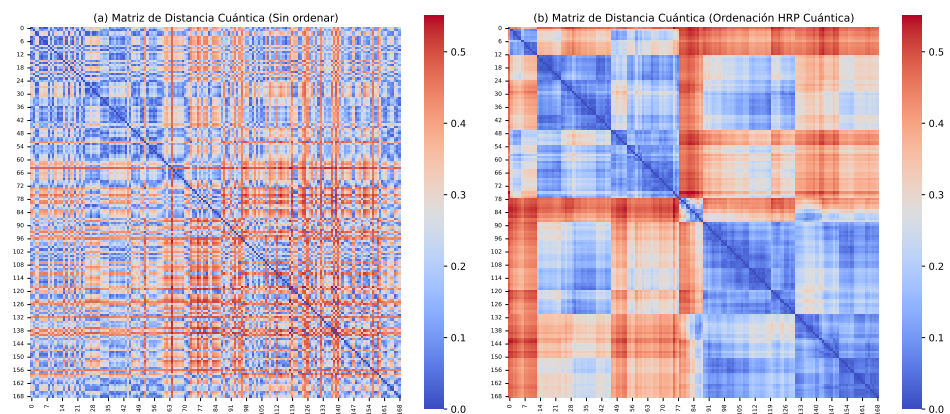
Figura 6.4: Figura de distancias cuánticas obtenida en este TFG con el mismo esquema metodológico que el utilizado en el artículo de referencia [1]. a) Matriz de distancia cuántica sin ordenar, b) Matriz de distancia cuántica ordenada por HRP Cuántico.
