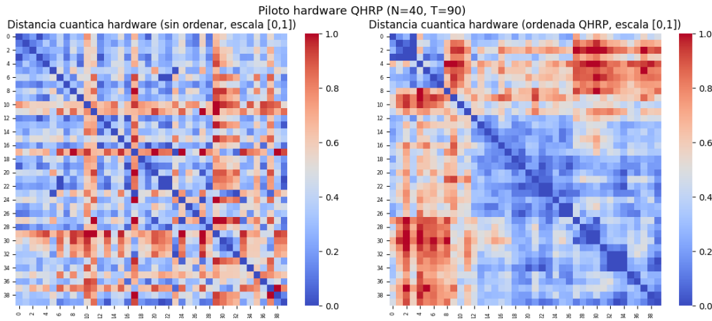
Figura 6.6: Equivalente a la Figura 4 del artículo de referencia [1], que se realizó en simulación, para el prototipo en hardware IBM ibm_fez. a) Matriz de distancia cuántica sin ordenar, b) Matriz de distancia cuántica ordenada por QHRP. El panel derecho evidencia la aparición de bloques de baja distancia cerca de la diagonal, indicando que la estructura jerárquica se transfiere al hardware real, si bien con mayor dispersión que en simulación ideal.
