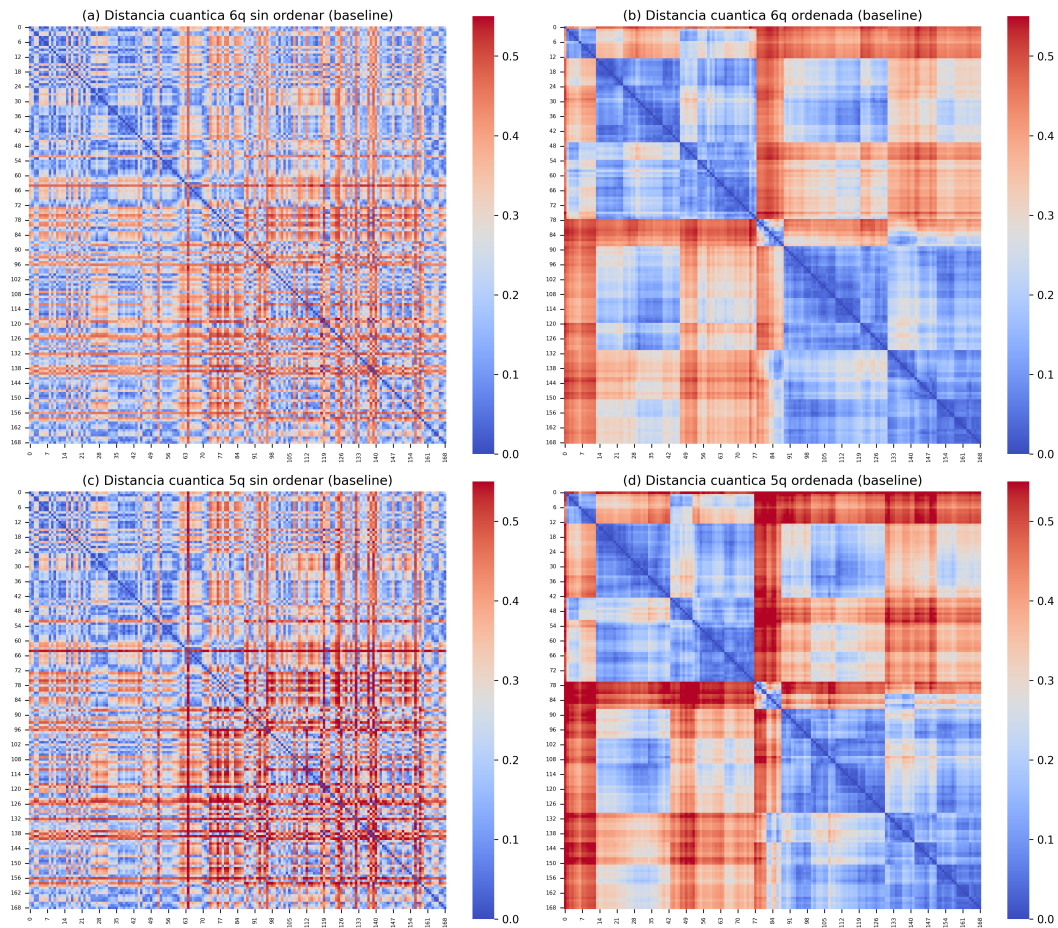
Figura 6.8: Matrices de distancia cuántica antes y después del ordenamiento QHRP para los escenarios de 6 y 5 qubits. a) Matriz de distancia cuántica sin ordenar con 6 qubits, b) Matriz de distancia cuántica ordenada por QHRP con 6 qubits, c) Matriz de distancia cuántica sin ordenar con 5 qubits, d) Matriz de distancia cuántica ordenada por QHRP con 5 qubits.
