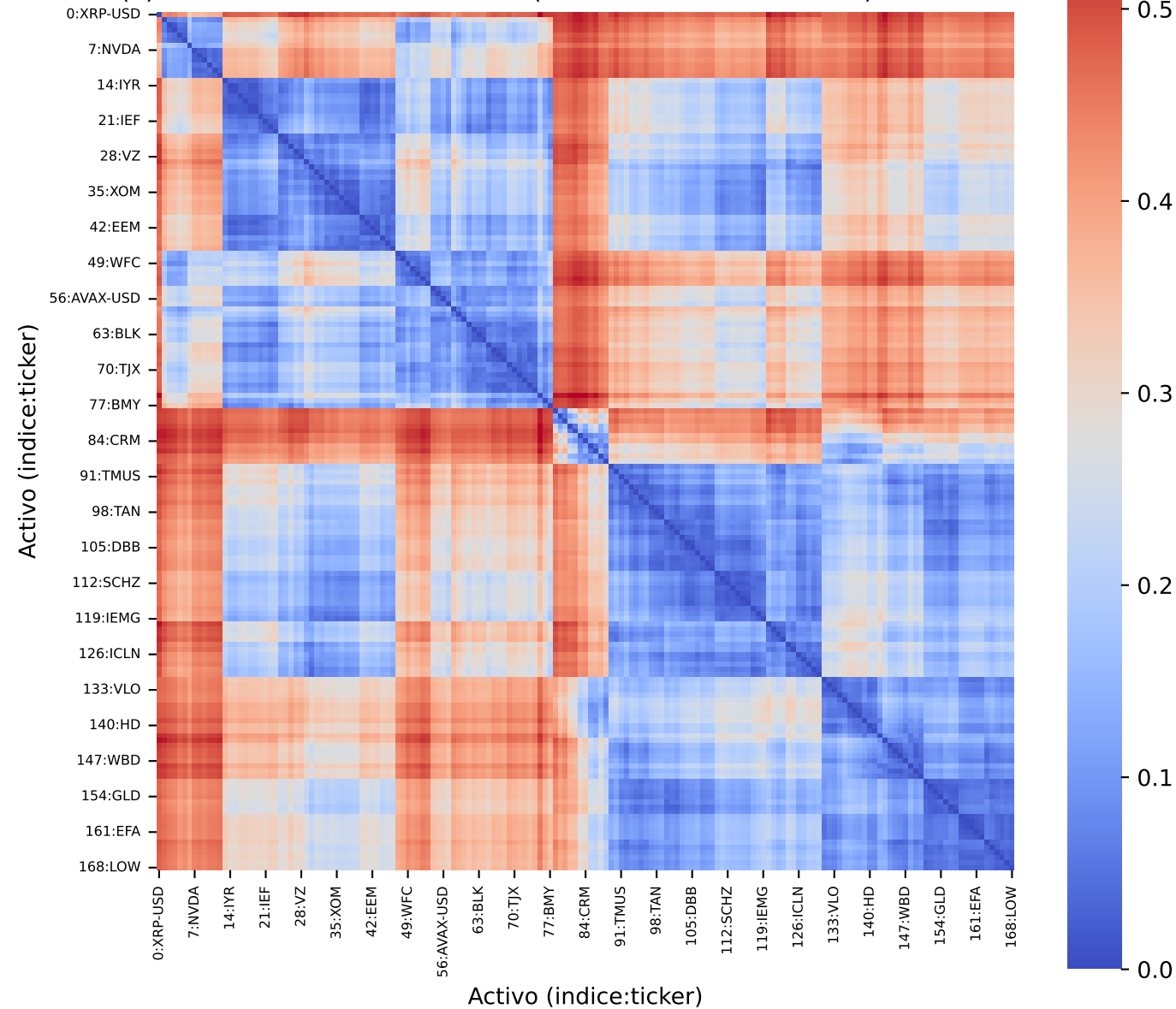
(b) Matriz de Distancia Cuántica (Ordenación HRP Cuántica) — Permutado
