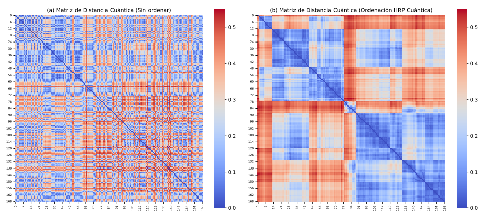
Figura 6.4: Figura de distancias cuánticas obtenida en este trabajo.
