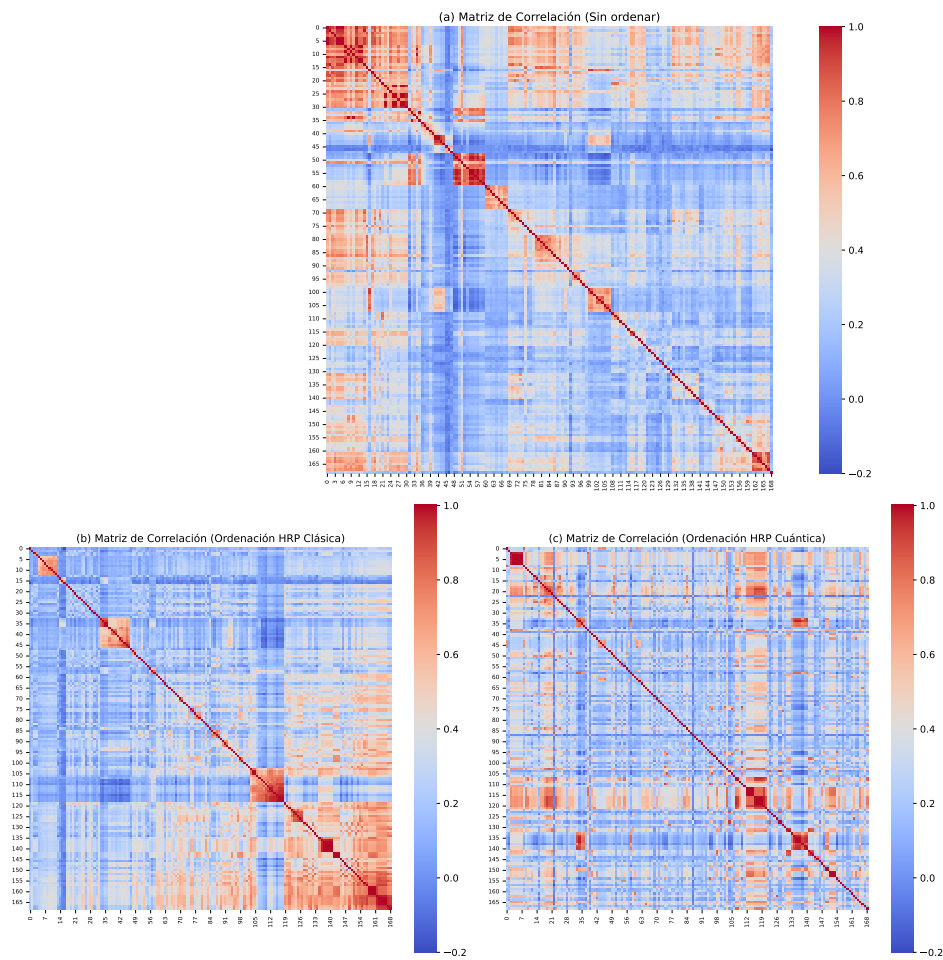
Figura 6.3: Figura de correlaciones reordenadas obtenida en este trabajo con el mismo esquema metodológico.
