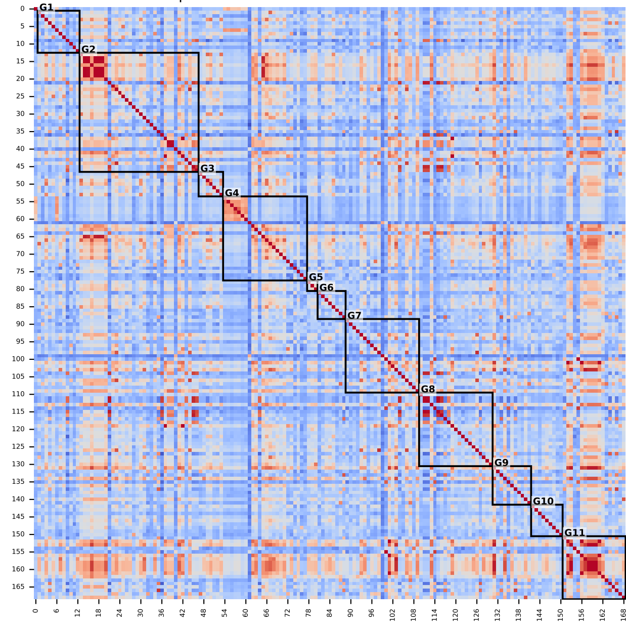
Bloques detectados en ordenación HRP cuántica
