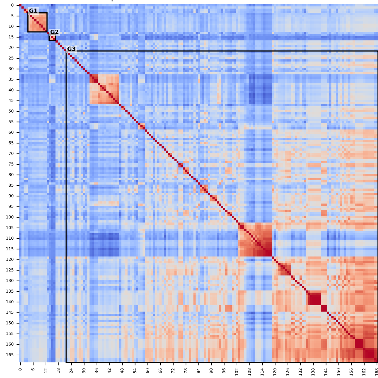
Bloques detectados en ordenación HRP clásica
