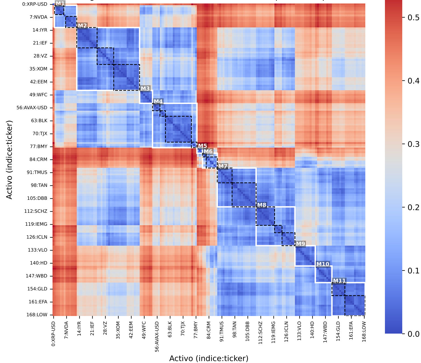
Fig.4(b) Distancia cuántica ordenada con bloque/subbloque
