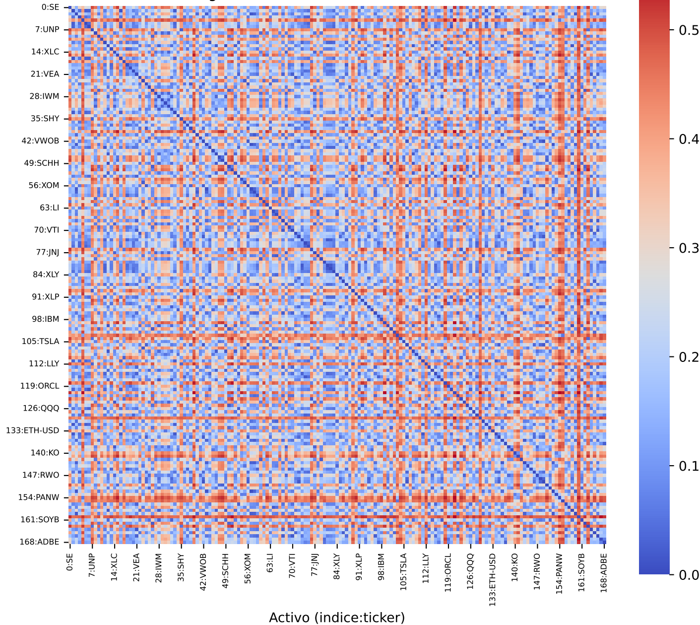
Fig.4(a) Distancia cuántica sin ordenar
