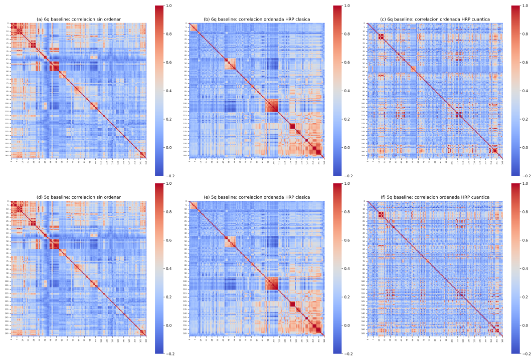
Figura 6.7: La estructura de bloques cuasi-diagonales es equivalente en ambas configuraciones. a) Matriz de correlación sin ordenar con 6 qubits, b) Matriz de correlación ordenada por HRP clásico con 6 qubits, c) Matriz de distancia cuántica ordenada por HRP Cuántico con 6 qubits, d) Matriz de correlación sin ordenar con 5 qubits, e) Matriz de correlación ordenada por HRP clásico con 5 qubits, f) Matriz de distancia cuántica ordenada por HRP Cuántico con 5 qubits.
