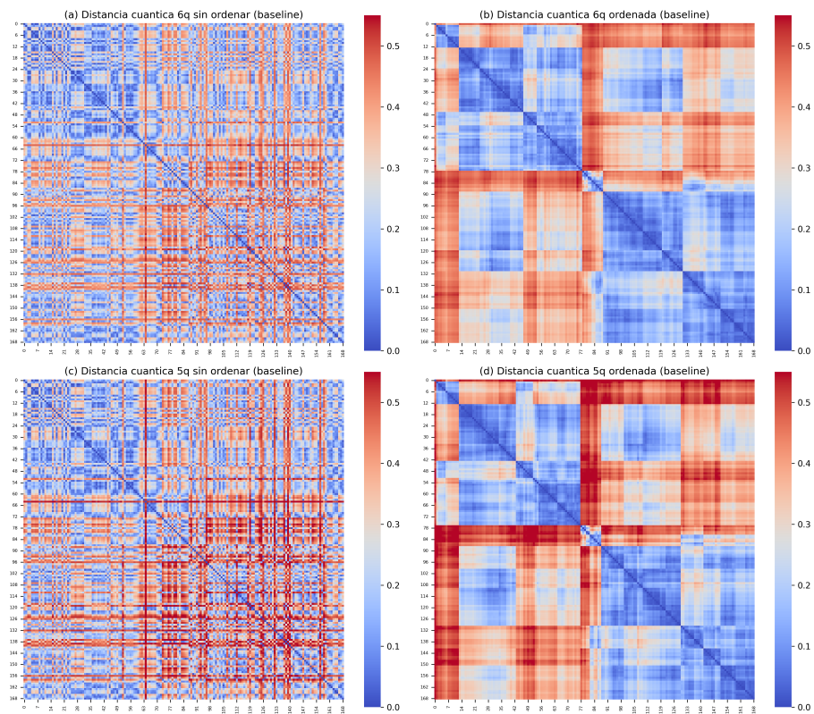
Figura 6.8: a) Matriz de distancia cuántica sin ordenar con 6 qubits, b) Matriz de distancia cuántica ordenada por QHRP con 6 qubits, c) Matriz de distancia cuántica sin ordenar con 5 qubits, d) Matriz de distancia cuántica ordenada por QHRP con 5 qubits.
