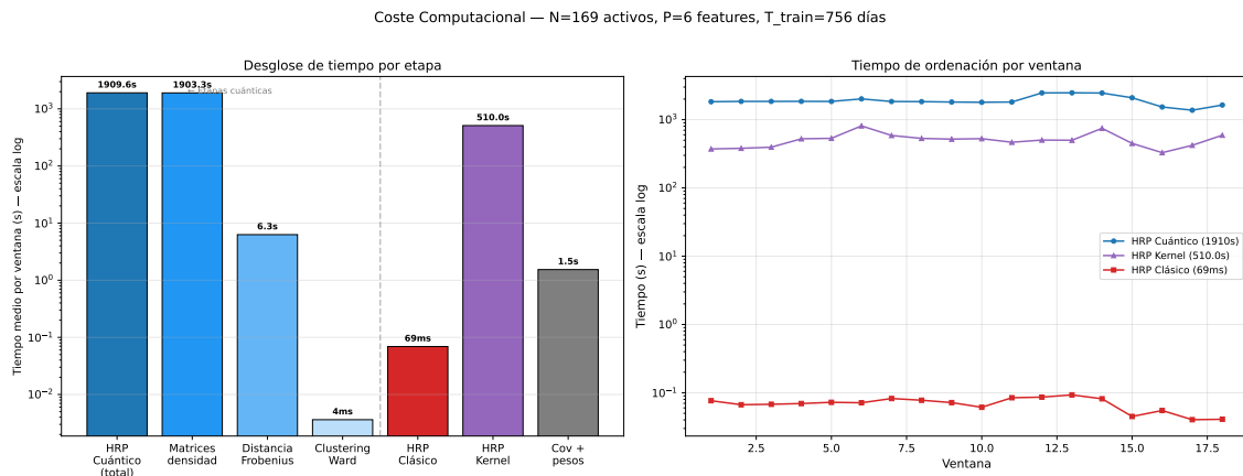
Figura 5.9: Comparativa de tiempo por método y por ventana. Se observa que la etapa dominante del enfoque cuántico es la construcción de matrices densidad, mientras que el enfoque clásico tiene coste prácticamente despreciable en la misma escala.
