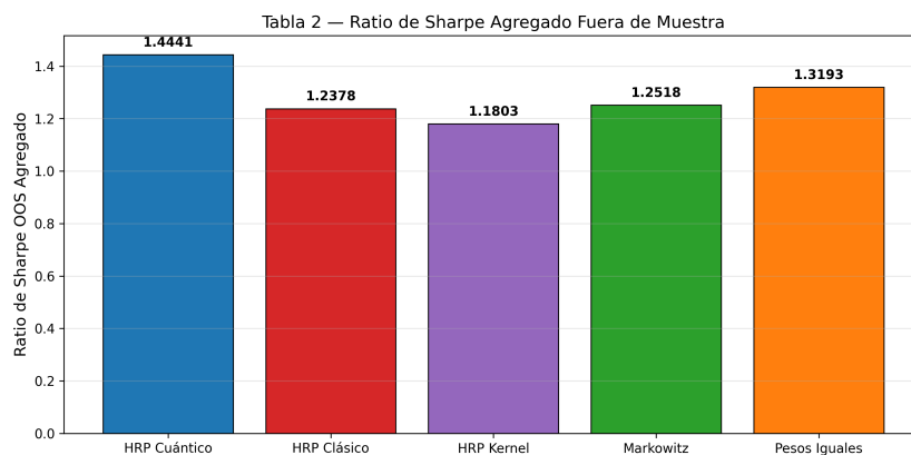
Figura 5.2: Comparación del Sharpe fuera de muestra agregado por método. Esta figura resume el rendimiento global acumulado sobre las ventanas evaluadas.
