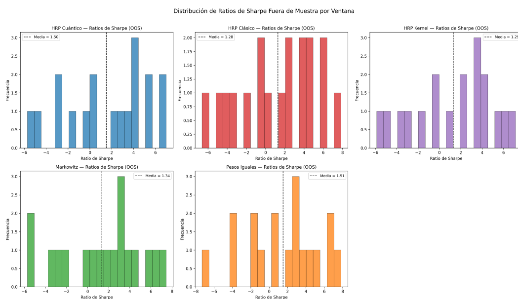
Figura 5.1: Histogramas de Sharpe y PSR por ventana para las estrategias comparadas. Permiten observar estabilidad, dispersión y sensibilidad de cada método.
