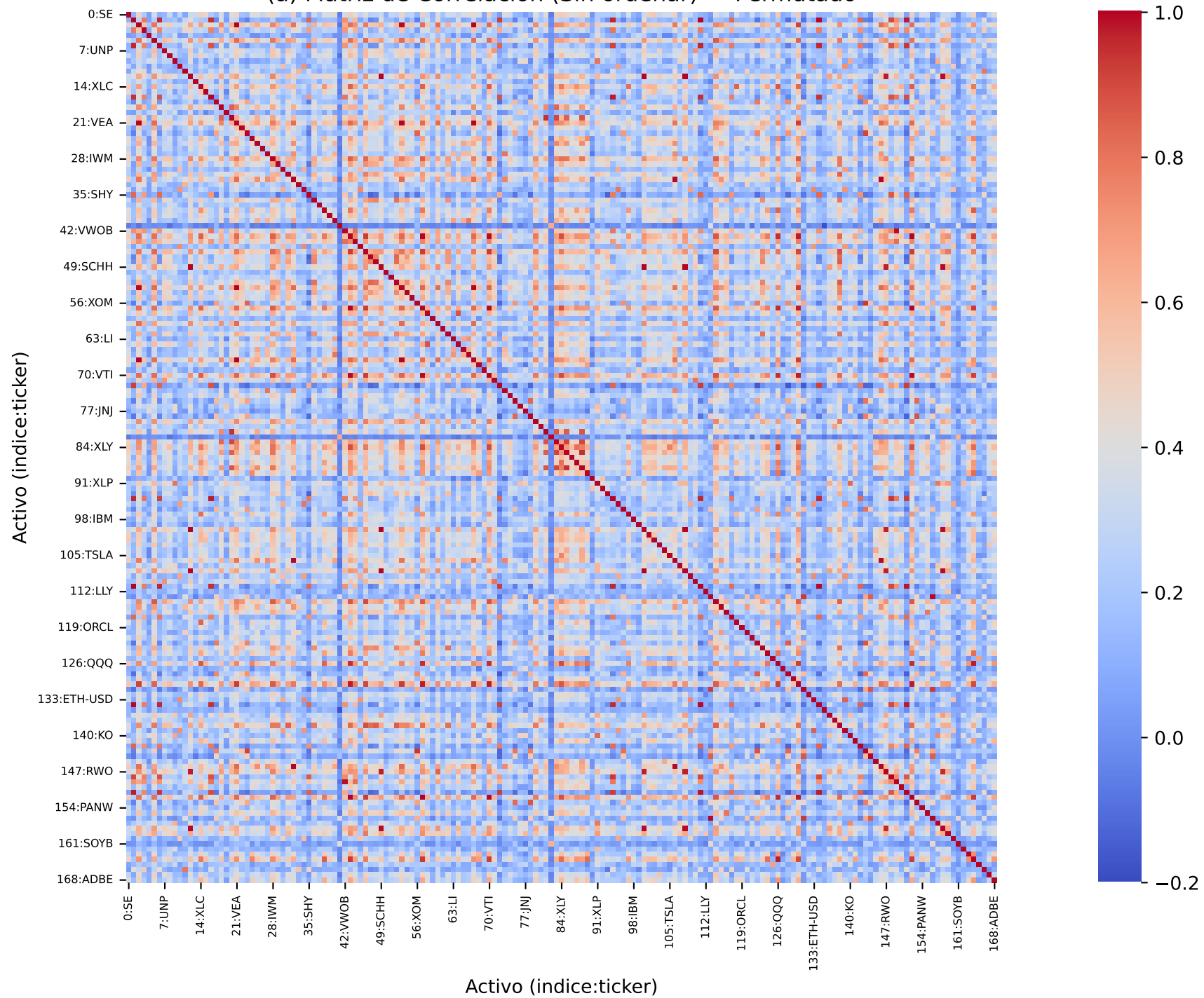
(a) Matriz de Correlación (Sin ordenar) — Permutado
