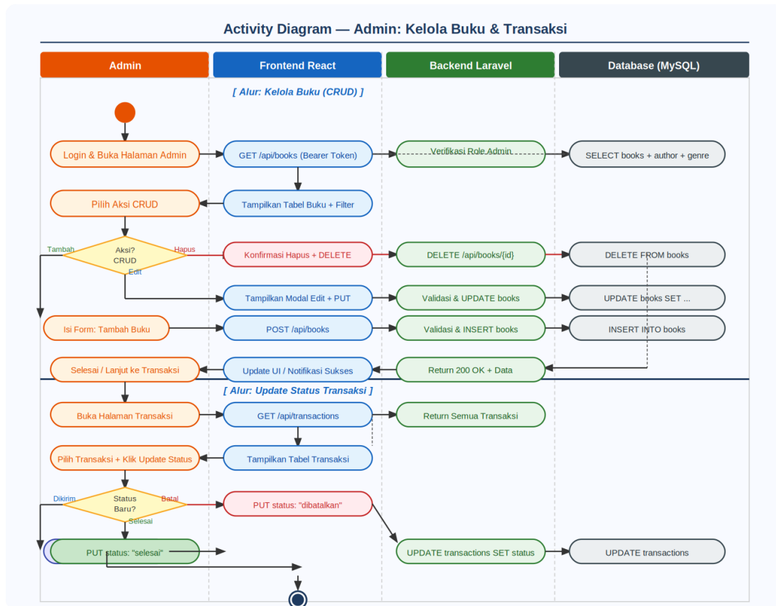
Gambar 7.3 — Activity Diagram: Admin Kelola Buku &amp; Transaksi
