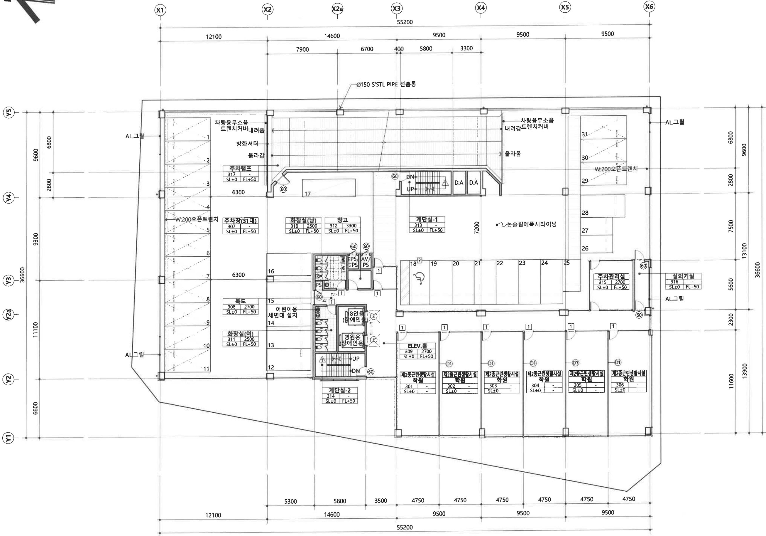
1 A 3 층 평 면 도 SCALE : 1/250
