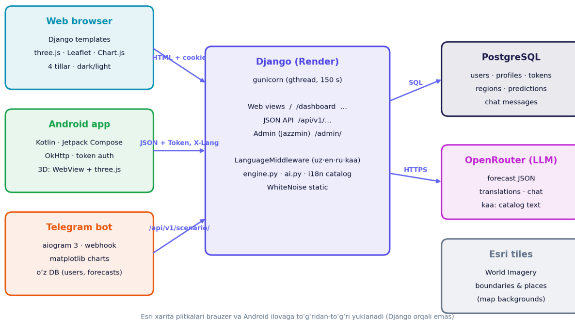
1-rasm. Tizim arxitekturas
