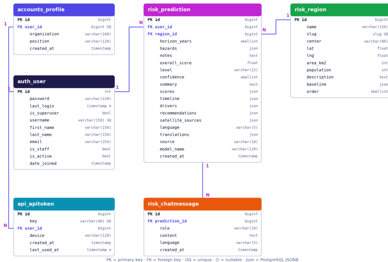
2-rasm. ER-diagramma (jadvallar va bog'lanishlar)
