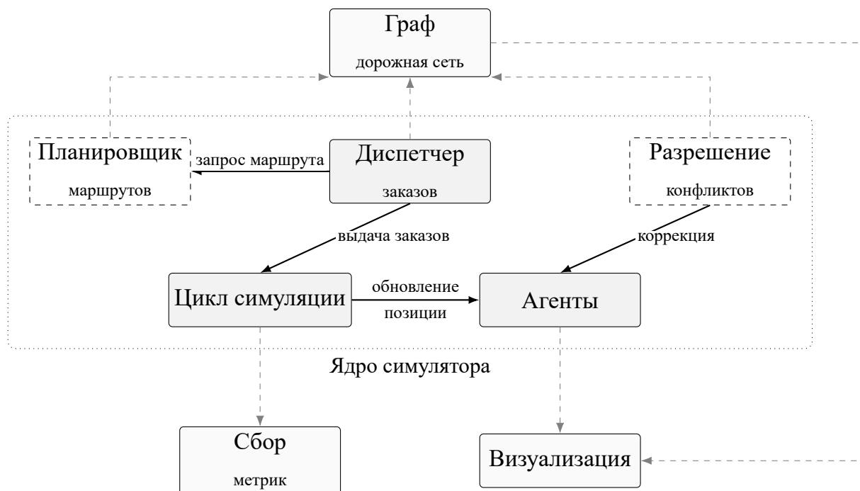
Рисунок 6 – Структура симулятора и взаимодействие основных компонентов.
