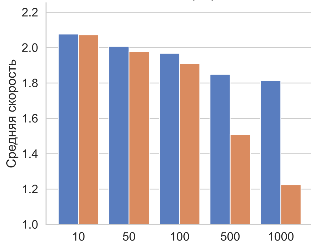
Малый граф
