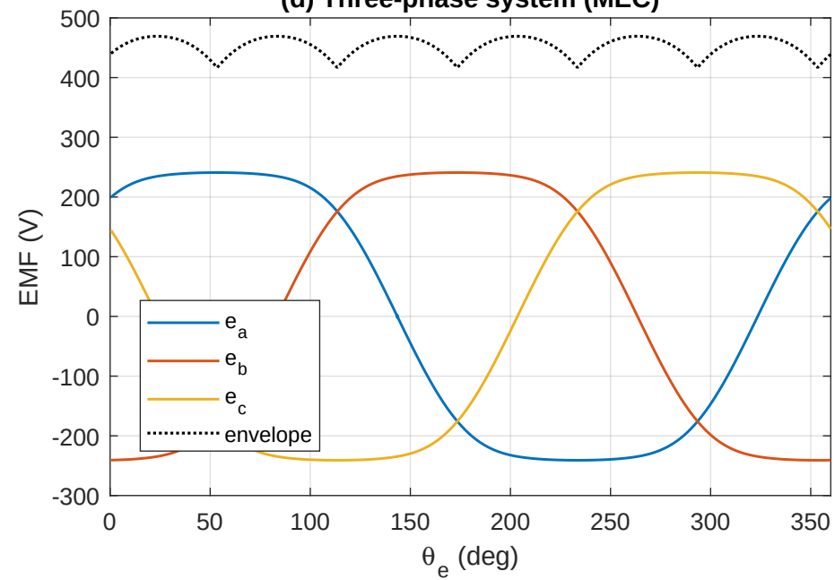
(d) Three-phase system (MEC)
