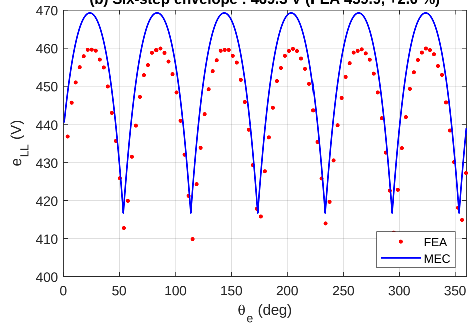
(b) Six-step envelope : 469.3 V (FEA 459.9, +2.0 %)
