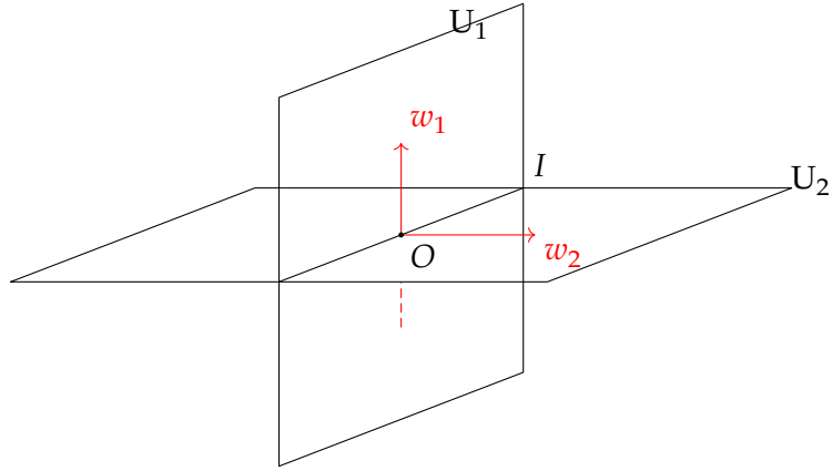
Figura 6.10: Sottospazi ortogonali
