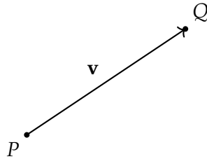
Figura 6.1: Vettore tra due punti
