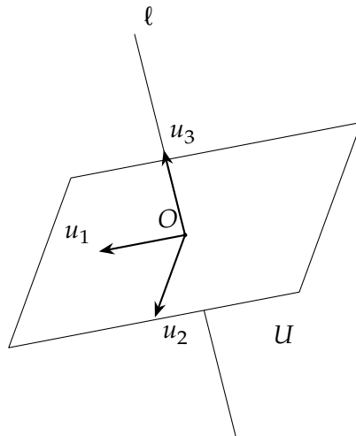
Figura 6.7: Caso 2
