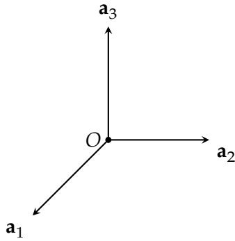
Figura 6.2: I versori degli assi
