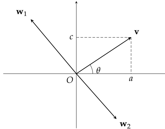
Figura 4.2: Esempio
