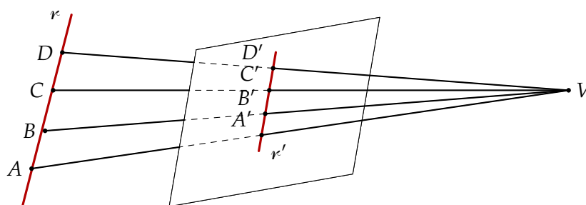
Figura 7.6: Proiezione centrale
