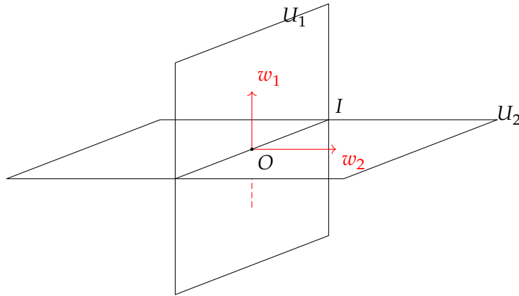
Figura 6.9: Sottospazi ortogonali
