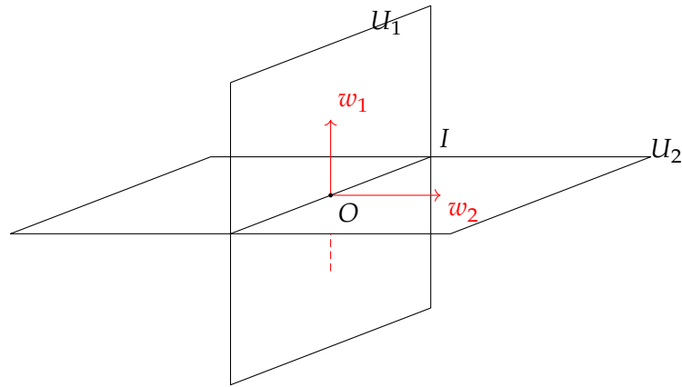
Figura 6.9: Sottospazi ortogonali
