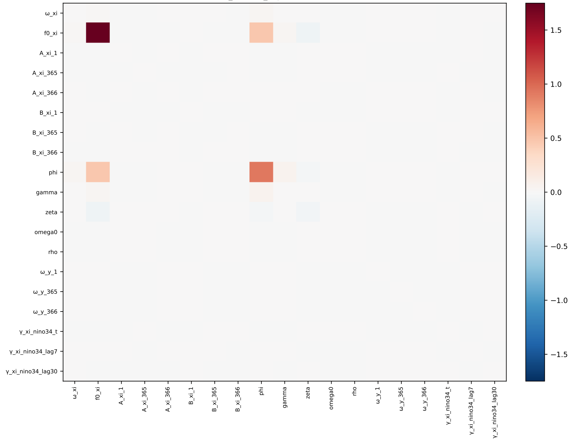
xi_nino34_lags — covariance
