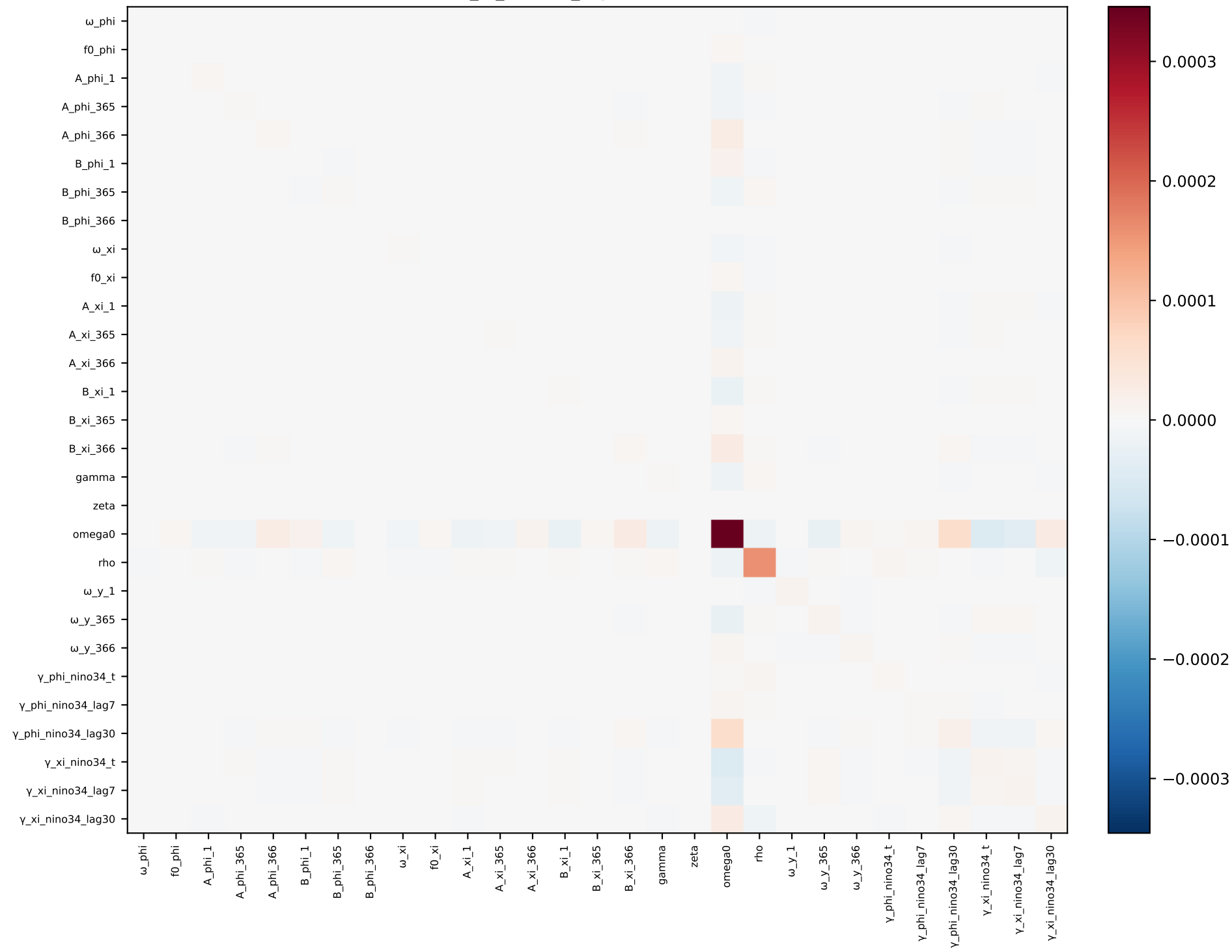
phi_xi_nino34_lags — covariance
