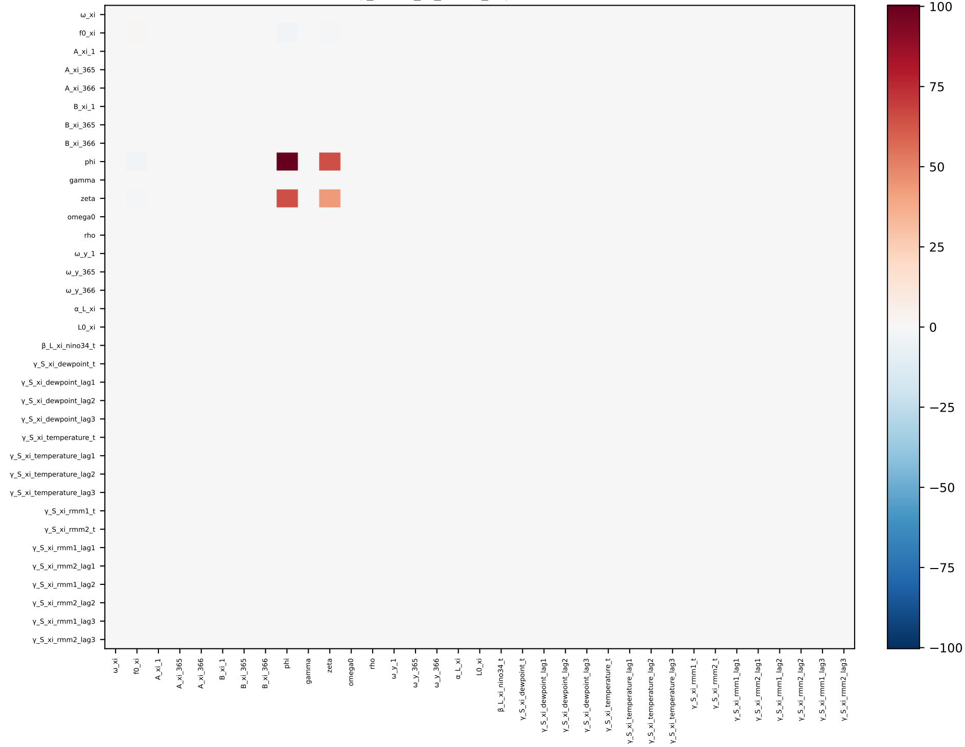
long_short_xi_short_lags — covariance
