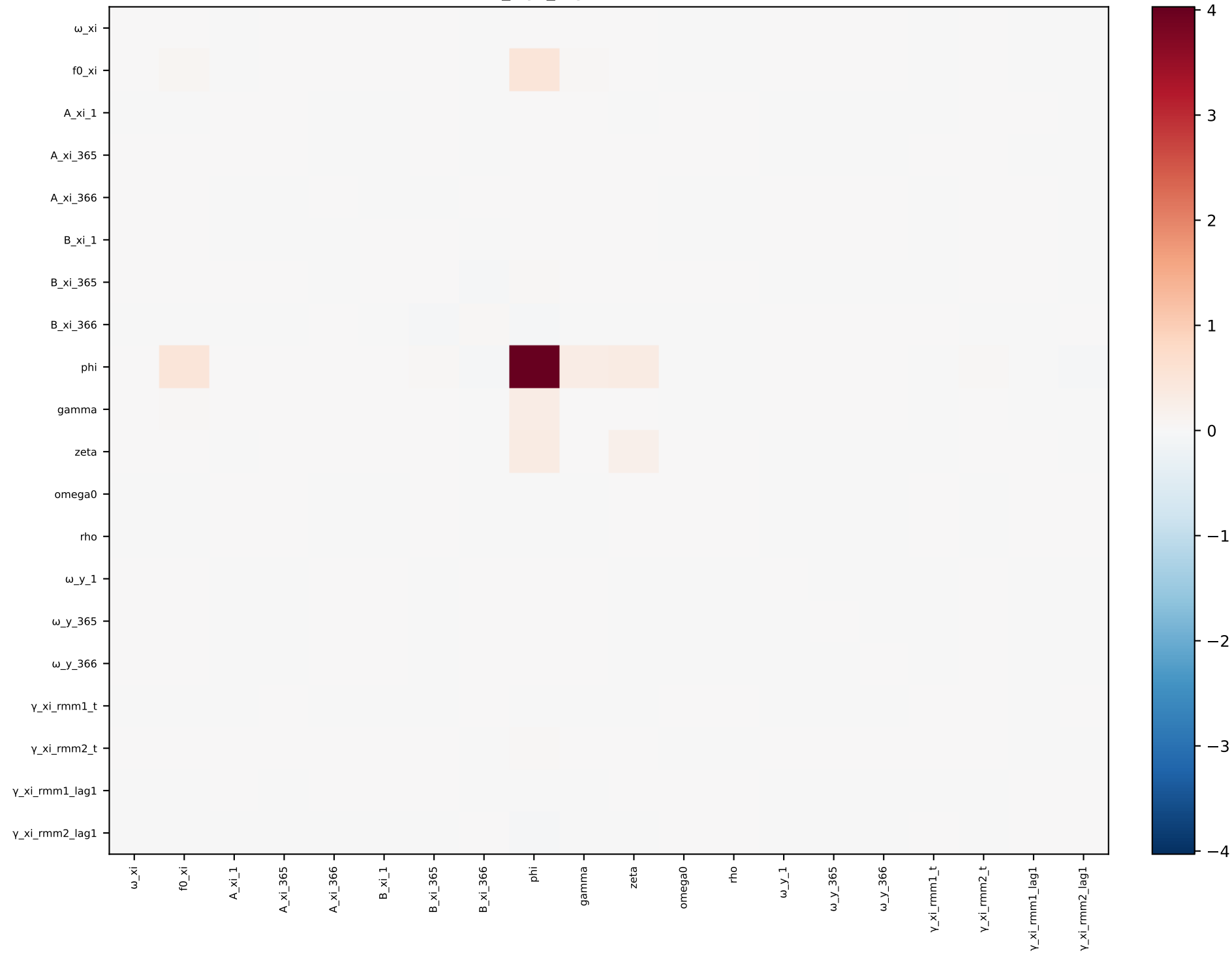
xi_mjo_lag1 — covariance
