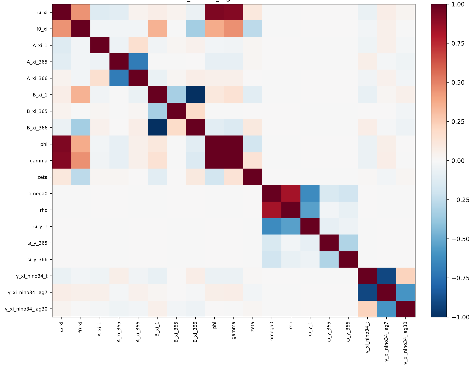
xi_nino34_lags — correlation
