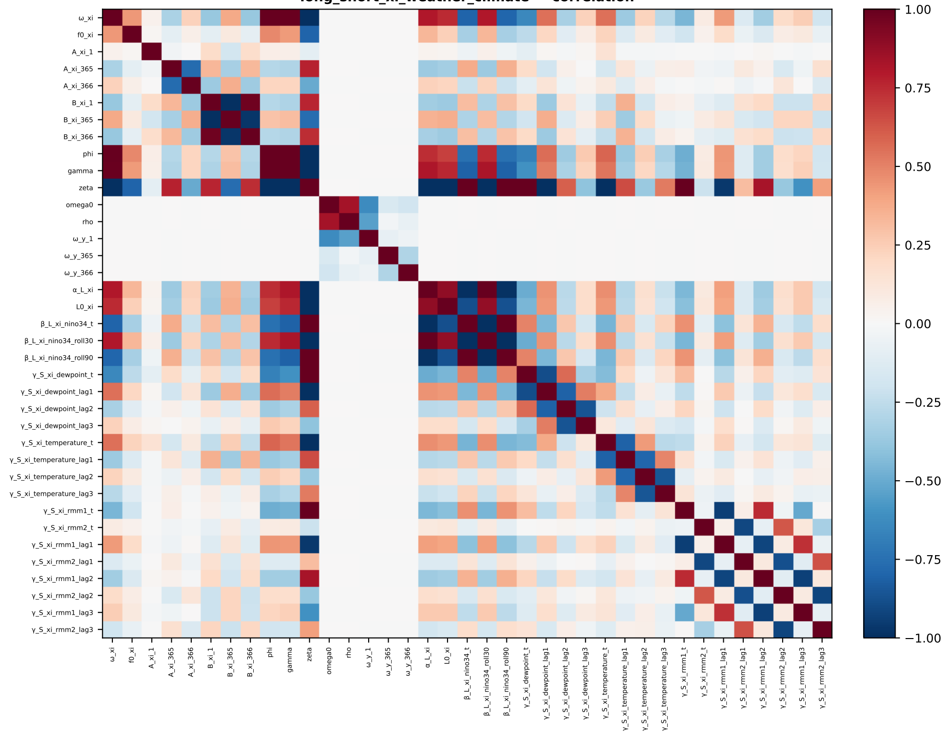
long_short_xi_weather_climate — correlation
