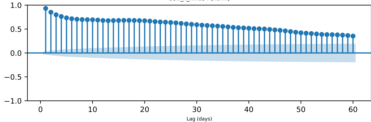
temp_x_nino34 (norm)
