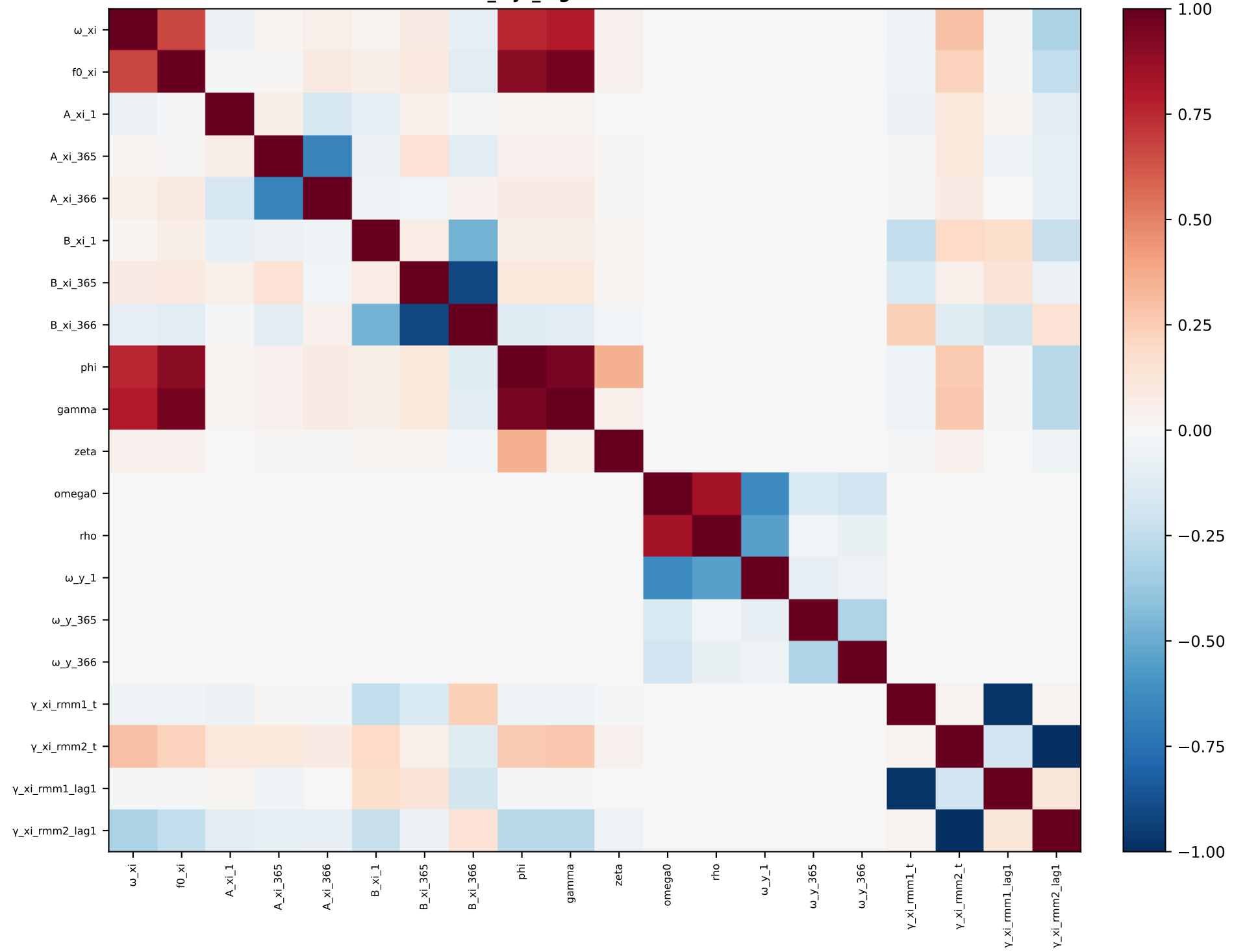
xi_mjo_lag1 — correlation
