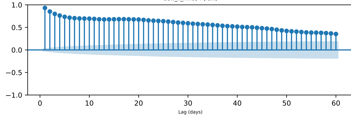
temp_x_nino34 (raw)
