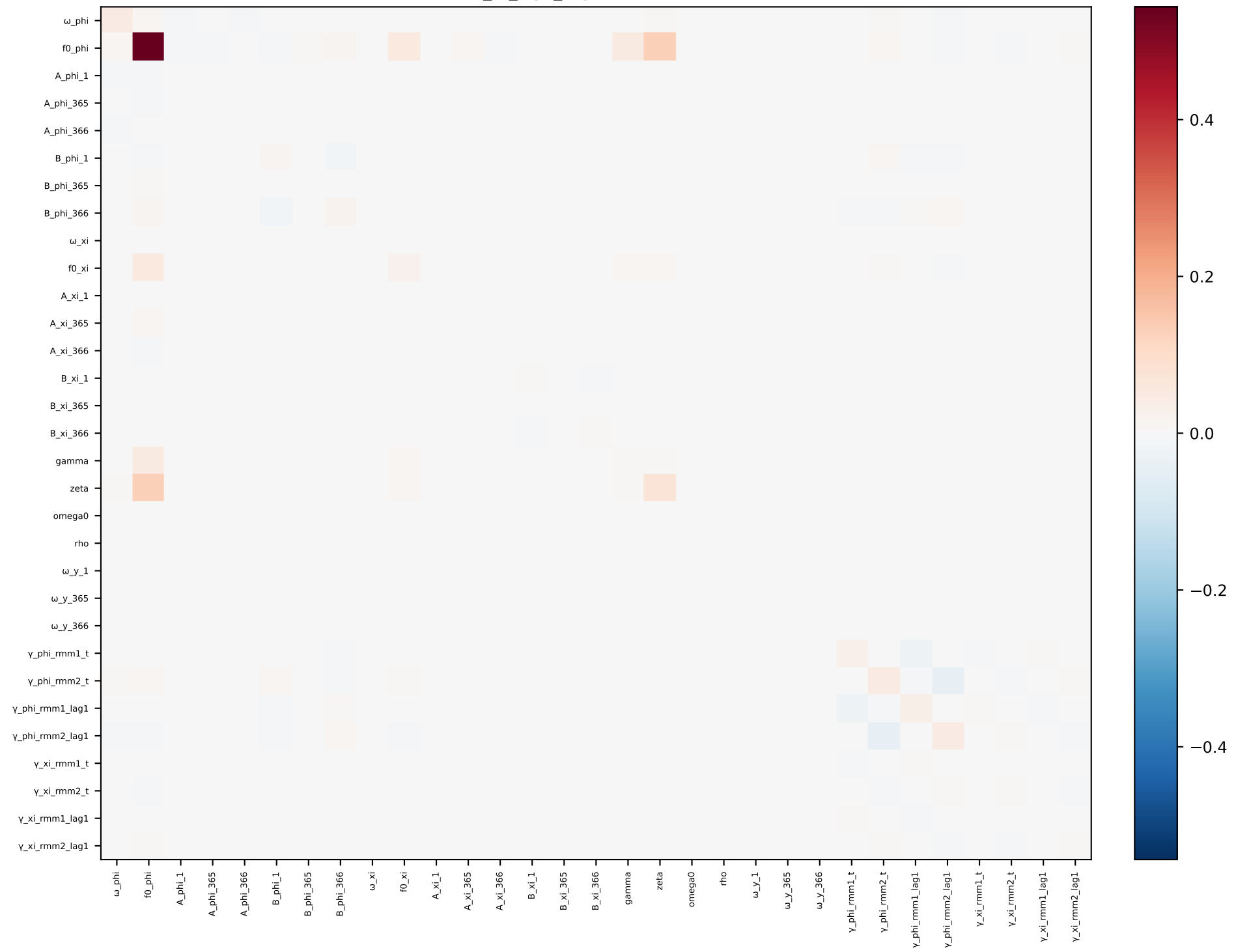
phi_xi_mjo_lag1 — covariance
