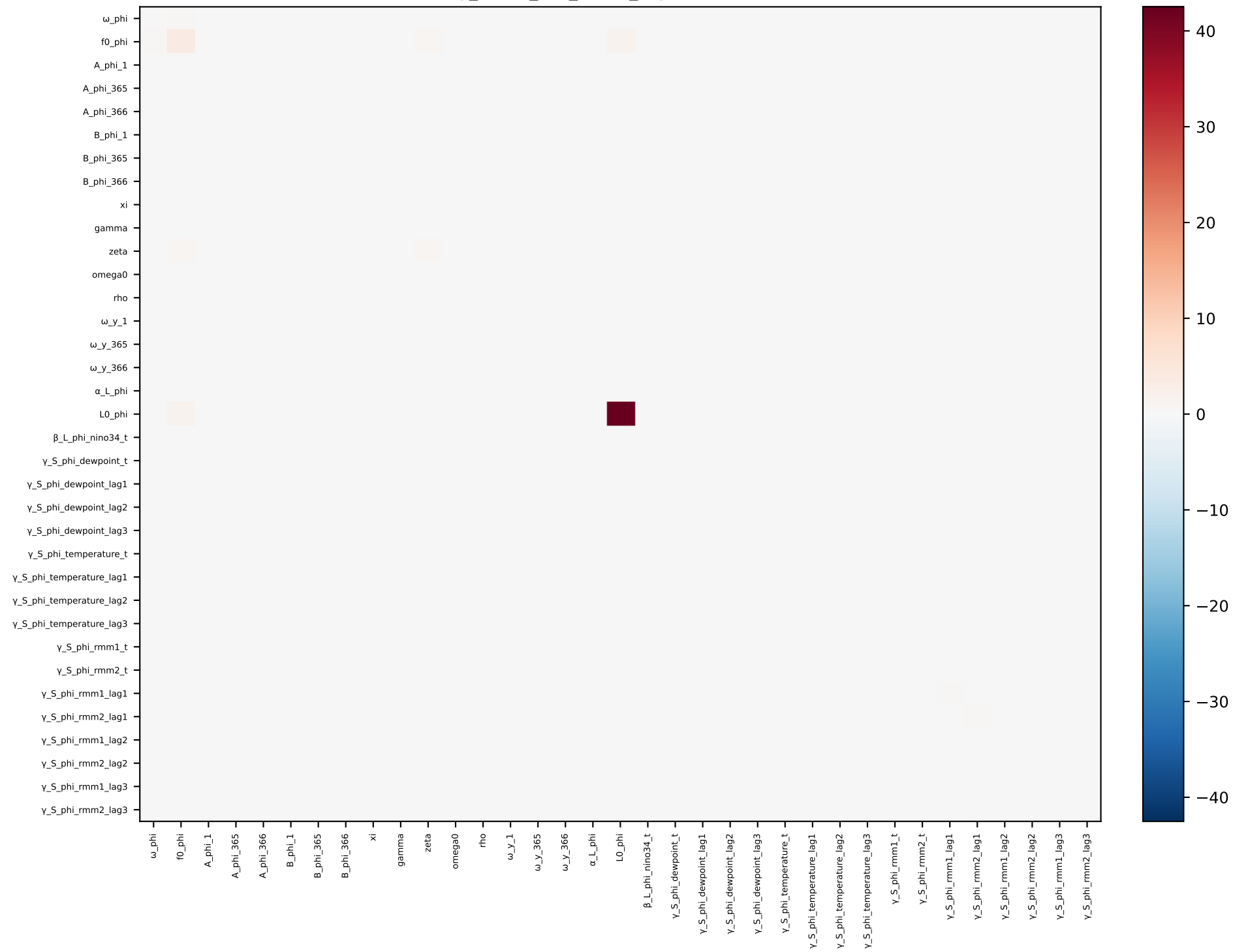
long_short_phi_short_lags — covariance
