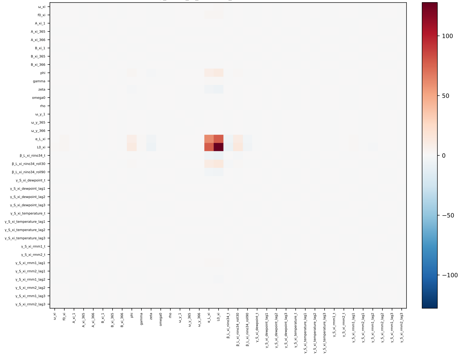
long_short_xi_weather_climate — covariance
