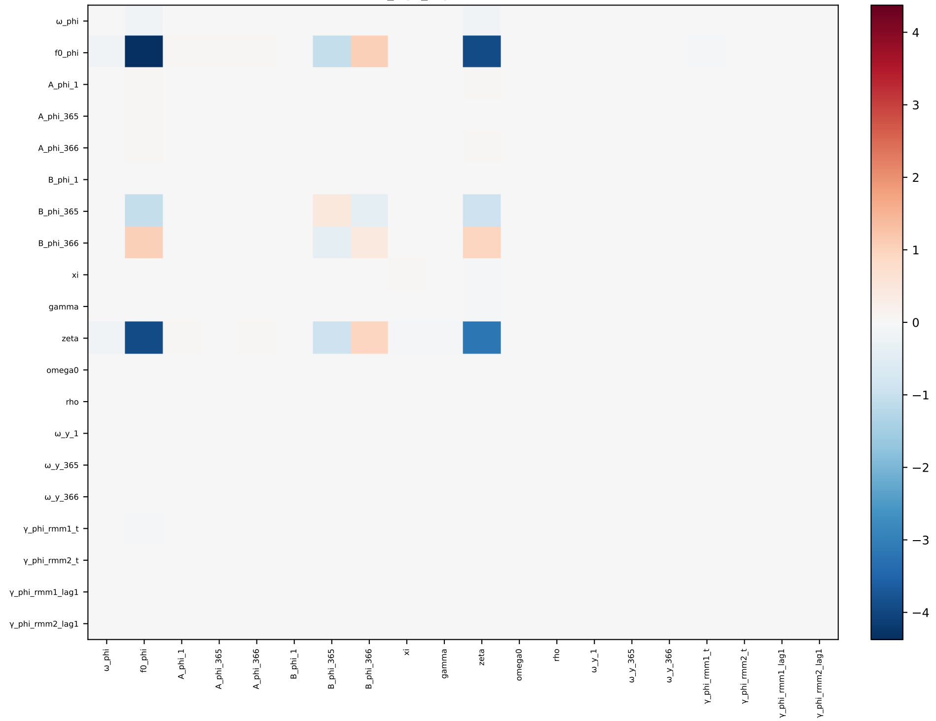
phi_mjo_lag1 — covariance
