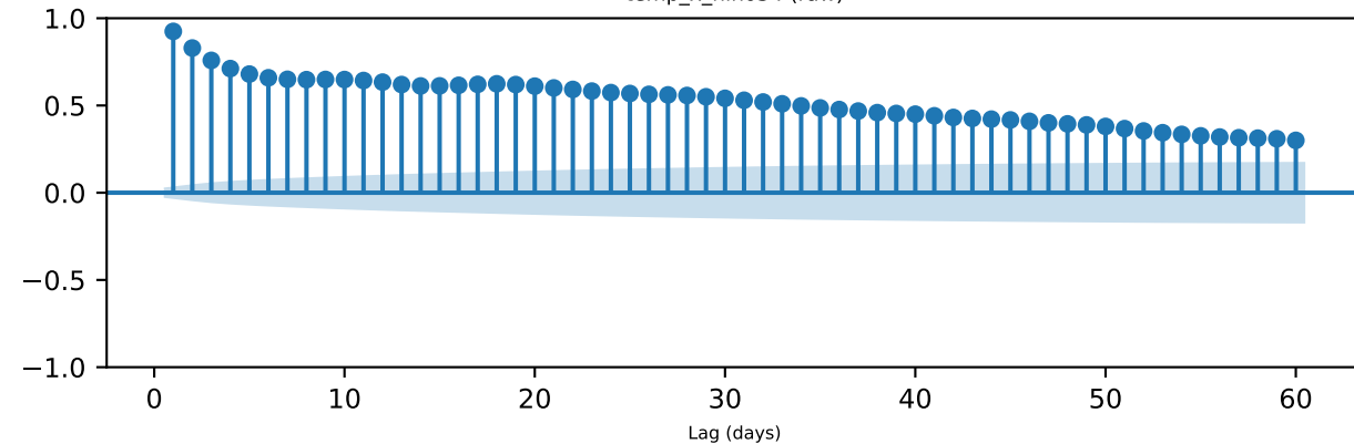
temp_x_nino34 (raw)
