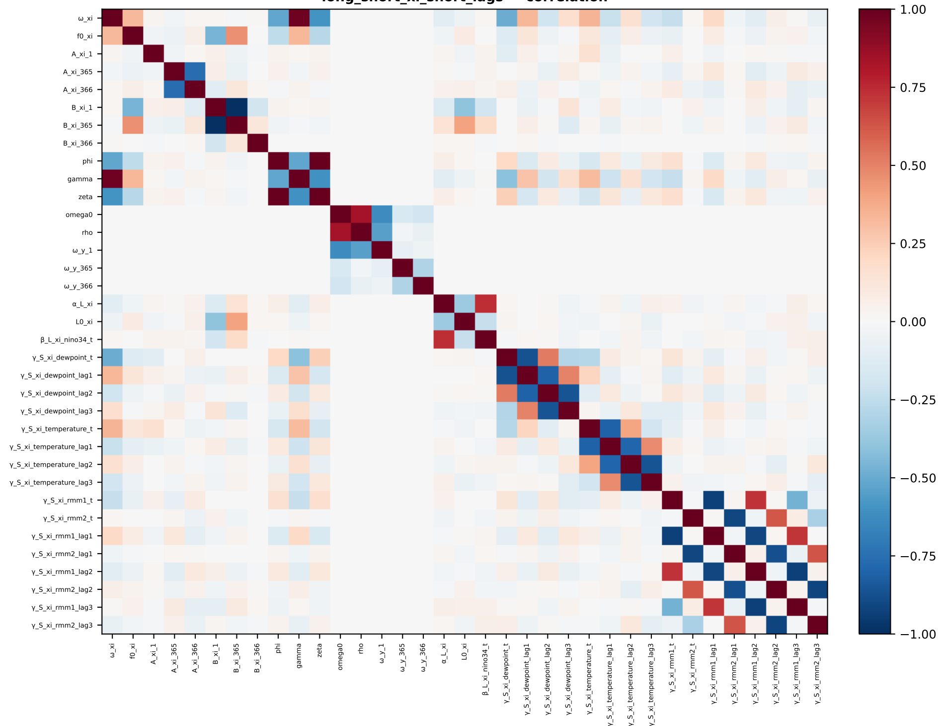
long_short_xi_short_lags — correlation
