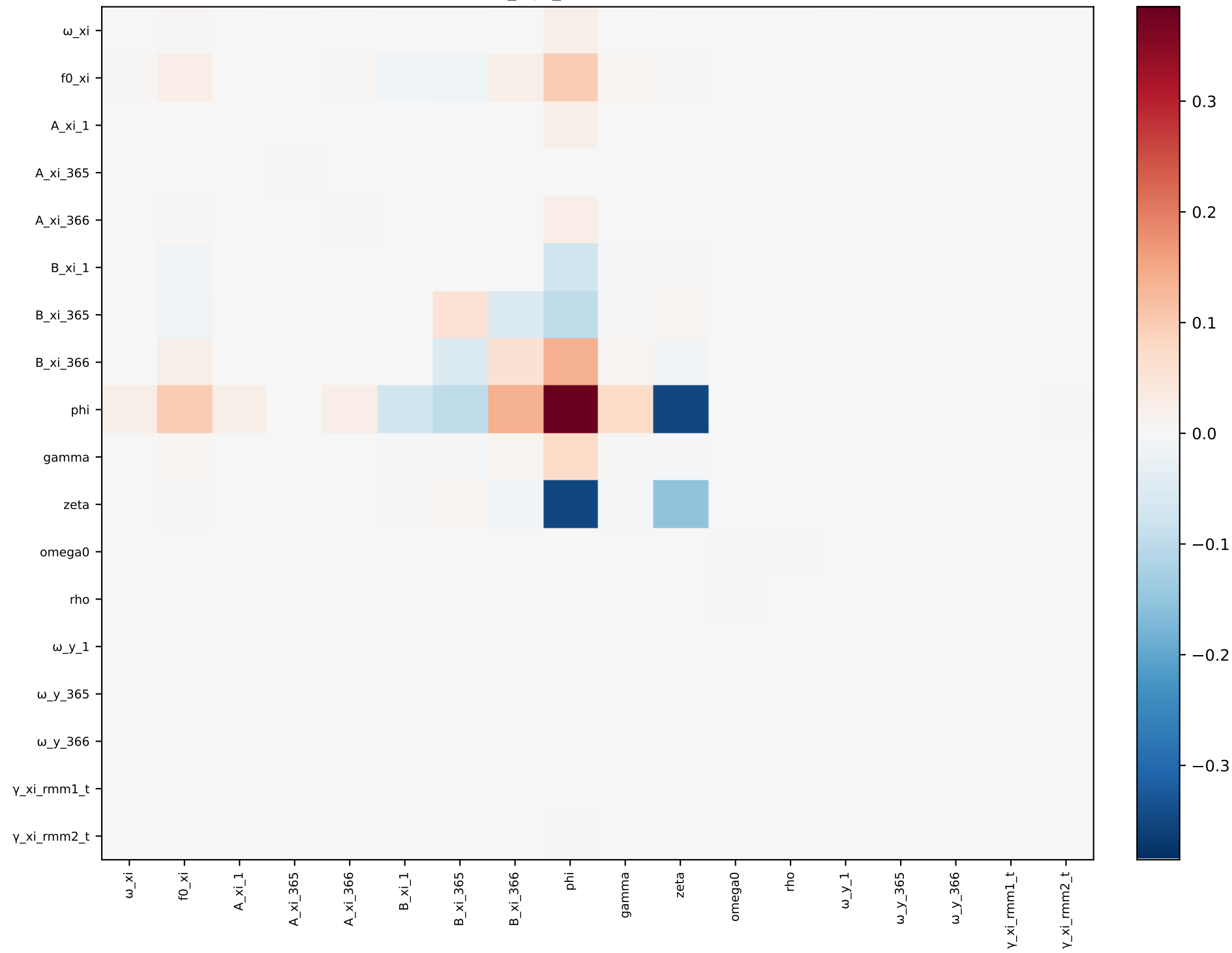
xi_mjo_t — covariance
