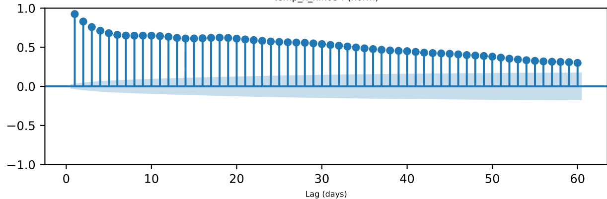
temp_x_nino34 (norm)
