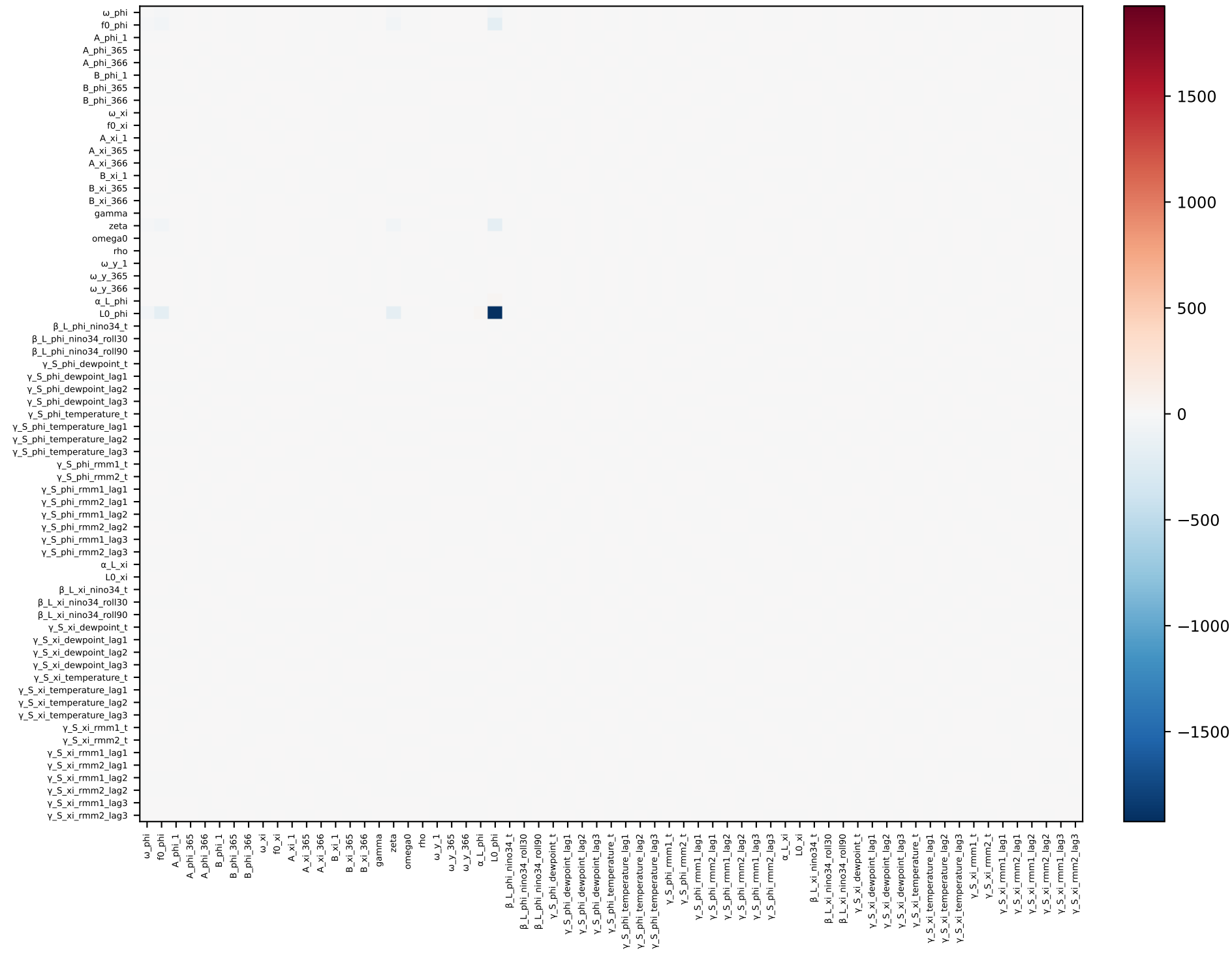
long_short_phi_xi_weather_climate — covariance
