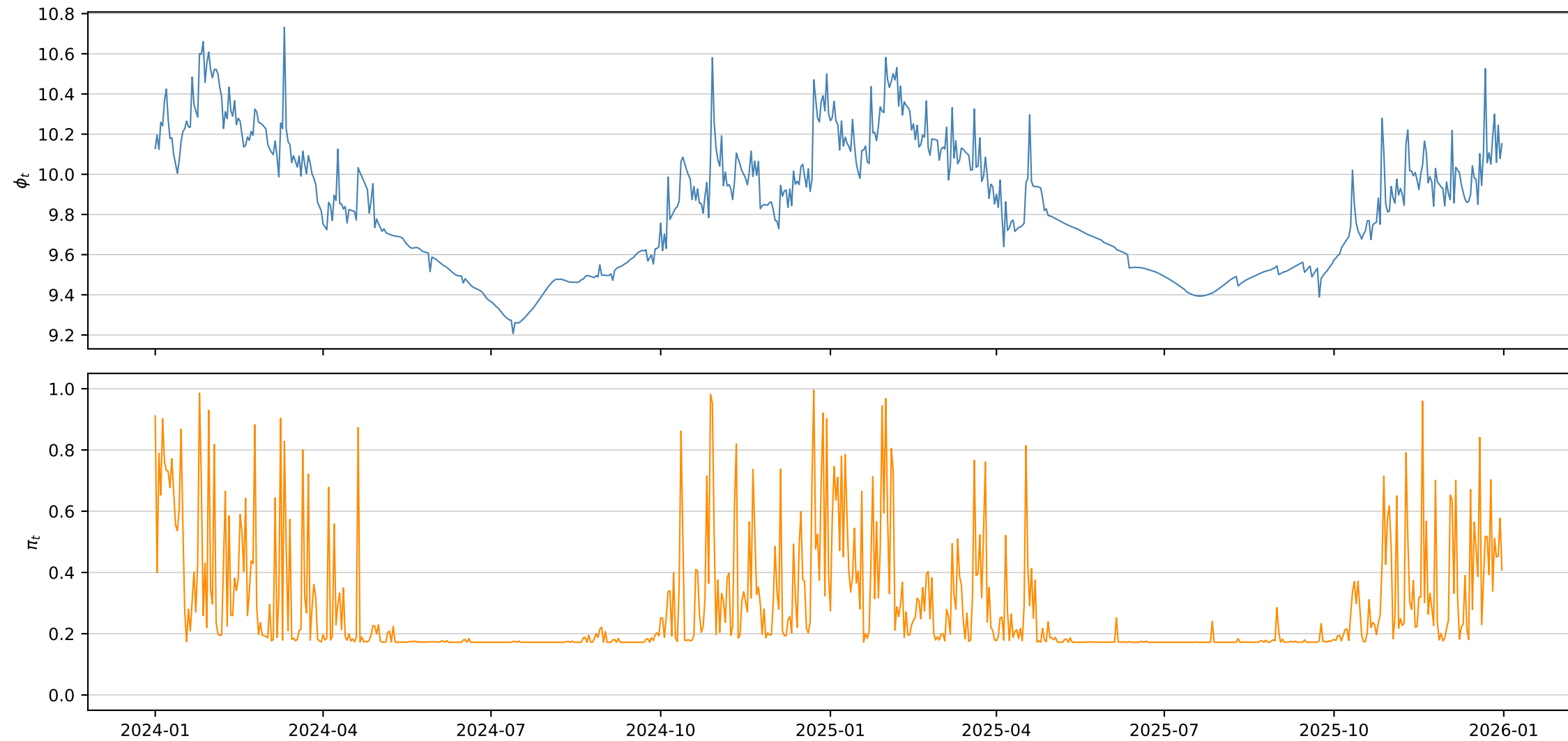
phi_mjo_lag1 — filtered states (OOS)
