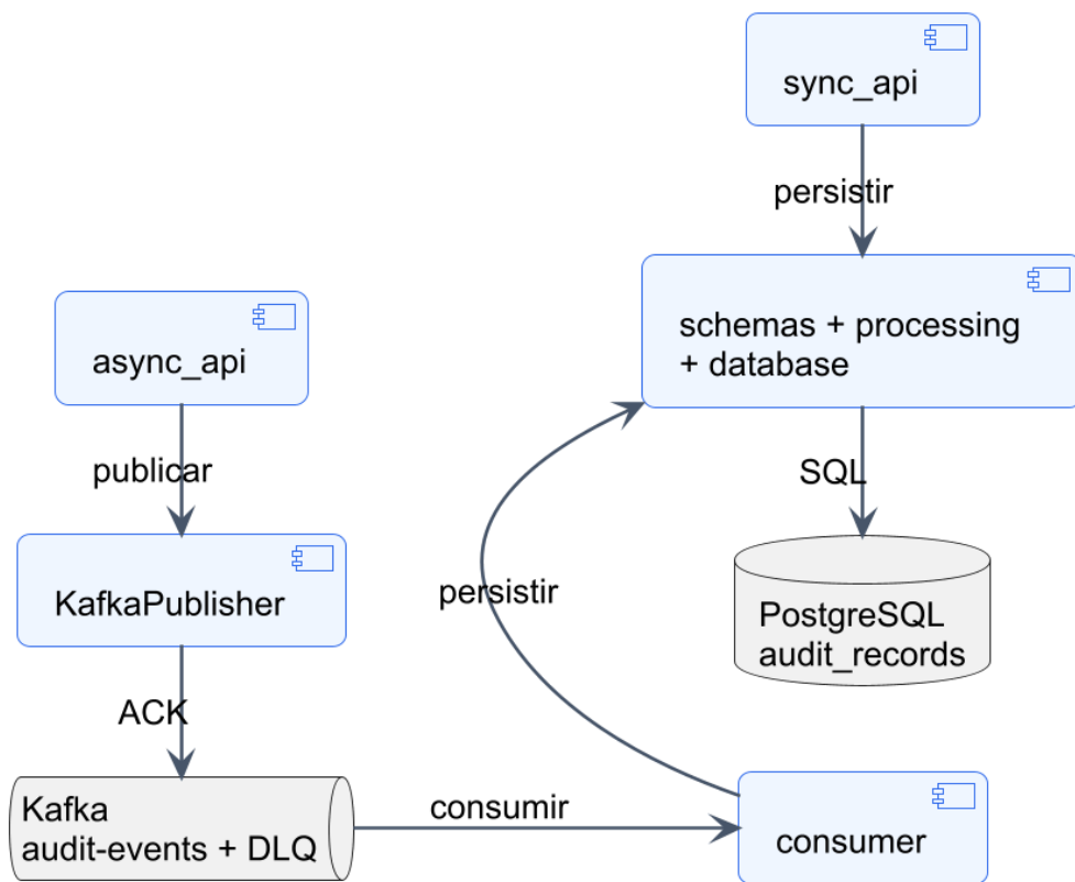
FIGURA 11 – Dependências principais dos componentes operacionais
