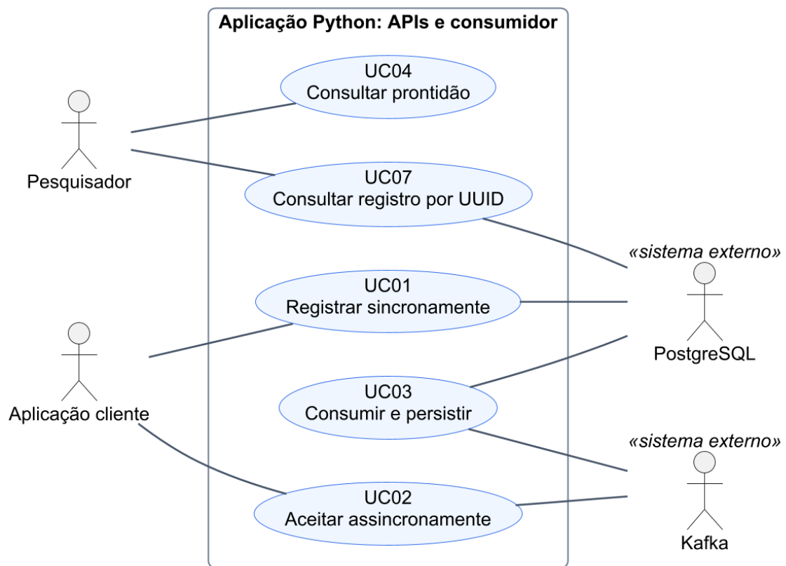
FIGURA 2 – Casos de uso da aplicação operacional
