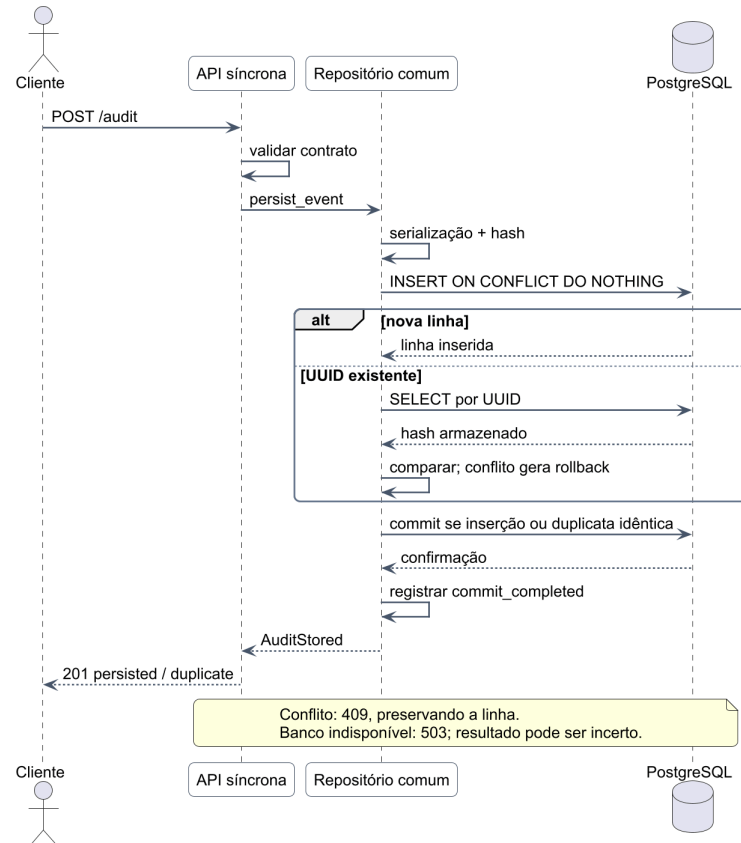
FIGURA 9 – Sequência síncrona com inserção idempotente
