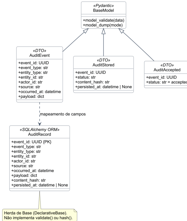
FIGURA 7 – Classes de contrato e persistência
