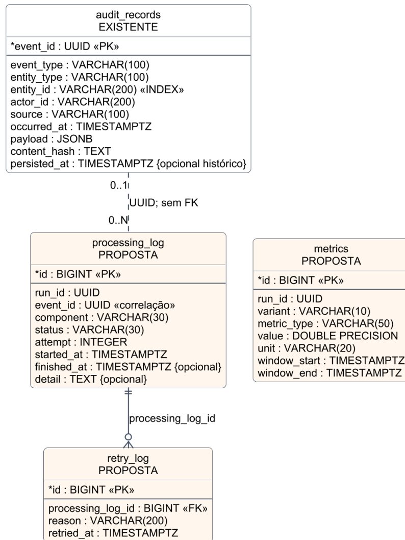
FIGURA 18 – Modelo lógico da extensão proposta, separado do esquema atual
