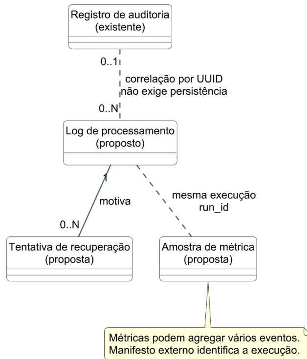
FIGURA 16 – Modelo conceitual da extensão de observabilidade proposta
