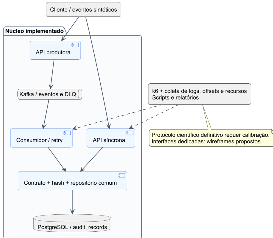
FIGURA 1 – Visão geral e delimitação do ambiente experimental
