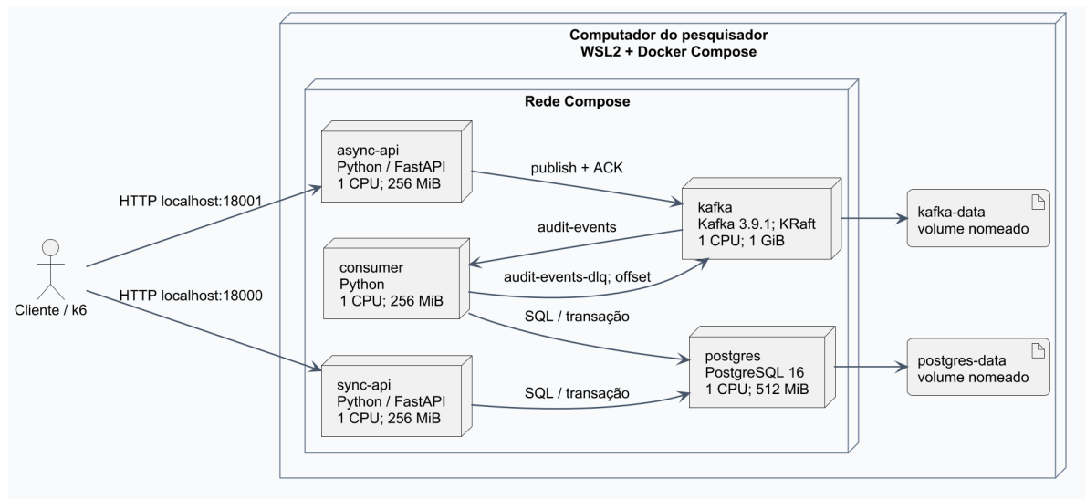
FIGURA 14 – Implantação real do protótipo no Docker Compose
