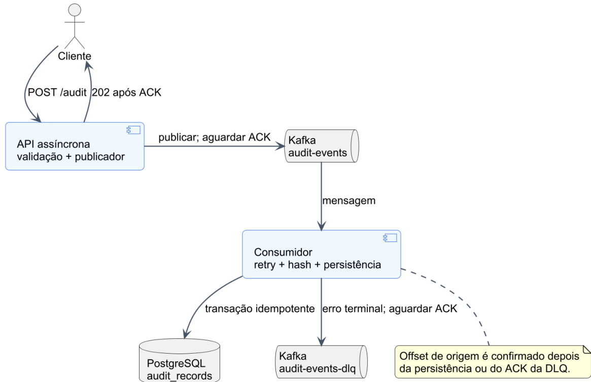
FIGURA 13 – Arquitetura da variante assíncrona e DLQ
