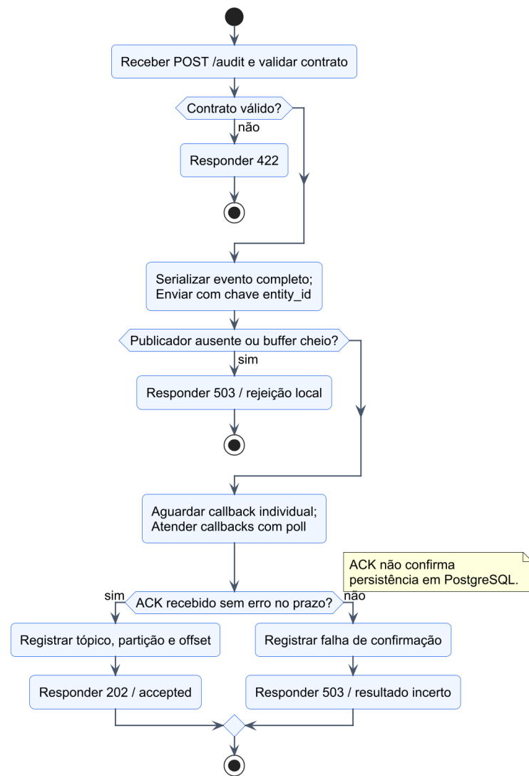
FIGURA 5 – Atividade da API produtora e confirmação de publicação
