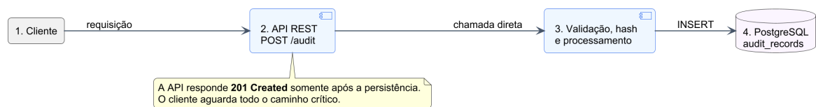
FIGURA 12 – Arquitetura da variante síncrona
