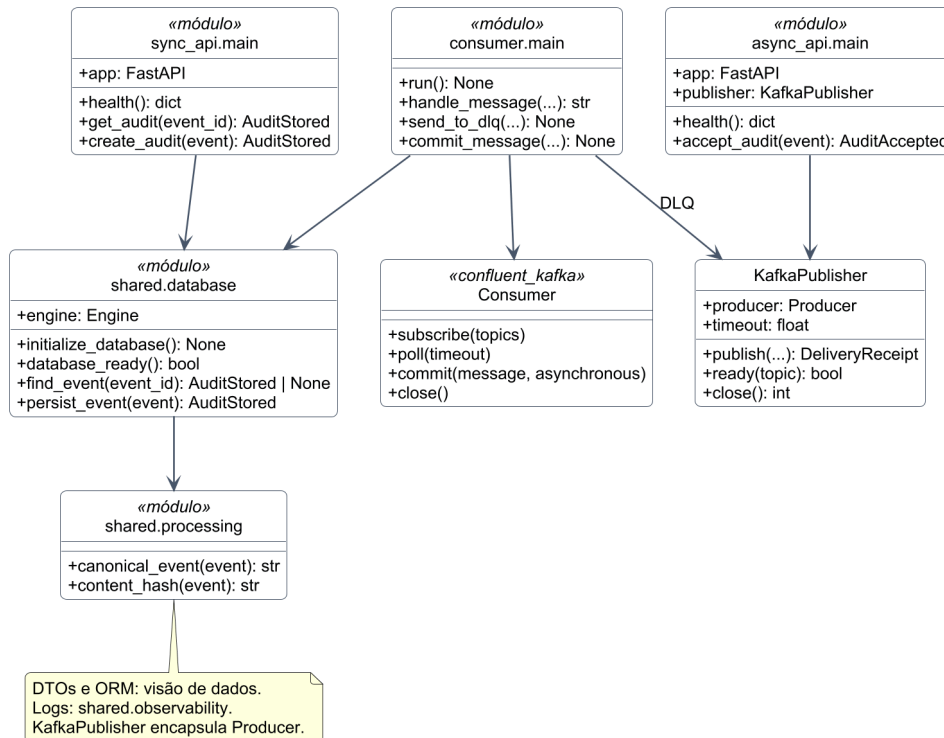
FIGURA 8 – Módulos de aplicação e publicador Kafka
