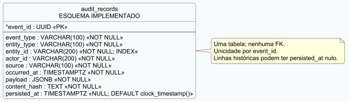
FIGURA 17 – Modelo lógico do banco implementado
