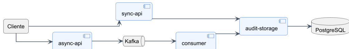
FIGURA 1 – Visão geral dos caminhos síncrono e assíncrono em Java
