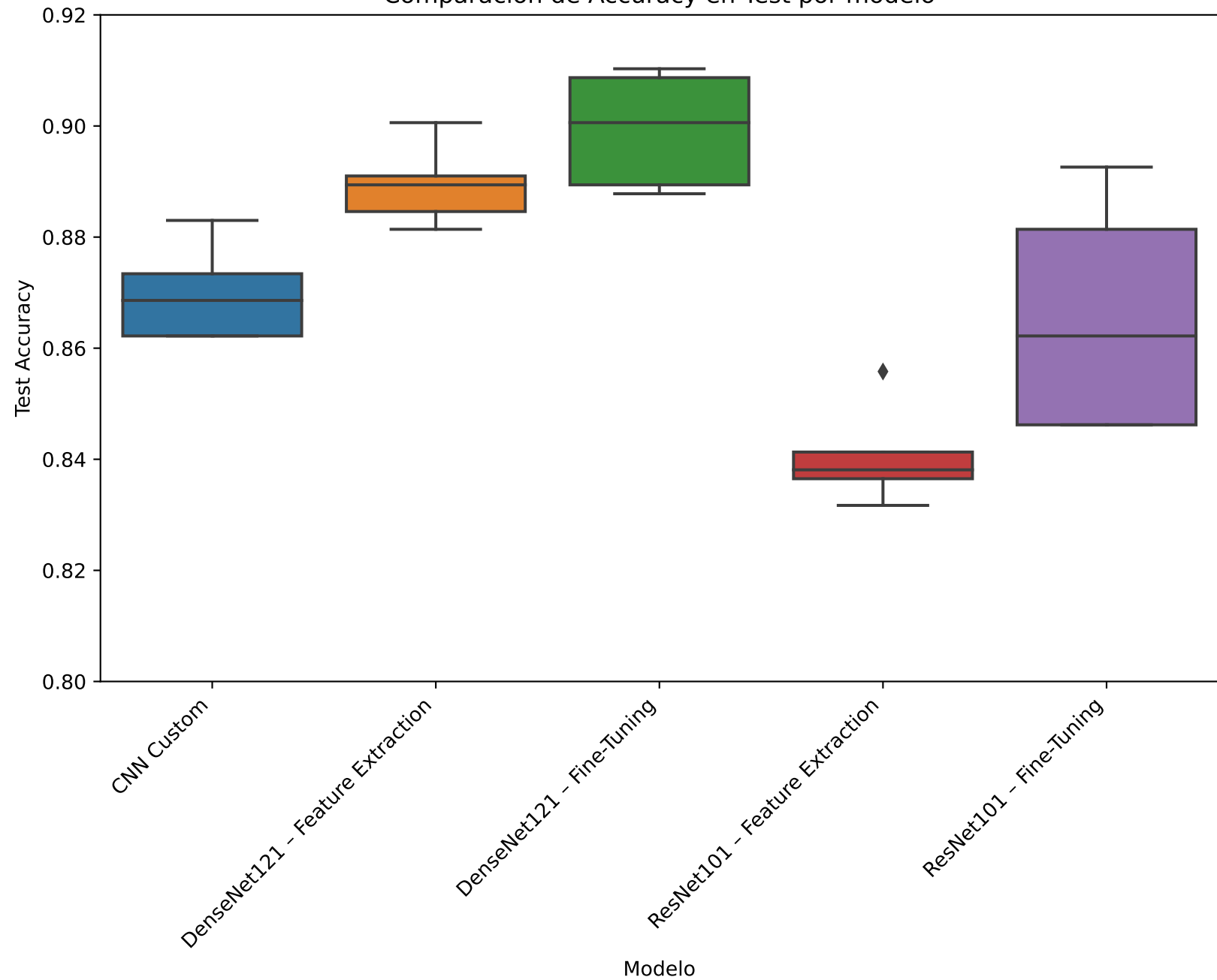
Comparación de Accuracy en Test por modelo
