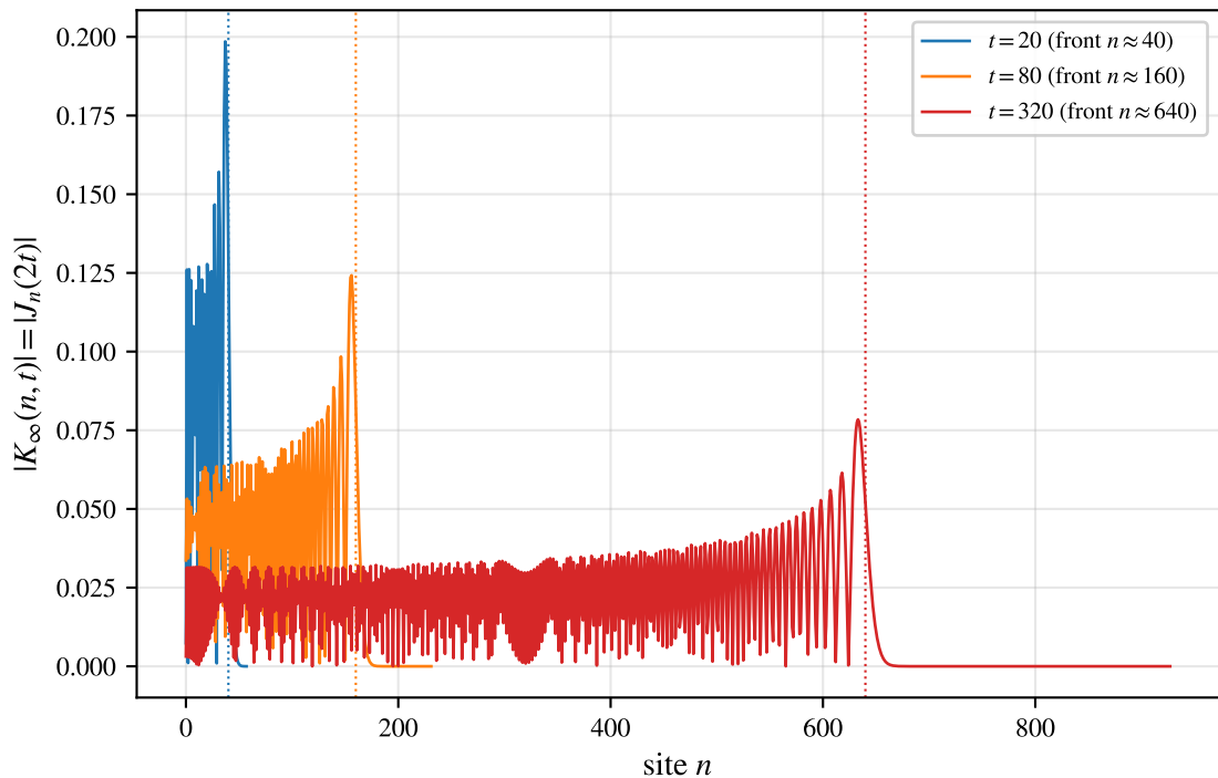
Bessel kernel |J_n(2t)| : ballistic front, (2t)^{-1/3} decay
