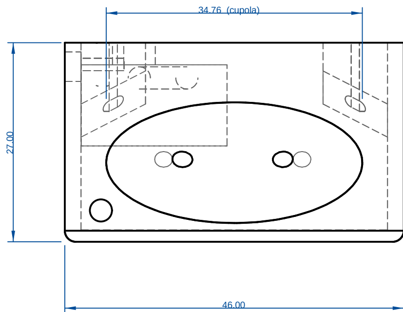
VISTA LATERALE DESTRA
