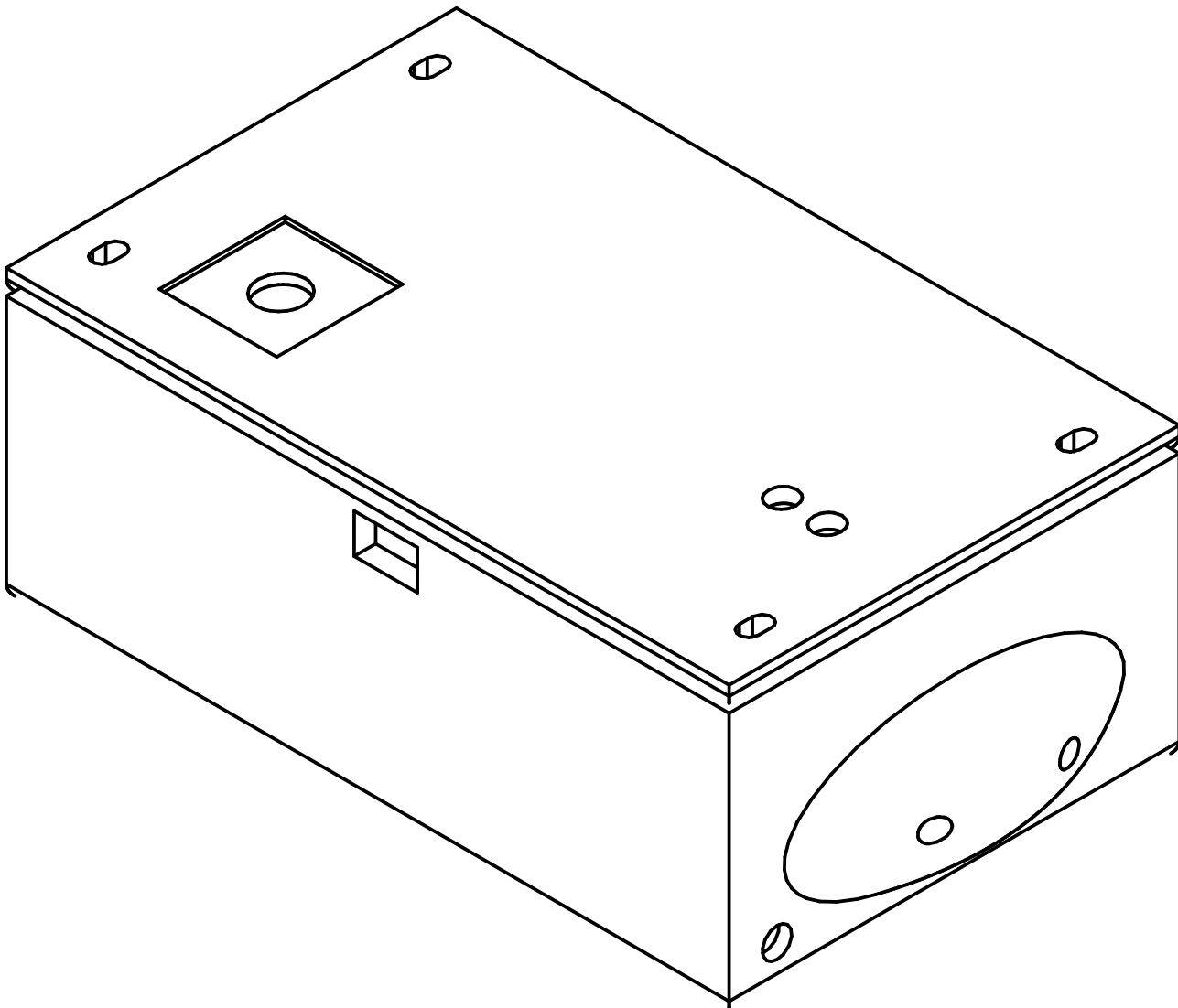
ASSIEME scatola + coperchio 2:1
