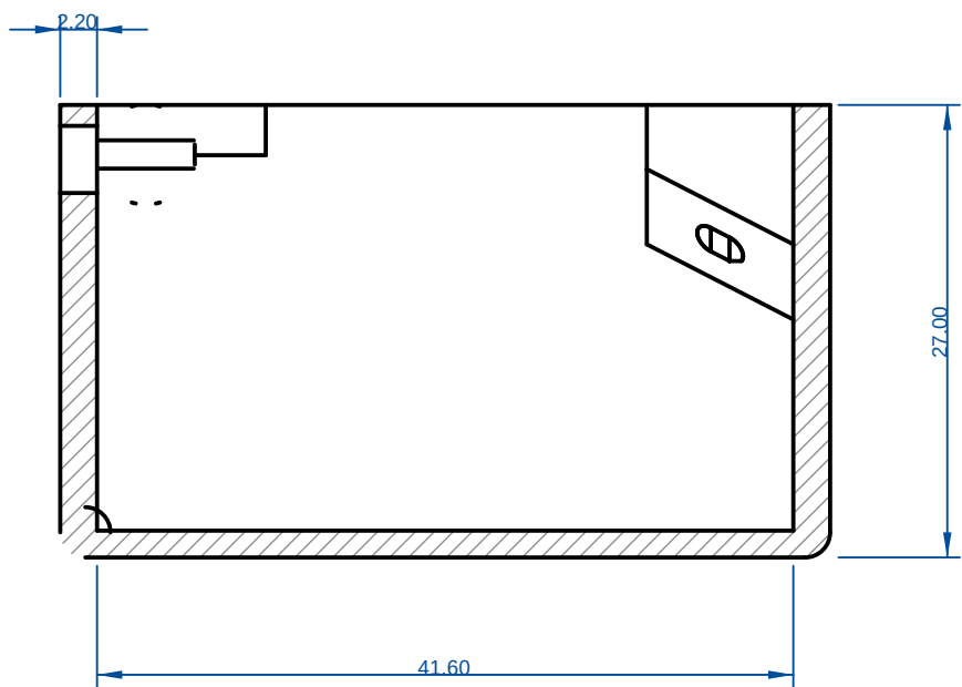
SEZIONE B-B
