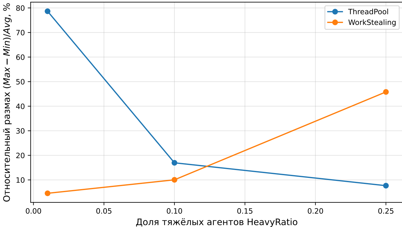
Тяжёлая нагрузка: стабильность времени кадра N=200 000
