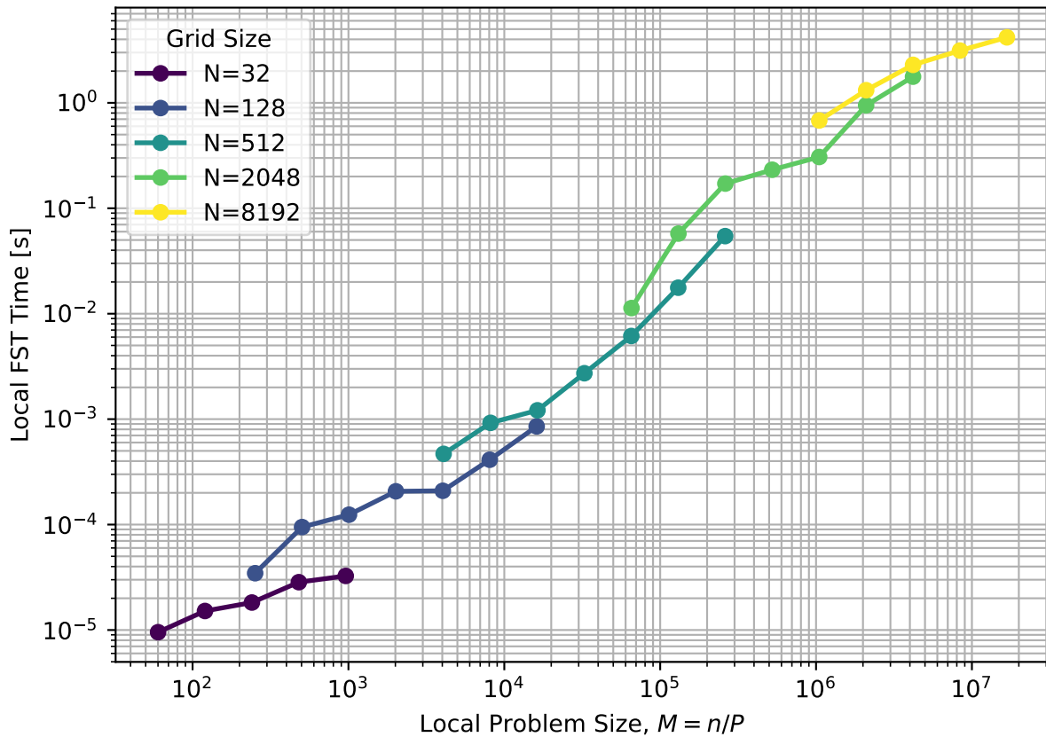
Local FST Time vs Local Problem Size
