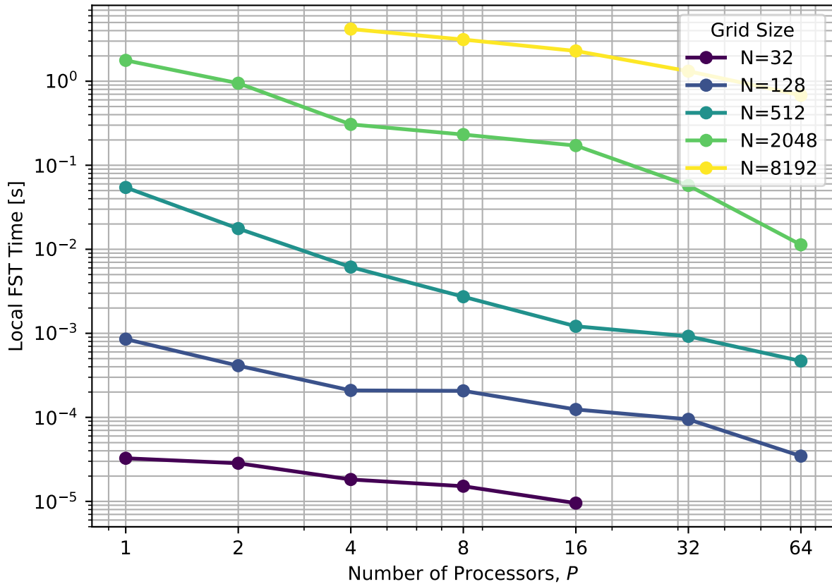
Local FST Time vs Processor Count
