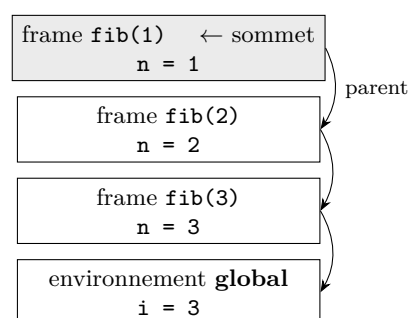
FIGURE 3.6 – Pile d’environnements pendant l’évaluation de fib(3) . Le lien parent sert à restaurer le frame courant en sortie de fonction; la résolution des variables, elle, est lexicale (frame courant puis global).
