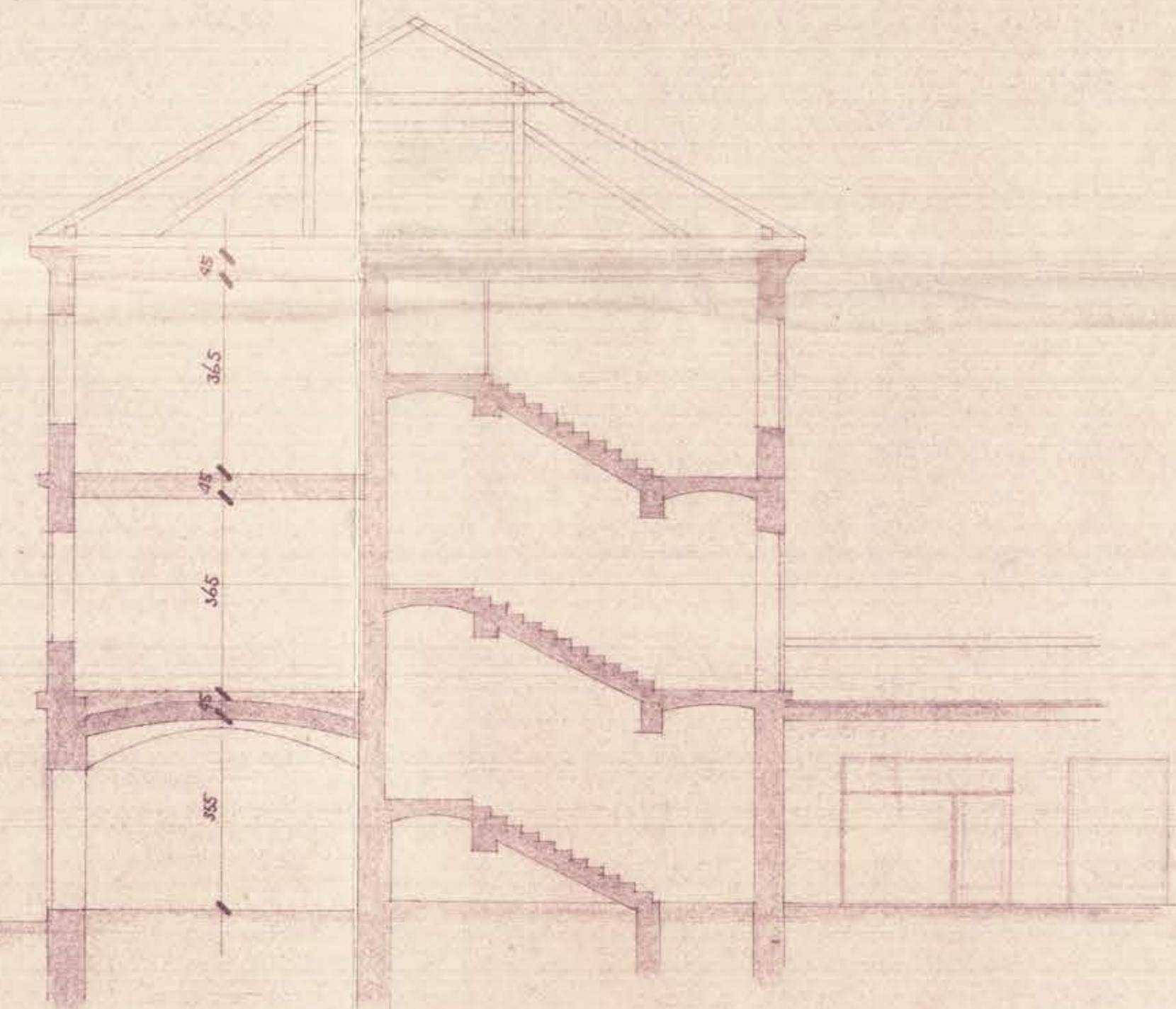
PRESJEK 1-1
