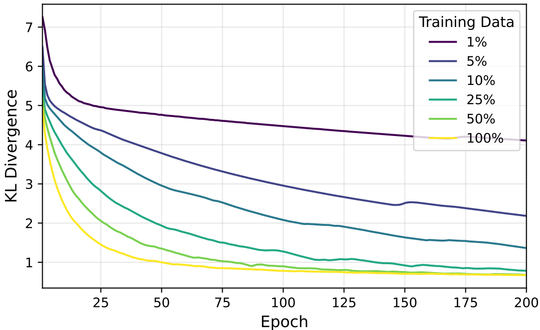
Posterior Collapse Monitoring (KL Term)
