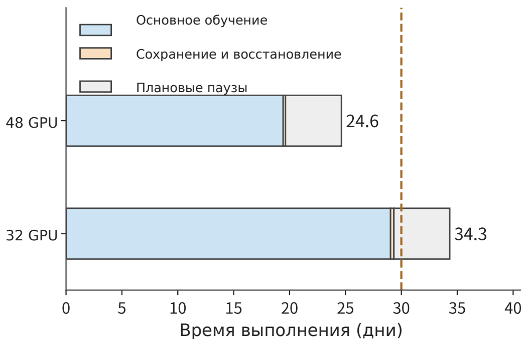
Рис. 10-45. Каждая горизонтальная полоса последовательно суммирует базовое время обучения, дополнительное время на сохранение и восстановление после сбоев, а также зарезервированные 5 дней плановых остановок. Базовое время обучения уже включает ожидание коммуникации и входных данных; небольшой оранжевый участок показывает дополнительные затраты времени, полученные из модели checkpoint. Обе конфигурации используют одну задачу и одинаковый глобальный батч, пунктирная линия обозначает срок в 30 дней.
