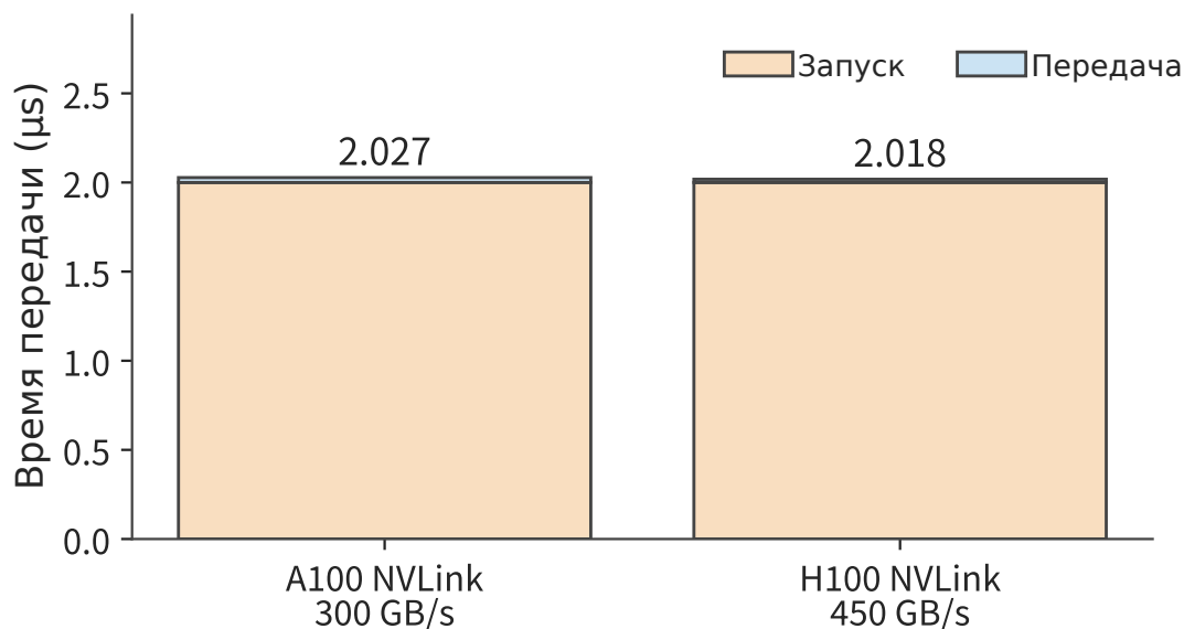
Рисунок 4-27. Время запуска и передачи 8 KiB данных. При фиксированных накладных расходах на запуск 2 μs замена NVLink A100 с пропускной способностью 300 GB/s в каждом направлении на NVLink H100 с 450 GB/s сокращает лишь тонкую синюю составляющую передачи.
