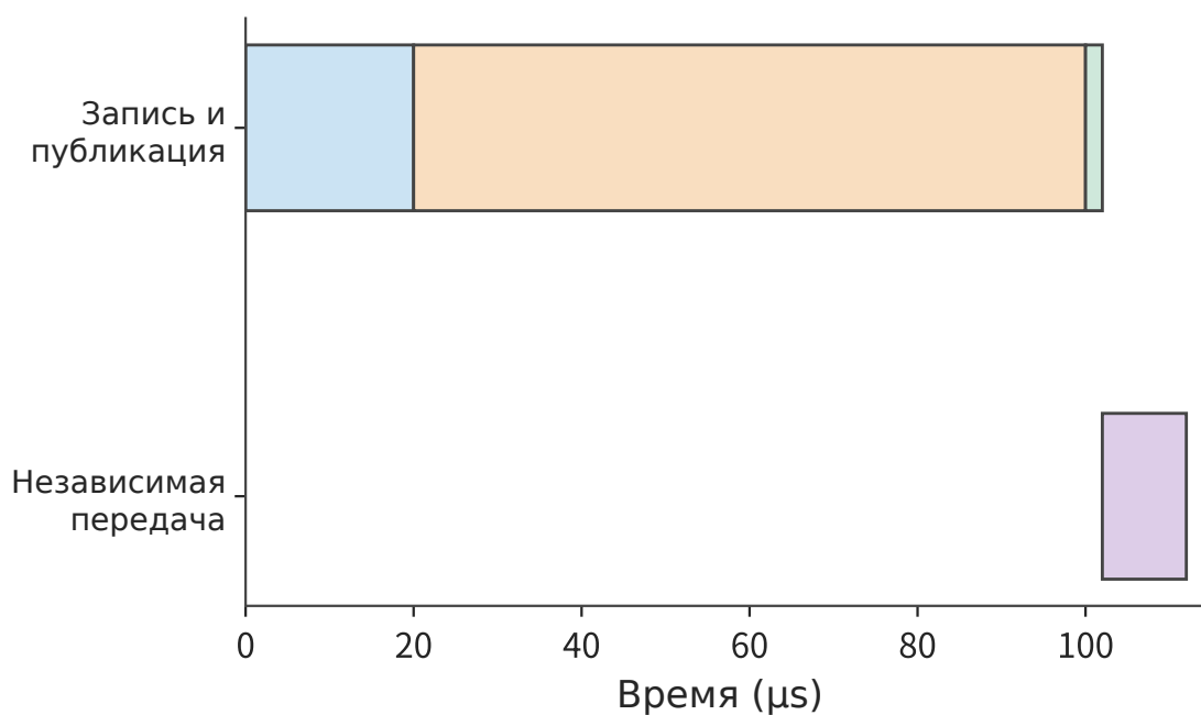
Рисунок 7-35. Независимая передача также поставлена после публикации: сначала запись 20 \mu s , затем восстановление и обеспечение видимости данных 80 \mu s , уведомление 2 \mu s и, наконец, независимая передача 10 \mu s .
