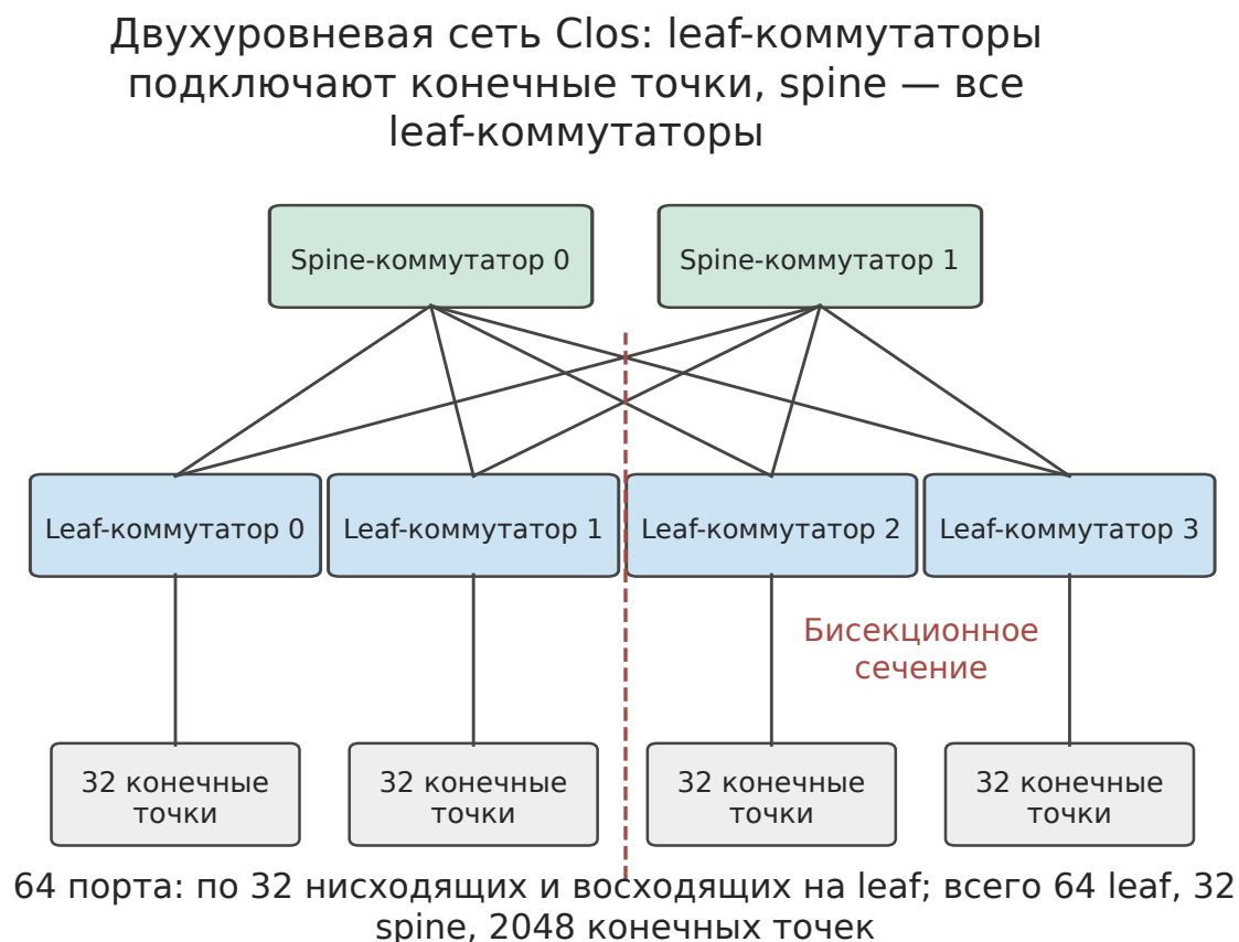
Рис. 7-3. Двухуровневая сеть Clos. Половина портов каждого leaf-коммутатора подключена к серверам, а другая половина — к spine-коммутаторам; любые два leaf-коммутатора могут обмениваться данными через любой spine-коммутатор. Пунктирная линия делит конечные узлы на две половины, а пересекающие её соединения между leaf- и spine-коммутаторами образуют бисекционный разрез. На рисунке для наглядности показаны четыре leaf-коммутатора и два spine-коммутатора; при 64 портах фактически используются 64 leaf-коммутатора и 32 spine-коммутатора.
