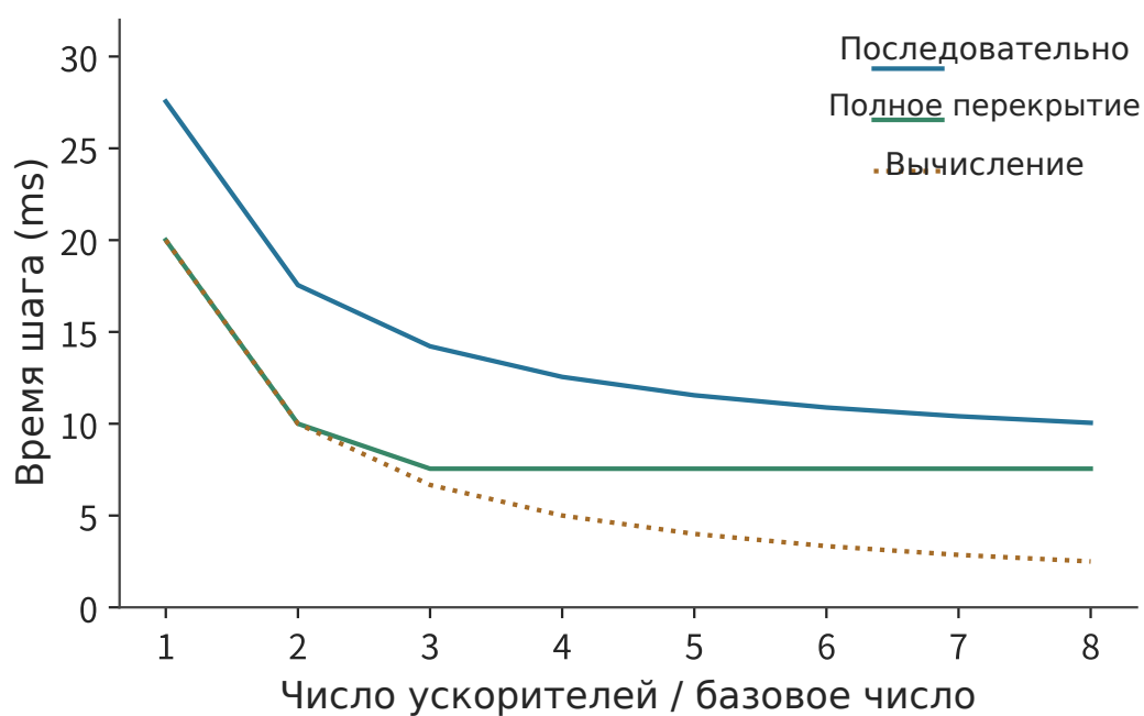
Рис. 7-2. Эффект увеличения числа карт при фиксированном объеме межсерверной передачи. В каждом направлении через одну сетевую карту с пропускной способностью 50 GB/s передаётся 360 MiB; исходное время вычислений составляет 20 ms и сокращается обратно пропорционально увеличению числа карт. Кривые рассчитаны для последовательного выполнения вычислений и коммуникации и для их полного перекрытия; коммуникационная составляющая равна времени передачи через разрез.
