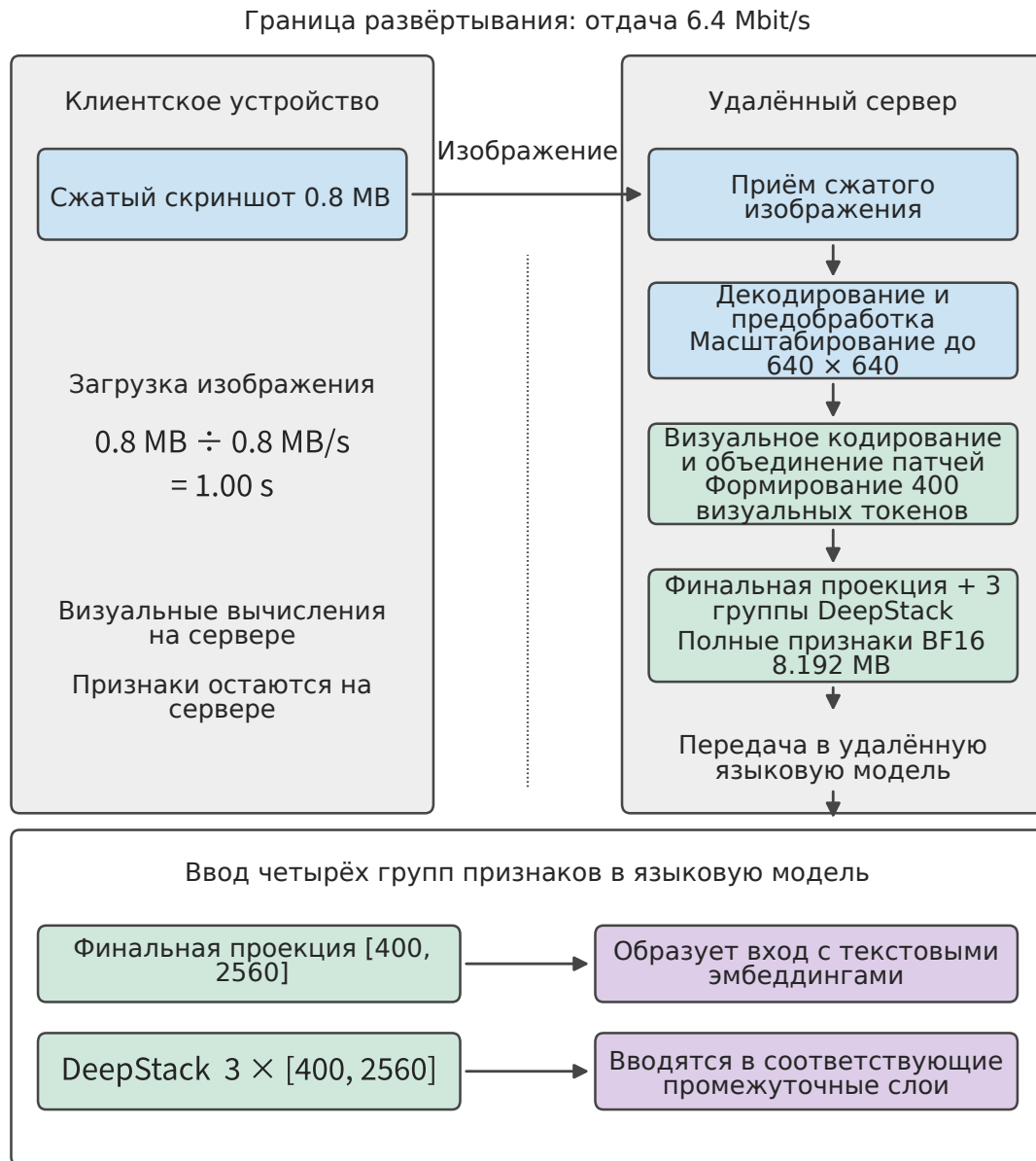
Рис. 12-10. Путь выполнения при удалённом кодировании. Конечное устройство загружает сжатый снимок экрана размером 0,8 MB, после чего удалённая сторона последовательно выполняет декодирование и предварительную обработку, визуальное кодирование и подключение признаков; итоговая проекция и три группы признаков DeepStack остаются внутри сервера. При исходящей скорости 6,4 Mbit/s передача изображения занимает 1 секунду; время кодирования и ожидания в очереди учитывается отдельно.
