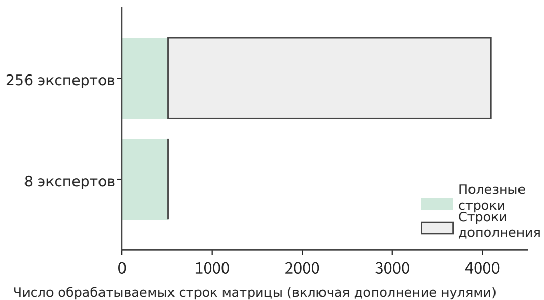
Рисунок 4-10. Объём вычислений для одинаковых 512 полезных входных строк у всех экспертов. После распределения между 256 экспертами в общей сложности обрабатываются 4096 строк, а при концентрации у восьми экспертов — только 512 строк.
