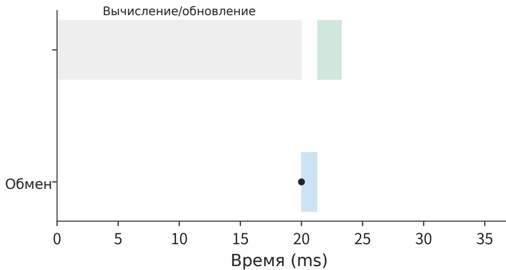
Рисунок 7-55. Здесь используется иерархическая редукция, но вычисление, обмен и обновление по-прежнему выполняются последовательно. Обмен сокращается приблизительно до 1.3 ms, а весь шаг занимает около 23.3 ms. Серым показано вычисление, синим — обмен, зелёным — обновление; точка обозначает готовность данных для обмена.
