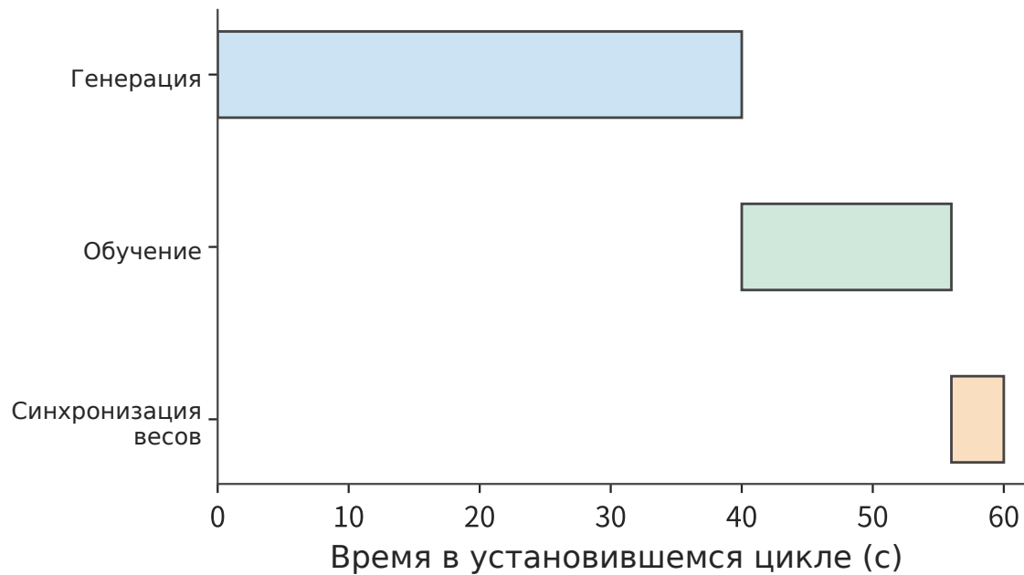
Рис. 10-42. Синхронный цикл последовательно генерирует текущую порцию образцов, обучается на ней и синхронизирует веса, затрачивая соответственно 40, 16 и 4 s, всего 60 s.
