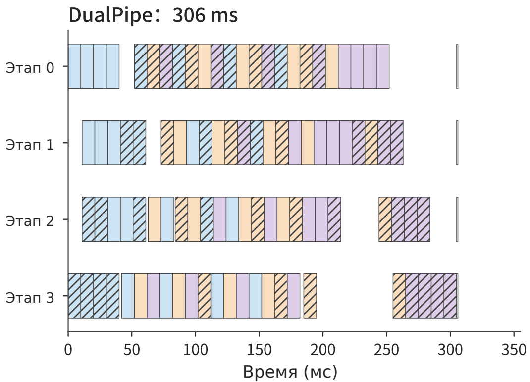
Рис. 10-23. Временная шкала этапов DualPipe, время завершения — 306 ms. Цвета соответствуют рис. 10-22, а заштрихованные блоки обозначают вычисления второй половины micro-batch, поступающей с этапа 3 в обратном направлении. Каждый этап одновременно обслуживает два направления; промежутки прогрева и опустошения одного направления заполняются блоками другого. Цена — хранение двух копий параметров на каждой карте.
