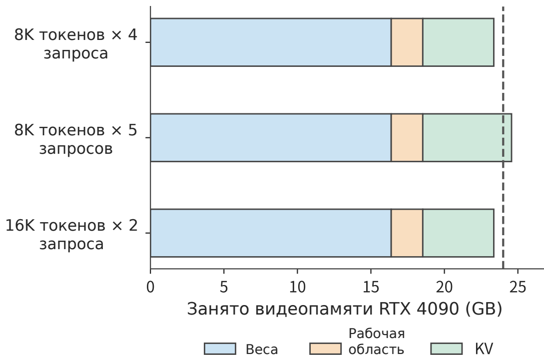
Рисунок 4-13. Веса, рабочая область и KV-кэш в 24 GB видеопамяти RTX 4090. Четыре запроса с контекстом 8K и два запроса с контекстом 16K помещаются, а пять запросов с контекстом 8K превышают обозначенный пунктиром предел ёмкости.
