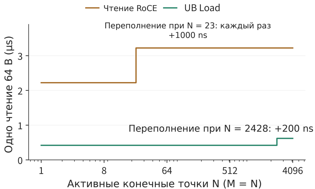
Рисунок 7-34. Зависимость задержки одного чтения 64 В от количества активных конечных точек при внутрикристалльном кэше объёмом 256 KiB. Для попарных соединений задержка возрастает на 1000 ns при 23 конечных точках, а для конечных точек и каналов — на 200 ns при 2428 конечных точках. Ось абсцисс имеет логарифмический масштаб.
