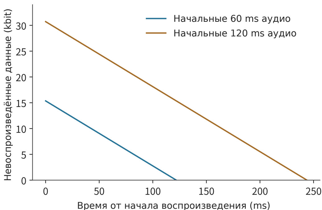
Рис. 12-7. Объем буфера равен начальному объему данных плюс совокупный объем принятых данных минус совокупный объем воспроизведенных данных. Для воспроизведения РСМ требуется 256 kbit/s, а скорость приёма составляет лишь 130 kbit/s, поэтому скорость уменьшения на обеих прямых равна 126 kbit/s. Начальные буферы содержат соответственно 60 ms и 120 ms аудио и исчерпываются примерно через 0,12 и 0,24 секунды; каждая линия показана до момента первого исчерпания.
