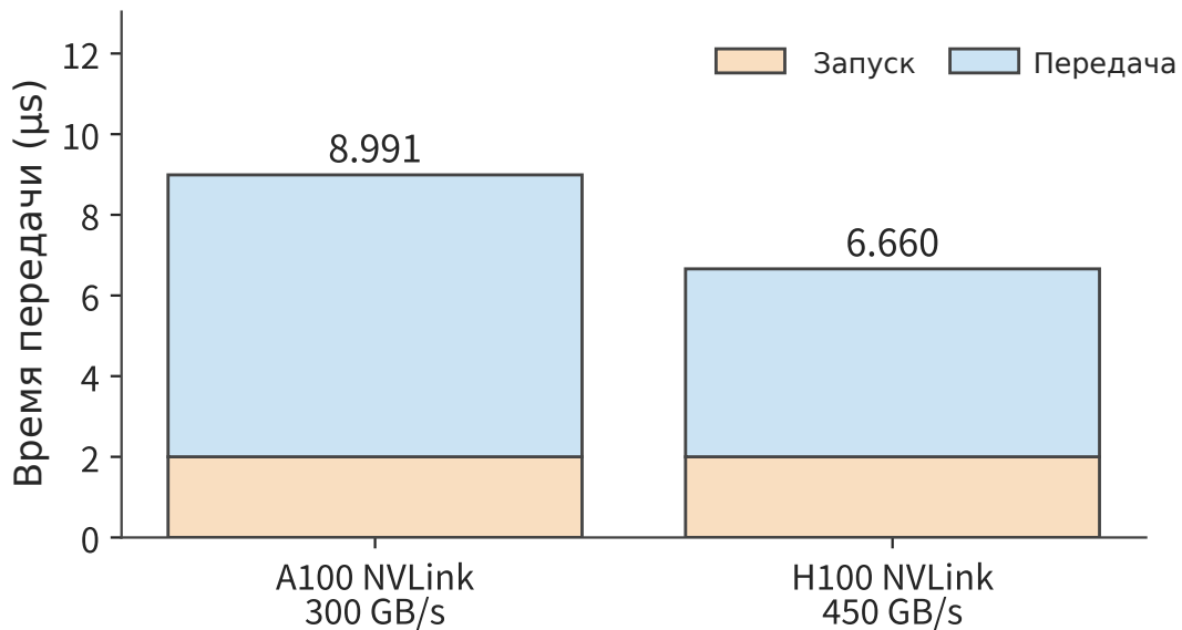
Рисунок 4-28. Время передачи 2 MiB данных при тех же условиях запуска. Синяя составляющая передачи занимает основную часть времени, поэтому переход на NVLink H100 даёт более заметный выигрыш; диапазон вертикальной оси на этом и предыдущем рисунках указан отдельно.
