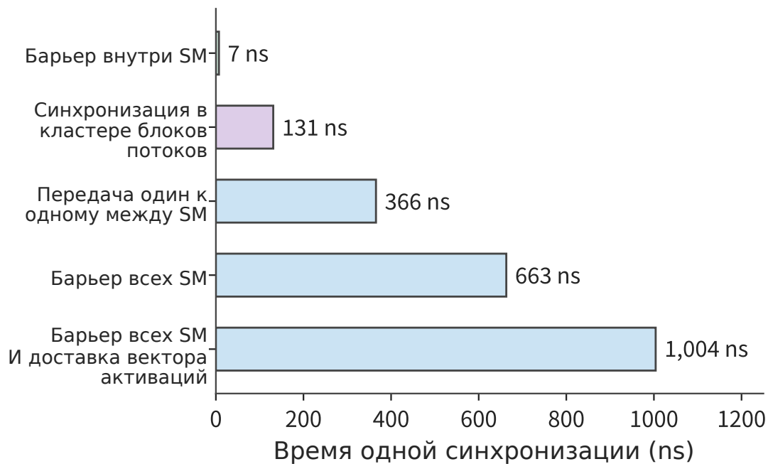
Рисунок 4-25. Время одной синхронизации разных уровней на RTX PRO 6000. Зелёный, фиолетовый и синий цвета соответствуют синхронизации внутри SM, внутри кластера блоков потоков и через L2; передача «один к одному» реализована с семантикой release-acquire, а при сведении всех SM доставляется вектор объёмом 8 KiB, размноженный в восьми экземплярах. Значения представляют собой минимумы из нескольких измерений во время совместного использования GPU.
