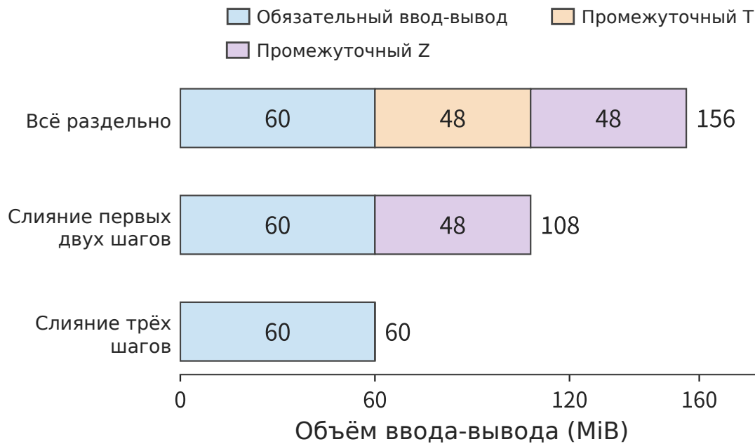
Рисунок 5-15: устранение сохранения каждого промежуточного результата размером 24 MiB включает одну запись и одно чтение, то есть в сумме 48 MiB. G и U представлены в BF16, конечный результат занимает 1 byte на элемент, scale квантования задан заранее. Во всех вариантах используются одинаковые операции и порядок округления.
