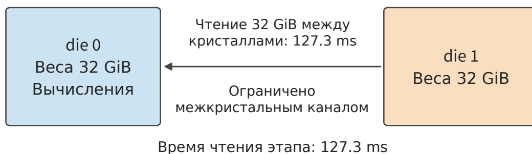
Рисунок 4-26. Когда все вычисления выполняются на кристалле 0, 32 GiB весов с кристалла 1 приходится читать через межкристальный канал. В B200 межкристальное чтение ограничено HBM кристалла 1 и занимает около 8,6 ms — столько же, сколько локальное чтение; в Ascend 910C оно ограничено межкристальным каналом и занимает около 127 ms.
