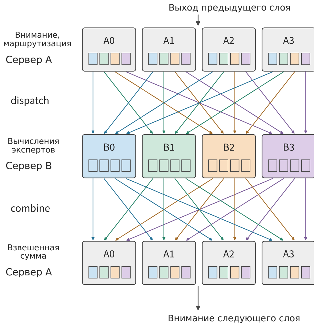
Рис. 9-16. Порядок выполнения одного слоя МоЕ между двумя серверами; время направлено сверху вниз. А0–А3 выполняют механизм внимания и маршрутизацию, В0–В3 — экспертов. Маленький прямоугольник обозначает группу входных данных, которую одна карта А отправляет одной карте В; цвет показывает целевую карту В. Dispatch доставляет прямоугольники картам В соответствующего цвета, а combine возвращает результаты исходным картам А. Оба обмена представляют собой All-to-All размером 4×4.
