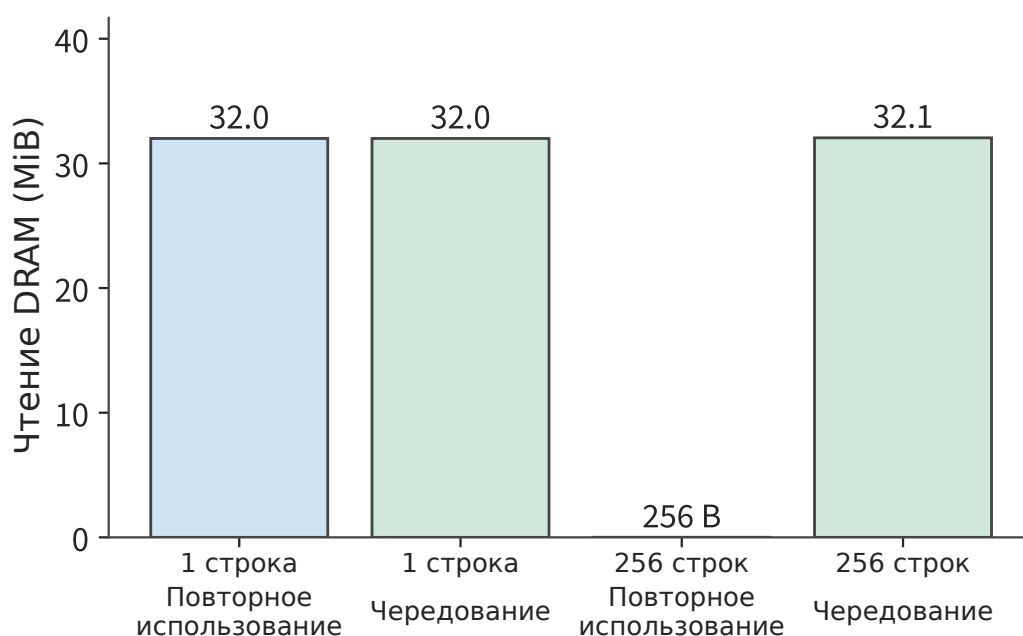
Рисунок 4-42. Отдельно собранные счётчики чтения DRAM для тех же четырёх условий. Для одной строки во всех случаях считывается около 32 MiB; для 256 строк при повторном использовании — 256 bytes, при чередовании — около 32,1 MiB. Счётчики доступа и обычные измерения времени собирались раздельно. «Повторное использование» и «чередование» означают соответственно сохранение и смену адреса весов.
