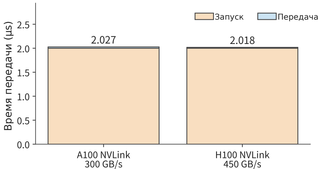
Рисунок 4-28. Время запуска и передачи 8 KiB данных. При фиксированных накладных расходах на запуск 2 μs замена NVLink A100 с пропускной способностью 300 GB/s в каждом направлении на NVLink H100 с 450 GB/s сокращает лишь тонкую синюю составляющую передачи.
