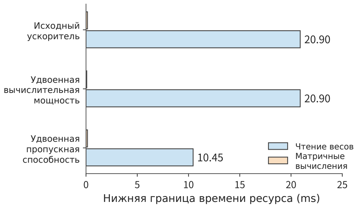
Рис. 1-9. При неизменных объёмах вычислений и чтения по отдельности удваиваются вычислительная мощность и пропускная способность. Синяя полоса показывает нижнюю границу чтения весов, оранжевая — нижнюю границу матричных вычислений; более продолжительное чтение определяет направление оптимизации при этих условиях. Каждый столбец показывает нижнюю границу времени вычислений или чтения данных, однако полное выполнение всё равно должно учитывать зависимости.
