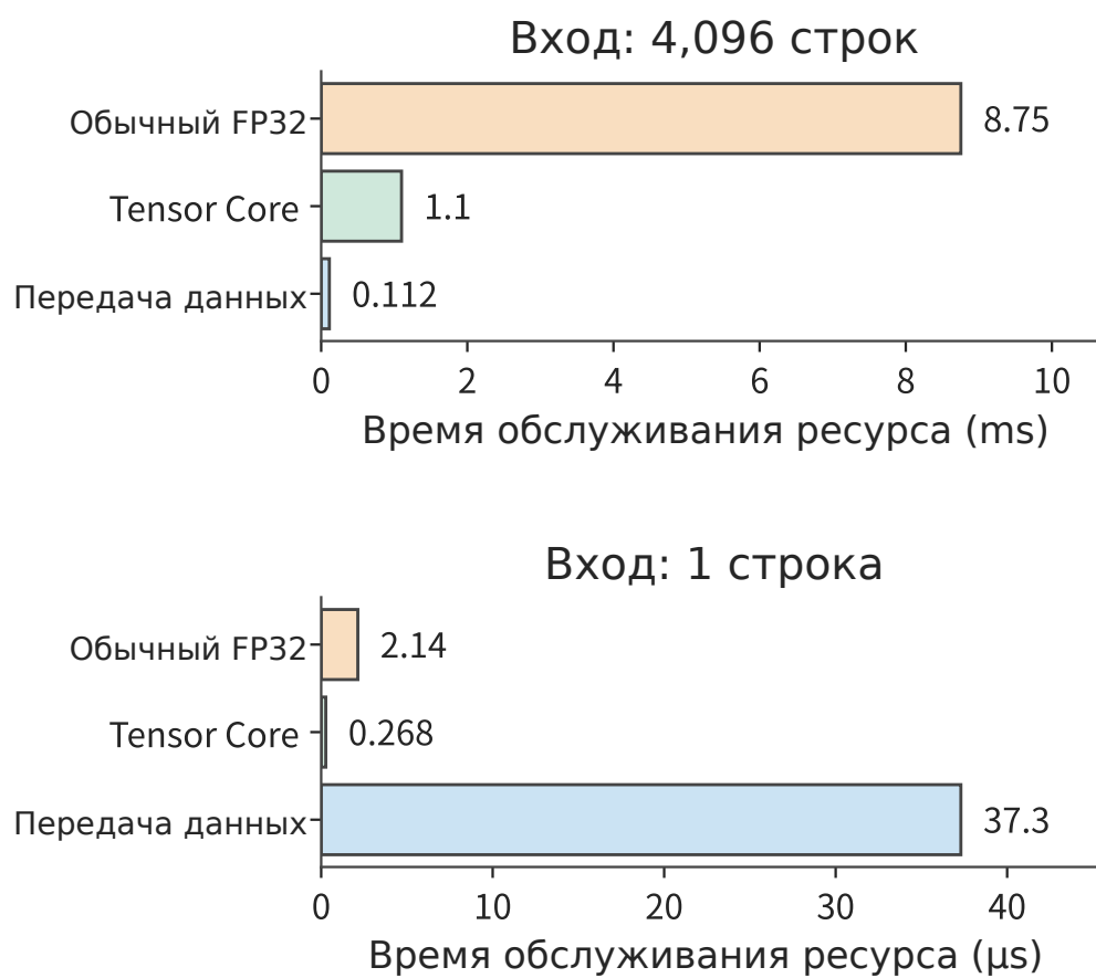
Рис. 4-30. Проекция Q на одном V100. При 4 096 строках Tensor Core значительно сокращает время матричных вычислений; при одной строке оба вычислительных тракта работают быстрее, чем выполняется передача весов. Для верхней и нижней групп отдельно указаны единицы времени.
