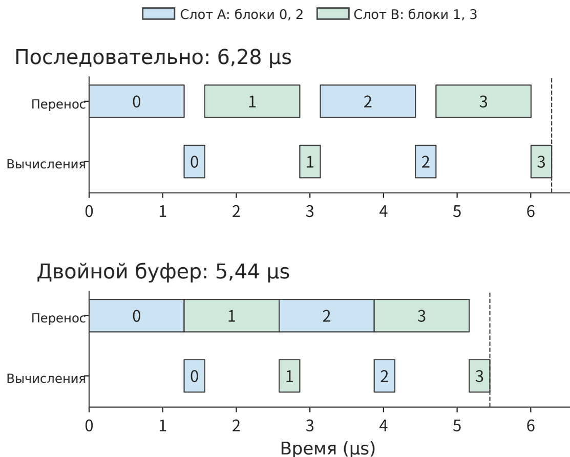
Рисунок 5-17: поочерёдное повторное использование двух входных слотов позволяет перекрыть перемещение и вычисления. На одном SM H100 перемещение каждого блока занимает 1,29 \mu s, а вычисление — 0,28 \mu s; ресурсы независимы, накладные расходы синхронизации не учитываются; одинаковый цвет обозначает один и тот же слот. Перекрытие скрывает только вычисления, а время завершения определяется непрерывной последовательностью перемещений.
