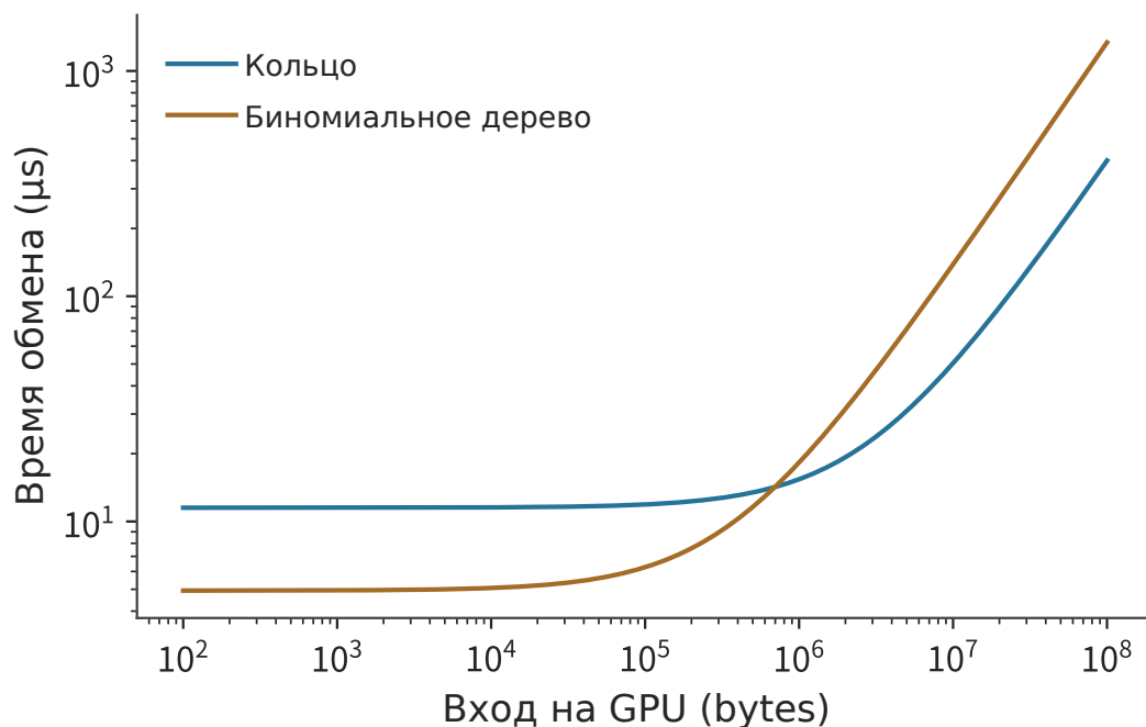
Рисунок 6-26. Модели времени для кольцевого алгоритма на восьми картах и несегментированного биномиального дерева при 0,822 \mu\text{s} на раунд и 450 GB/s в каждом направлении. Точка пересечения находится примерно на 680 KiB; вход decode размером 10 KiB расположен в области преимущественного влияния накладных расходов запуска, а вход prefill размером 80 MiB — в области преимущественного влияния времени передачи данных.
