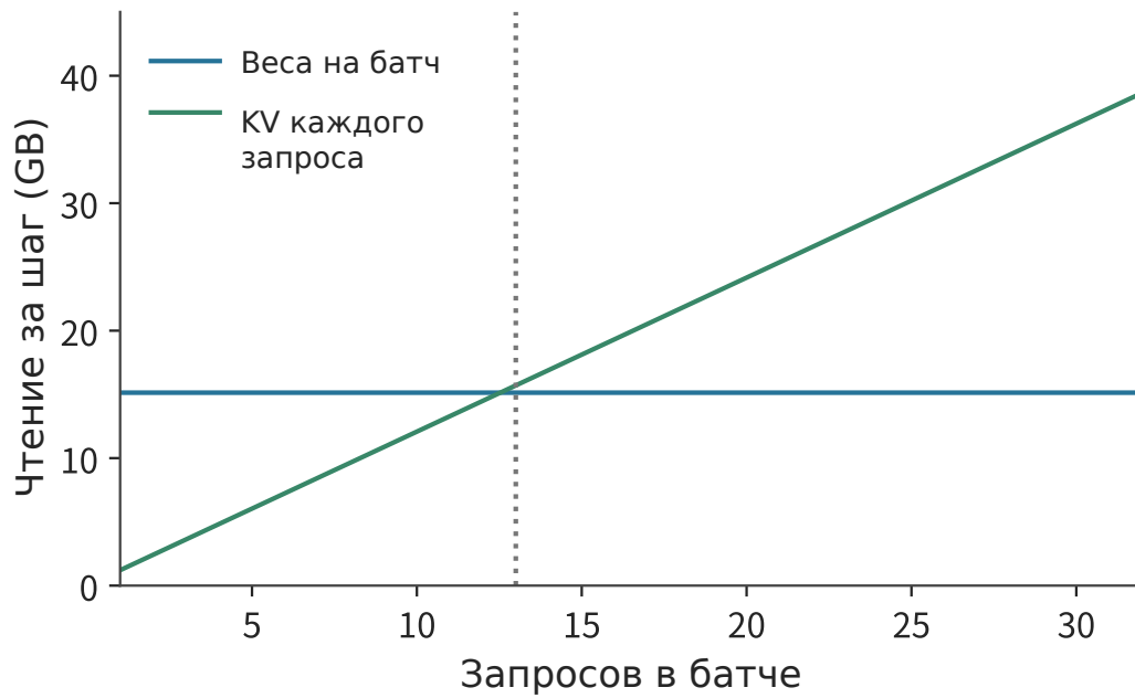
Рисунок 4-37. При фиксированных весах KV по-прежнему считывается отдельно для каждого запроса. По условию для каждого запроса сохраняется контекст 8K; начиная с размера пакета 13, объем чтения KV превышает объем чтения общих весов.
