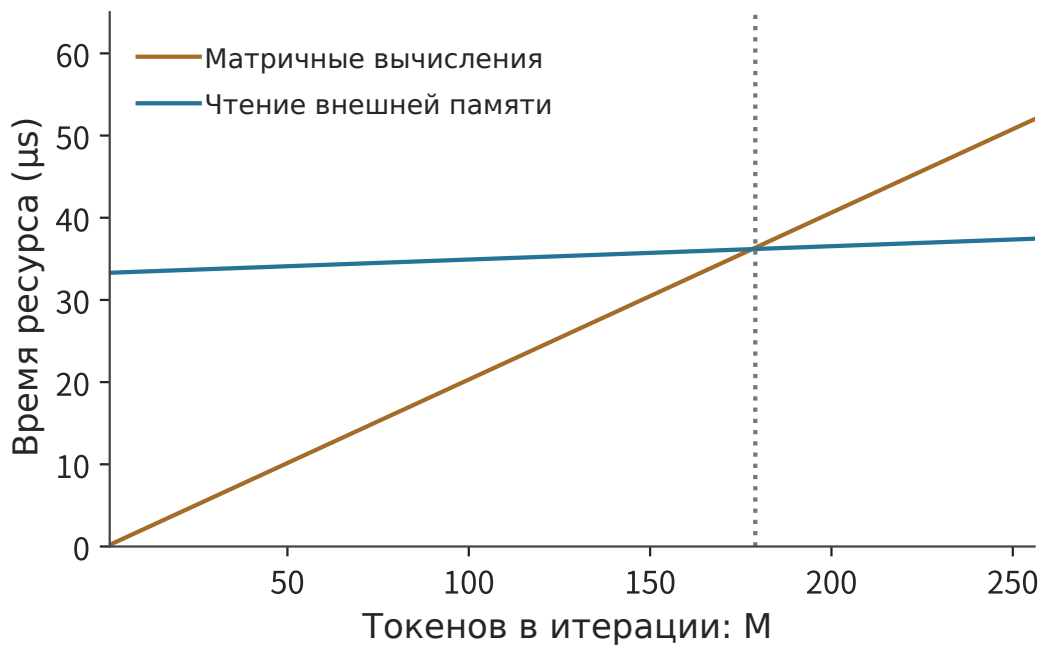
Рисунок 4-39. Изменение времени вычислений и обращений к памяти для одной и той же проекции Q при изменении числа входных строк. Объем вычислений растёт вместе с числом строк, а обращения к внешней памяти включают как фиксированный объем весов, так и растущие объёмы входных и выходных данных; начиная со 179 строк вычисления занимают больше времени.
