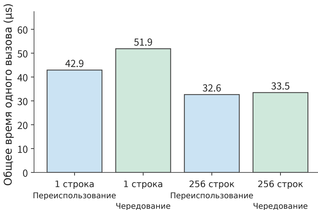
Рисунок 4-41. Полное время проекции на RTX PRO 6000. Для каждого условия выполнено одиннадцать раундов по шестнадцать вызовов; приведена медиана рассчитанного для каждого раунда среднего времени одного вызова. Измерение времени включает отправку команд и синхронизацию. «Повторное использование» означает, что несколько вызовов считывают веса по одному адресу; «чередование» означает смену адреса весов между вызовами.
