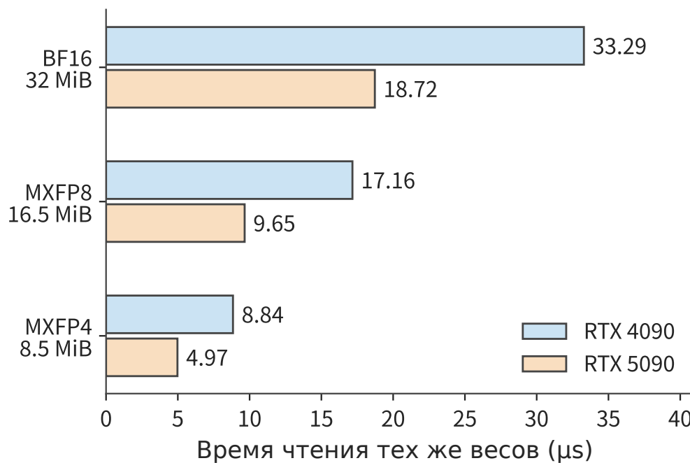
Рис. 4-31. Бюджет хранения и чтения одного и того же массива весов 4096×4096. Каждые 32 низкоточных значения используют общий однобайтовый масштабный коэффициент. При снижении разрядности с BF16 до MXFP4 общий объём весов и масштабных коэффициентов сокращается с 32 MiB до 8,5 MiB.
