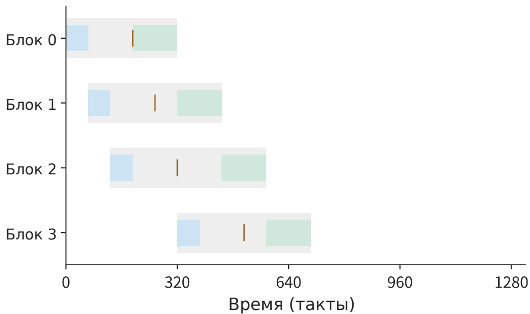
Рисунок 4-21. При трёх входных слотах первые три блока запускаются заранее, а после освобождения первого слота в него поступает четвёртый блок. Матричный блок непрерывно работает с 192 до 704 tick, поэтому четвёртый слот уже не сокращает время завершения. Один tick на горизонтальной оси соответствует одному такту SM B200; каждая строка соответствует одному блоку данных, серый цвет обозначает занятость входного слота, синий — передачу, зелёный — вычисление, а вертикальная метка — готовность данных.
