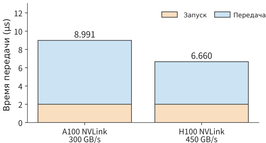
Рисунок 4-29. Время передачи 2 MiB данных при тех же условиях запуска. Синяя составляющая передачи занимает основную часть времени, поэтому переход на NVLink H100 даёт более заметный выигрыш; диапазон вертикальной оси на этом и предыдущем рисунках указан отдельно.
