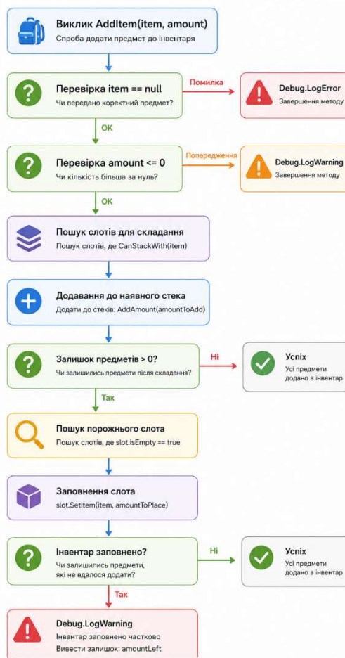
Рисунок 8 – Блок-схема алгоритму додавання предметів до інвентаря
