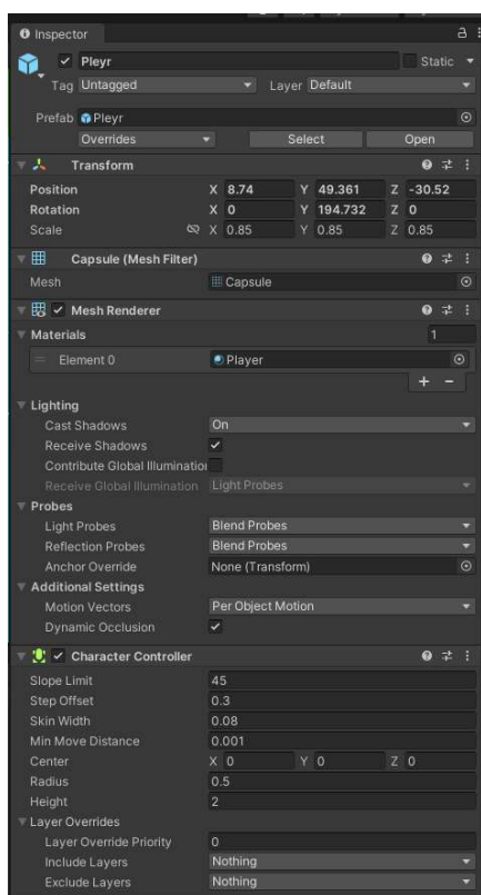
Рисунок 12 та 13 – Налаштування компонента PlayerControl в Inspector
