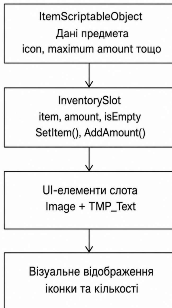
Рисунок 7 – Потік даних від ItemScriptableObject до візуального представлення слота
